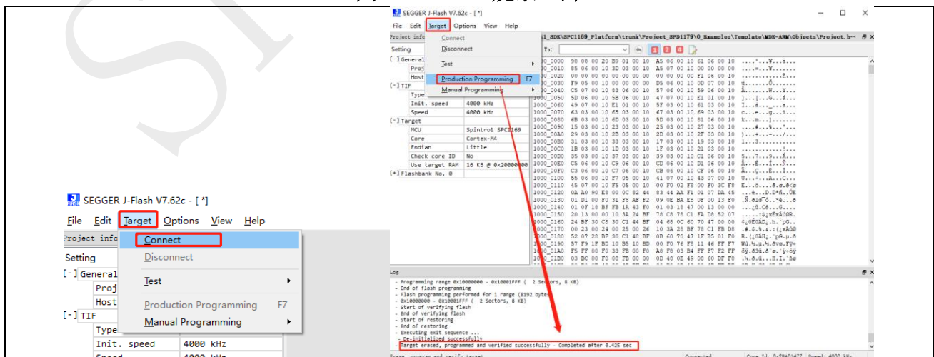
图 2-3: 烧录芯片
