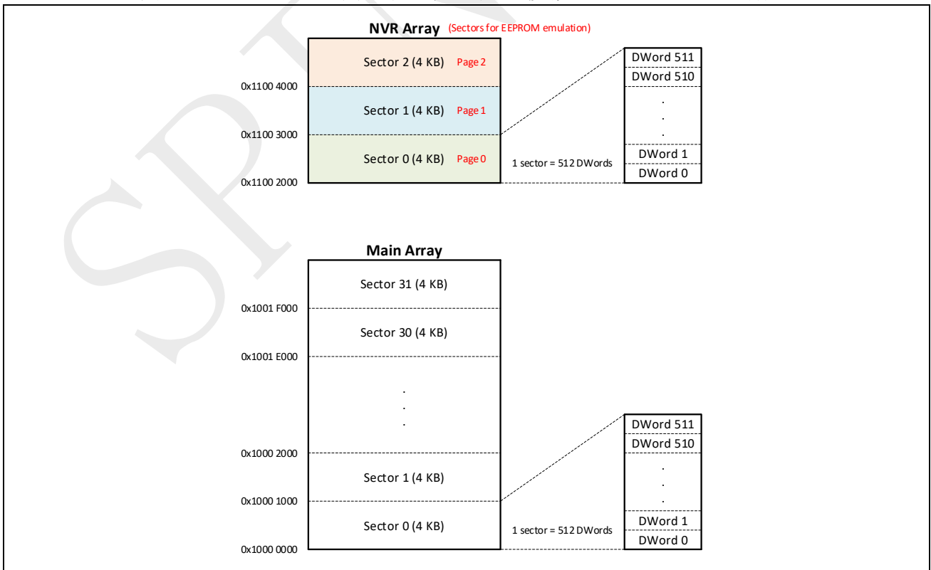
图 2-1: 以 SPC1169 为平台的产品用于模拟 EEPROM 的 Flash 扇区
