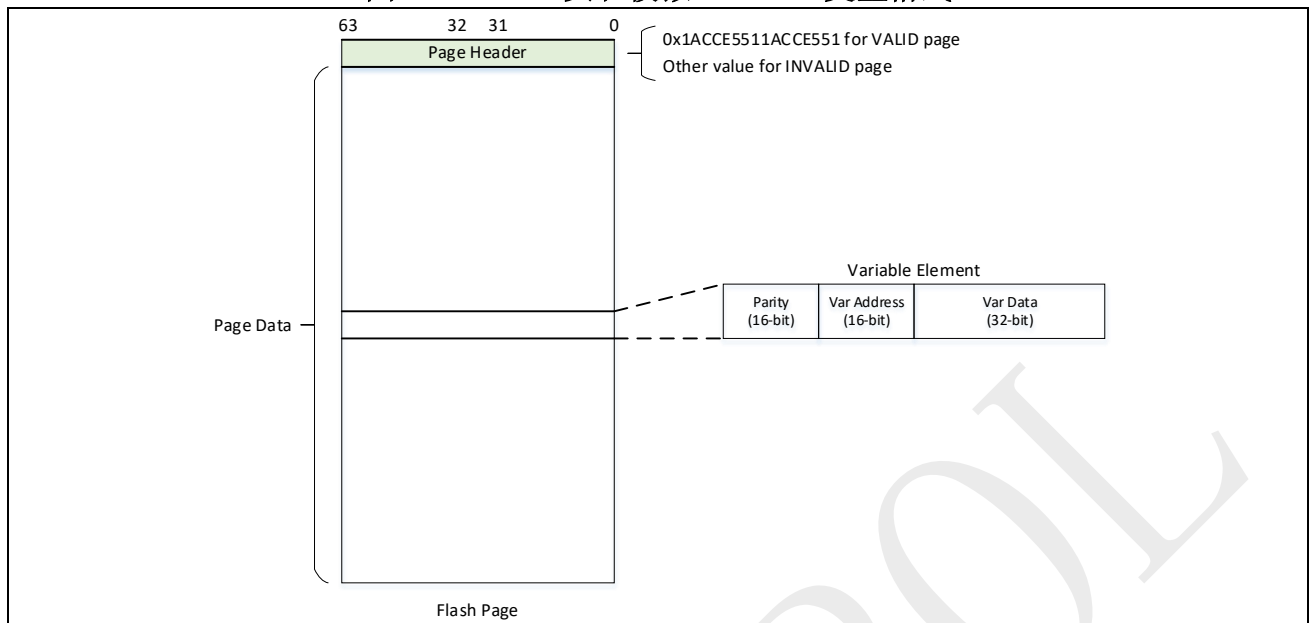
图 2-2: Flash 页和模拟 EEPROM 变量格式
