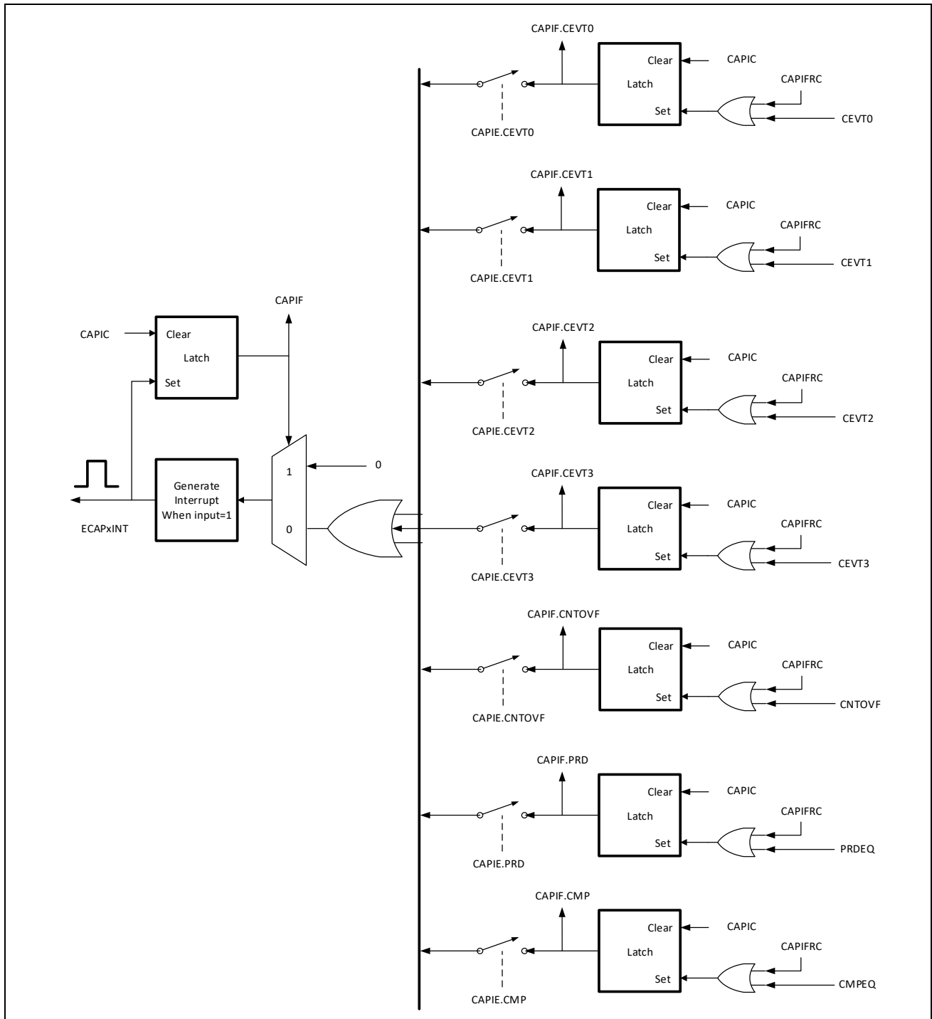
图 11-8: ECAP 模块的中断
