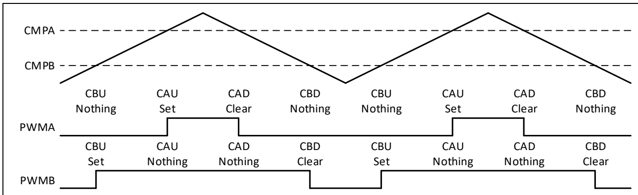
图 10-9: 上下计数时的 PWM 双边沿对称波形
