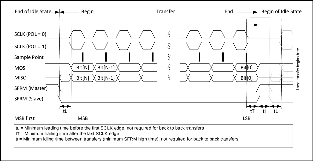
图 19-5: SSP 时钟格式 1 (PHS = 1)
