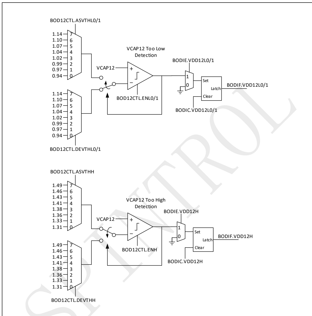
图 2-3: 1.2V 额定电压域检测电路框图
