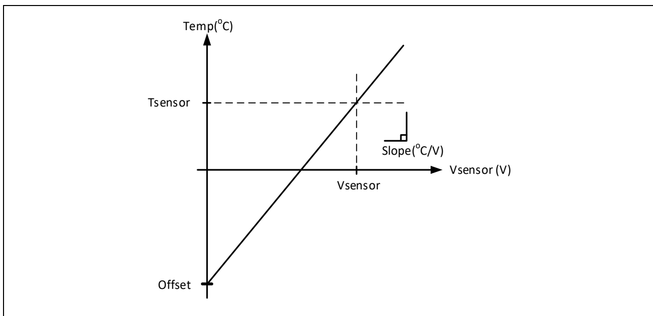
图 13-1：温度传感器转换曲线
