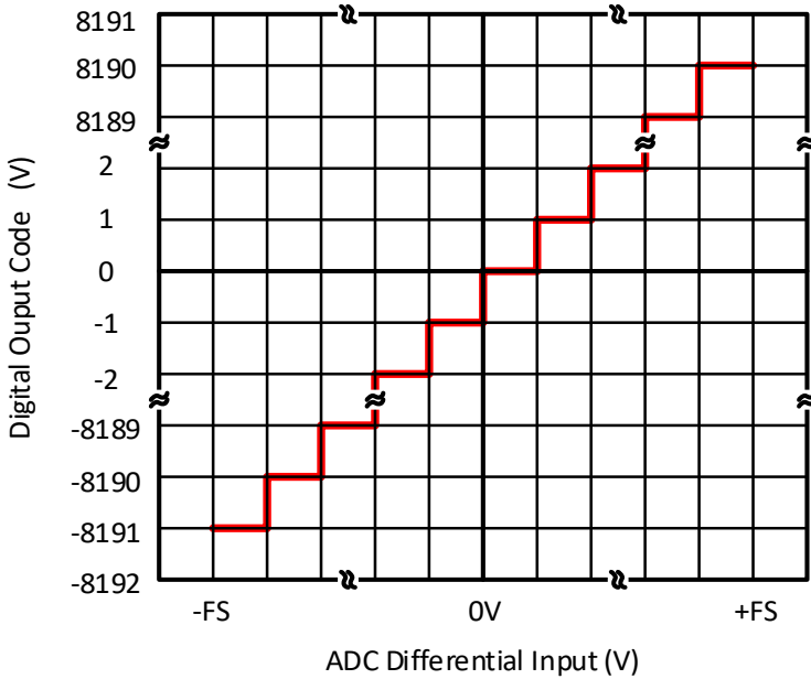
图 12-15: ADC 转换曲线
