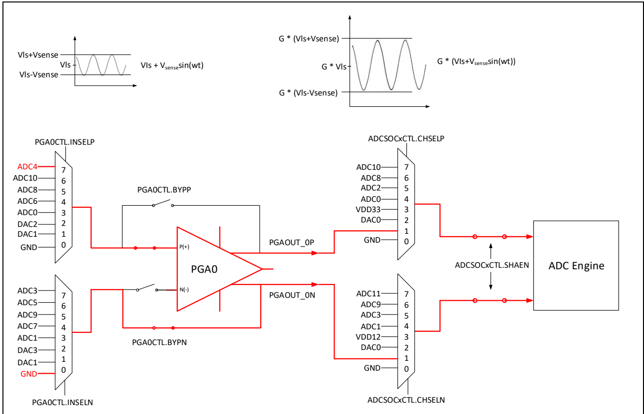
图 14-4: PGA0 选择 ADC4 作为输入（单端模式）
