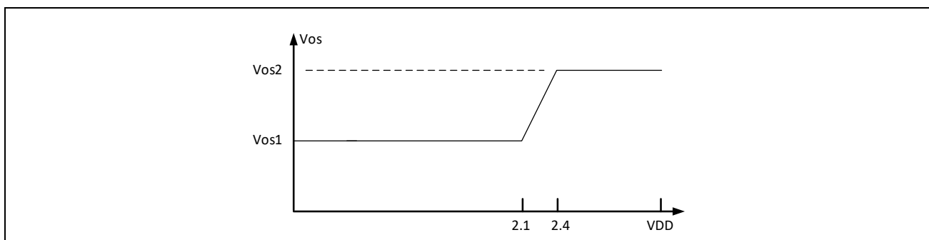
图 14-8: 偏移量随输入共模电压的变化
