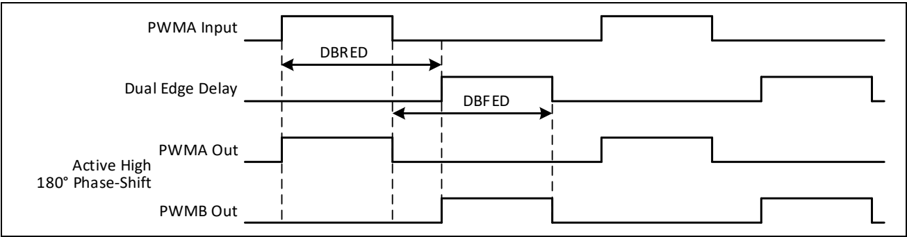
图 10-13: 双边沿延迟死区控制波形
