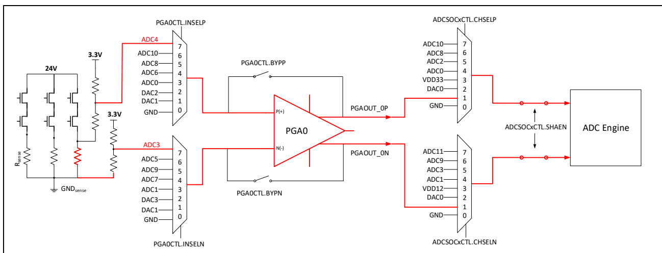
图 14-5: 电机采样示意图
