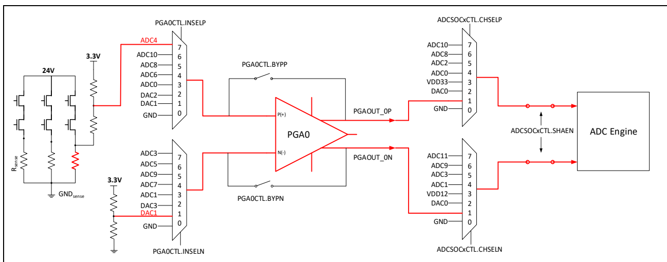
图 14-6: 电机采样示意图 (使用内部 DAC)
