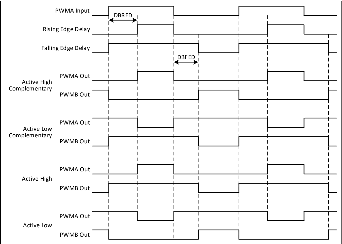
图 10-12: 死区控制典型波形
