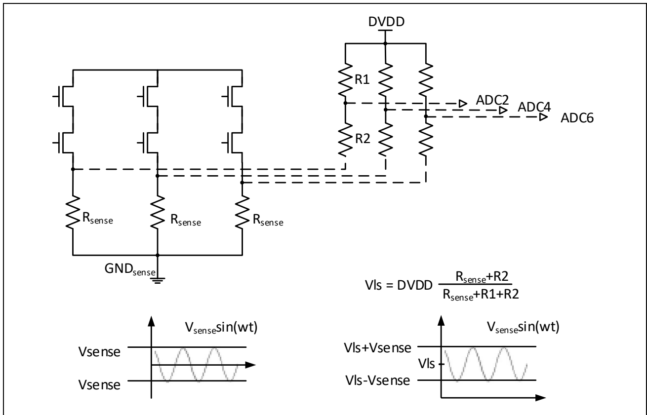
图 14-3：单端模式下采样电流示意图
