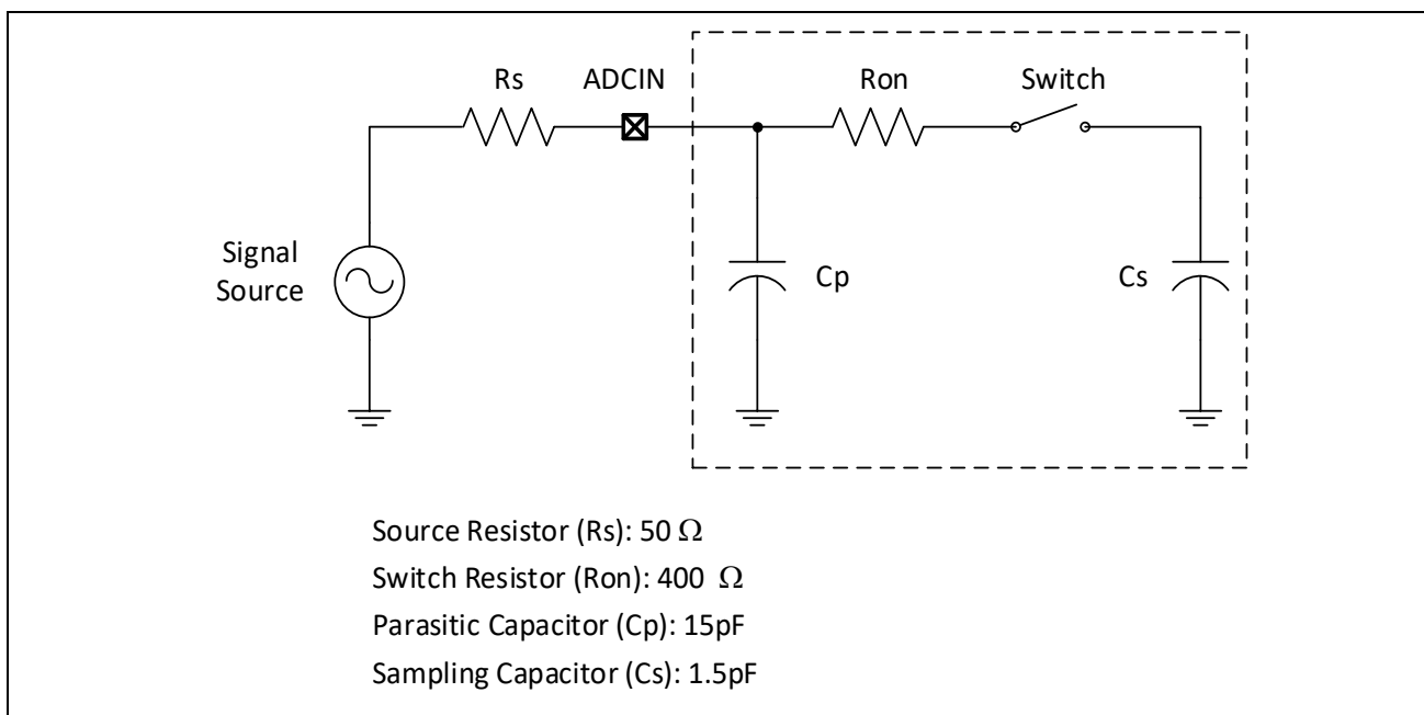
图 12-6: ADCx 输入通路 RC 网络
