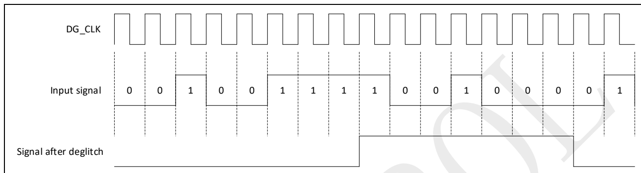
图 4-4：输入消抖
