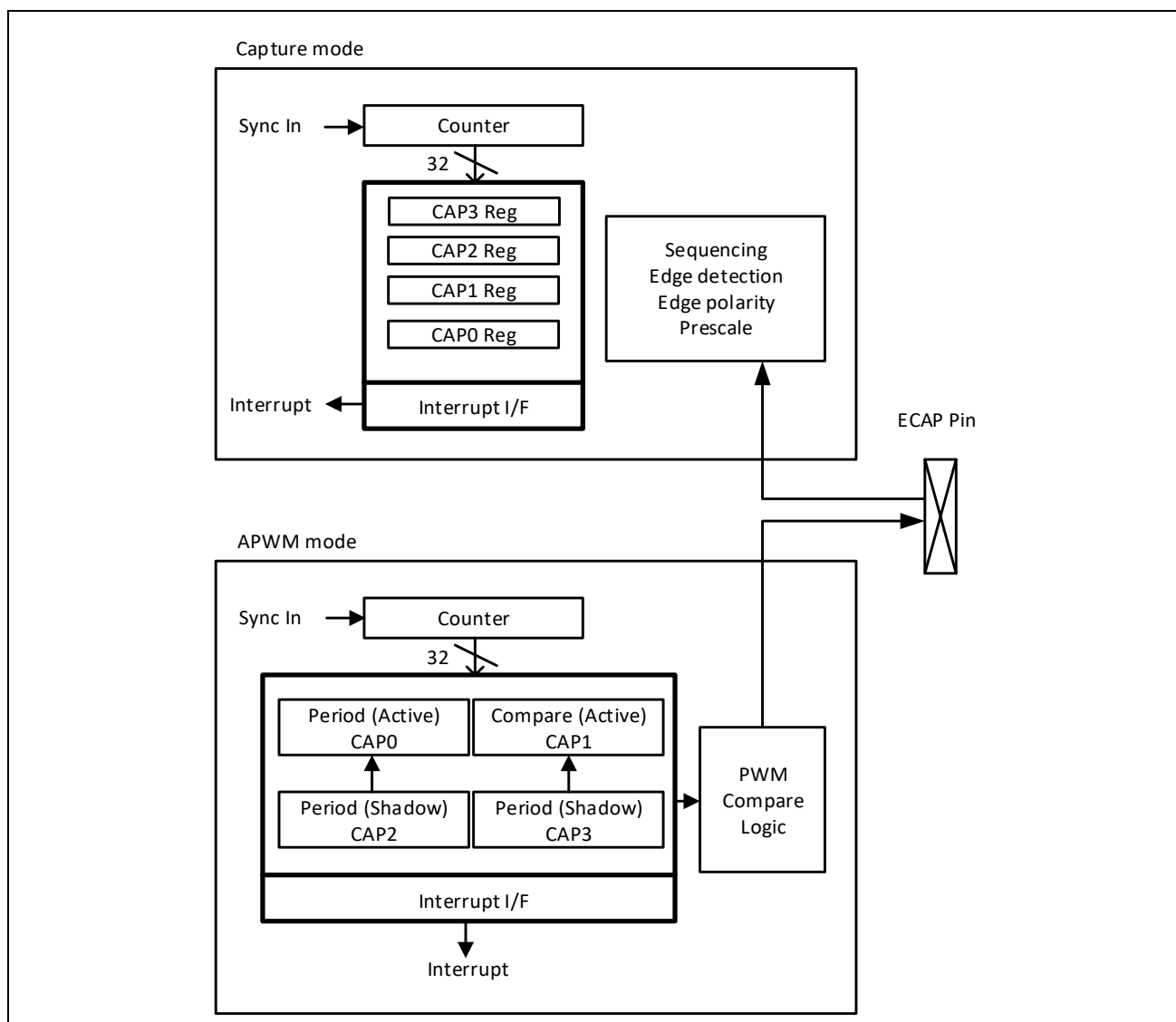
图 11-2: 捕获模式和 APWM 模式
