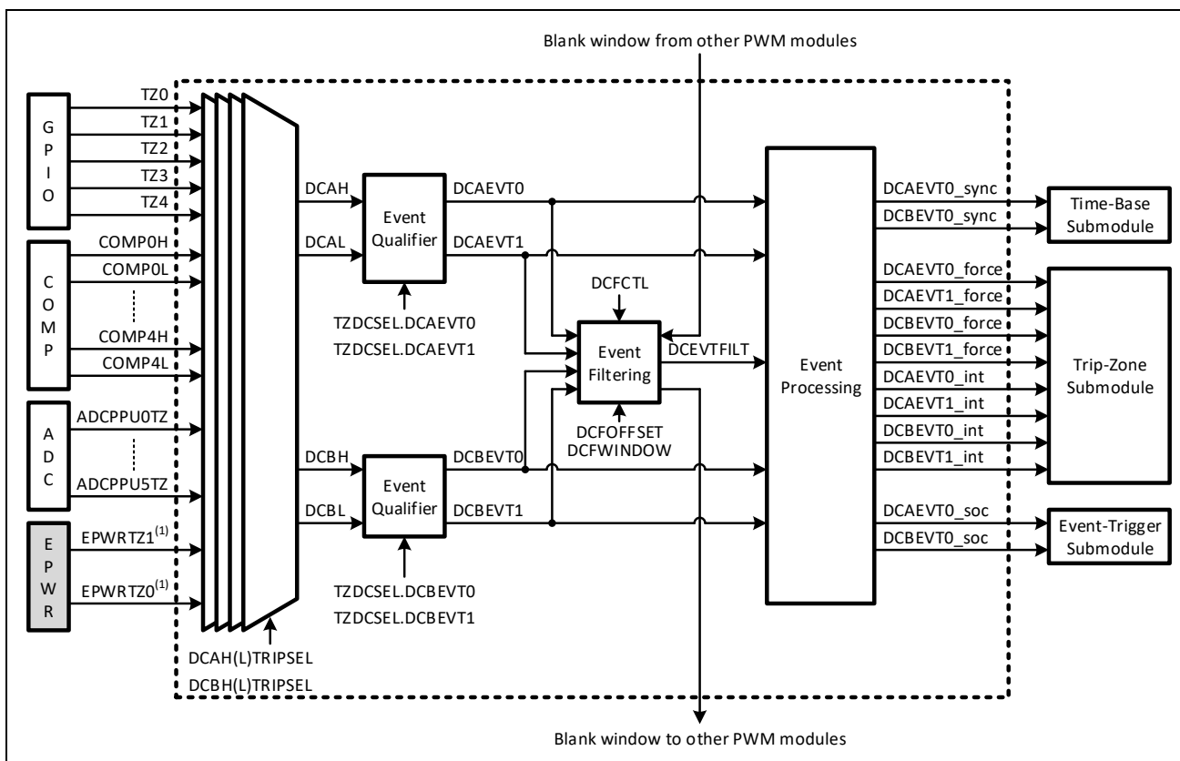
图 10-16：数字比较子模块结构
