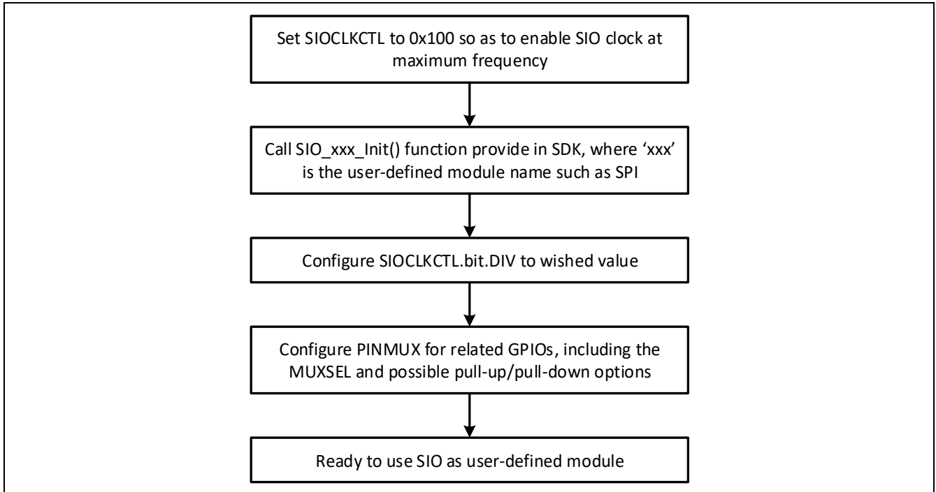
图 21-2: SIO 初始化流程
