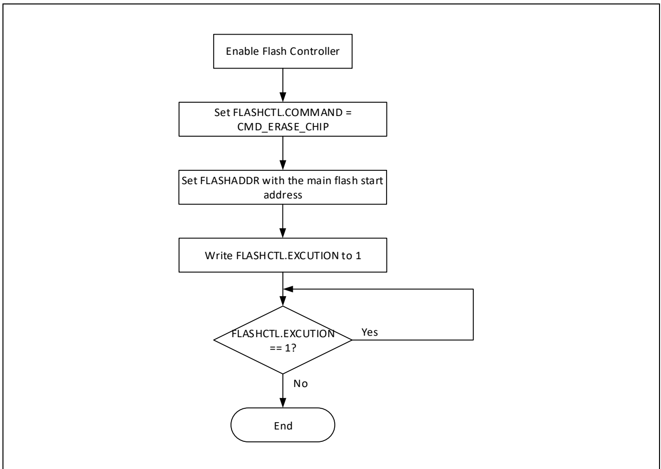
图 20-6: Flash 存储器整片擦除操作流程
