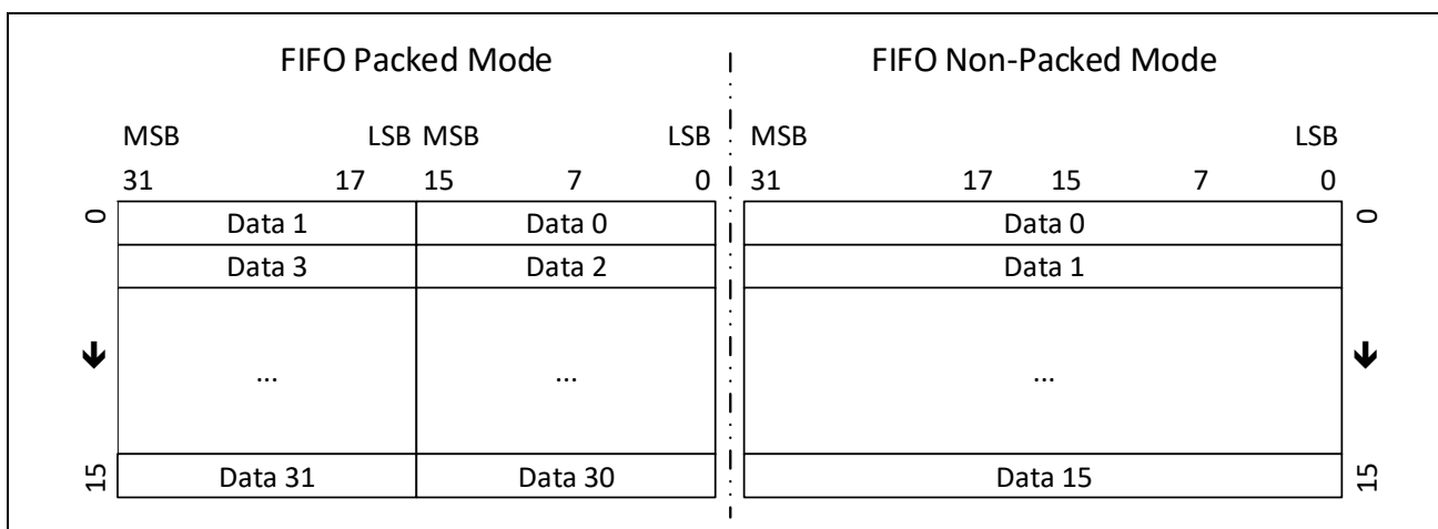
图 19-3: FIFO 压缩和非压缩模式
