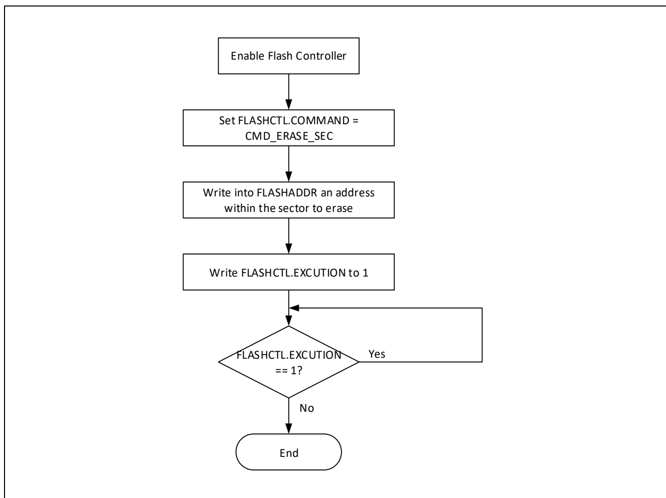
图 20-5: Flash 存储器扇区擦除操作流程
