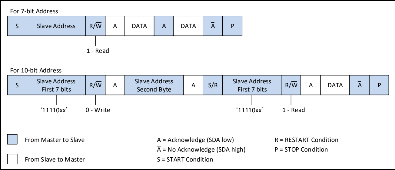
图 18-6: 主机-接收器协议
