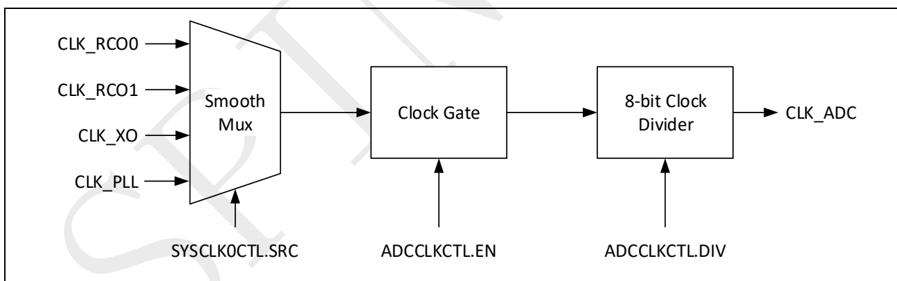
图 3-14：ADC 时钟控制框图
