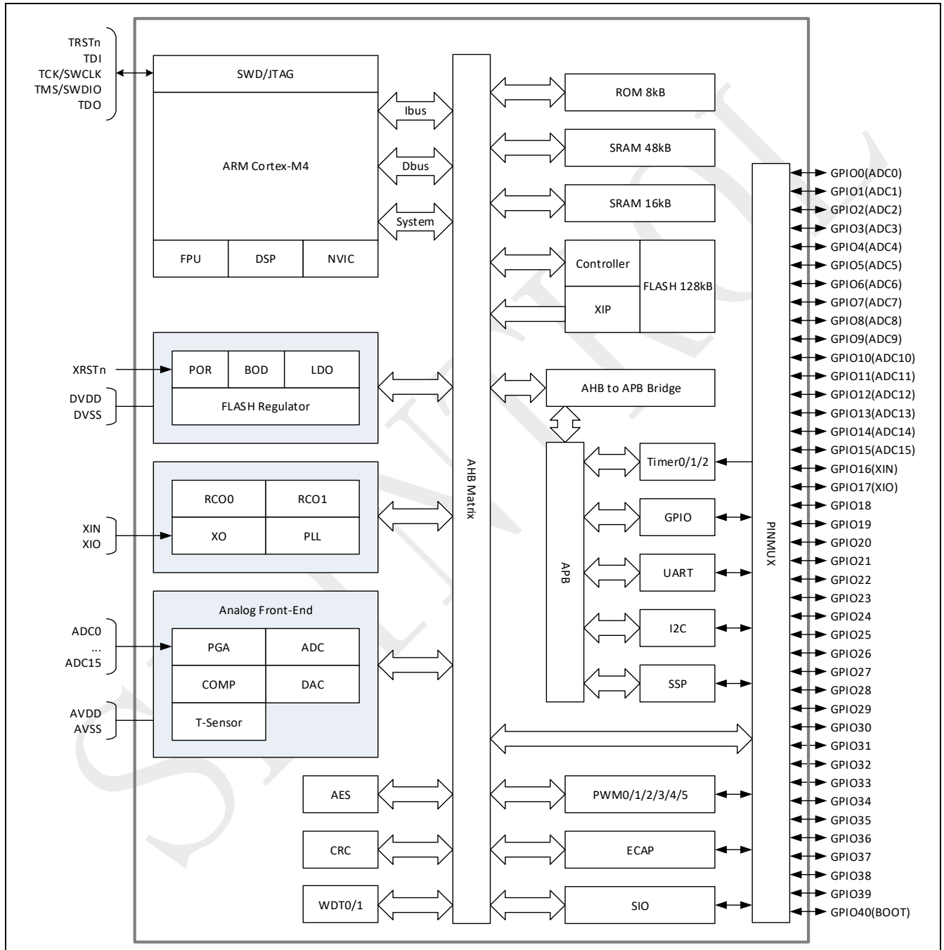
图 1-1: SPC1168 系统框图
