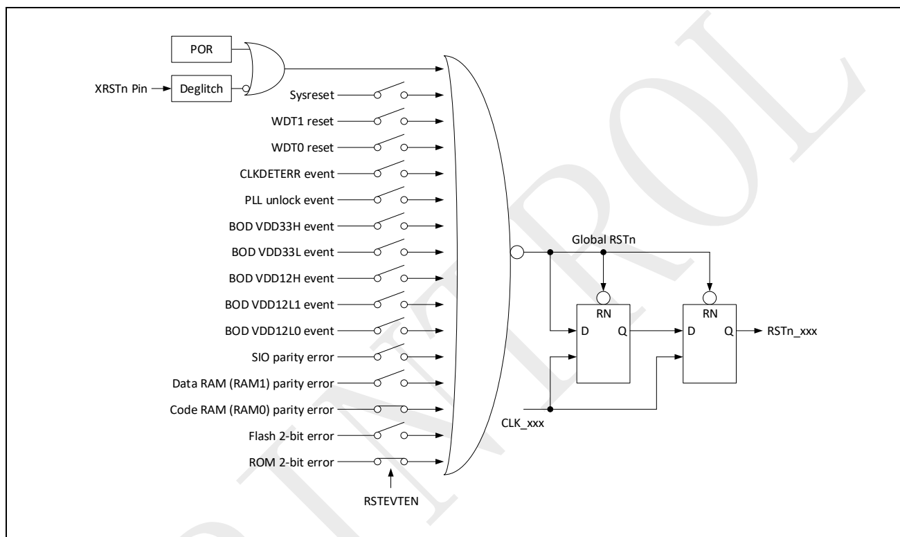
图 3-1：复位信号框图
