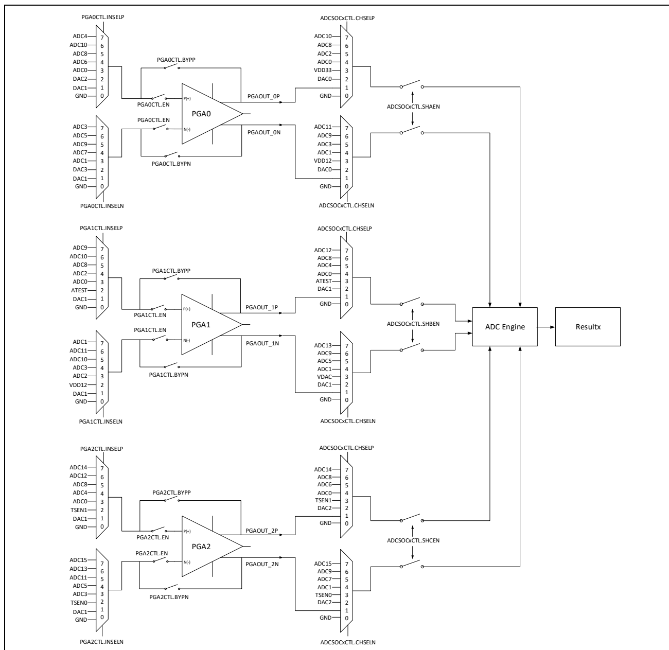
图 14-1: PGA 结构框图
