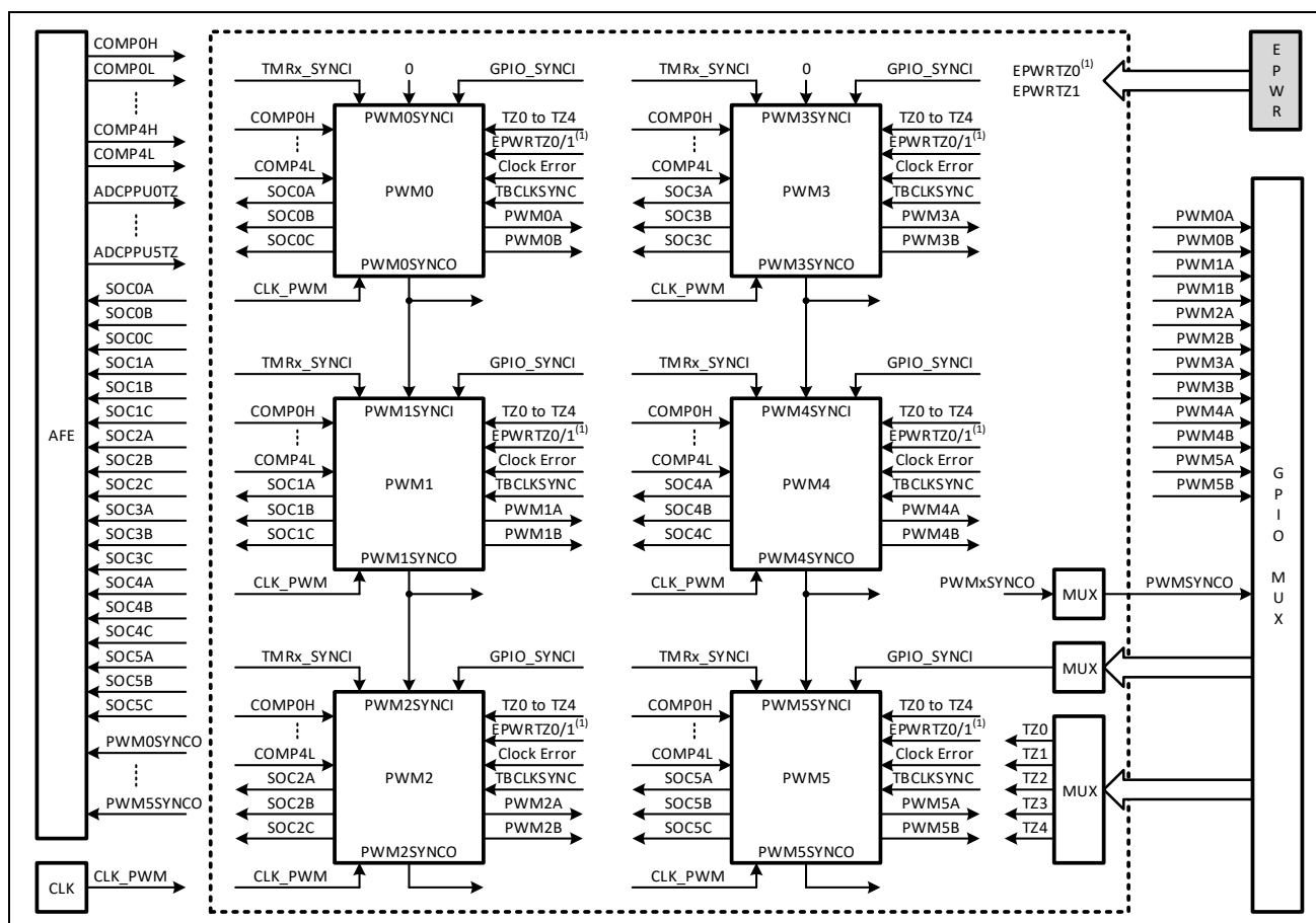
图 10-1: PWM 系统总览
