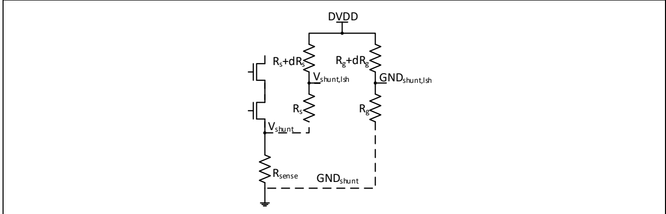
图 14-9：电平移位器电阻失配
