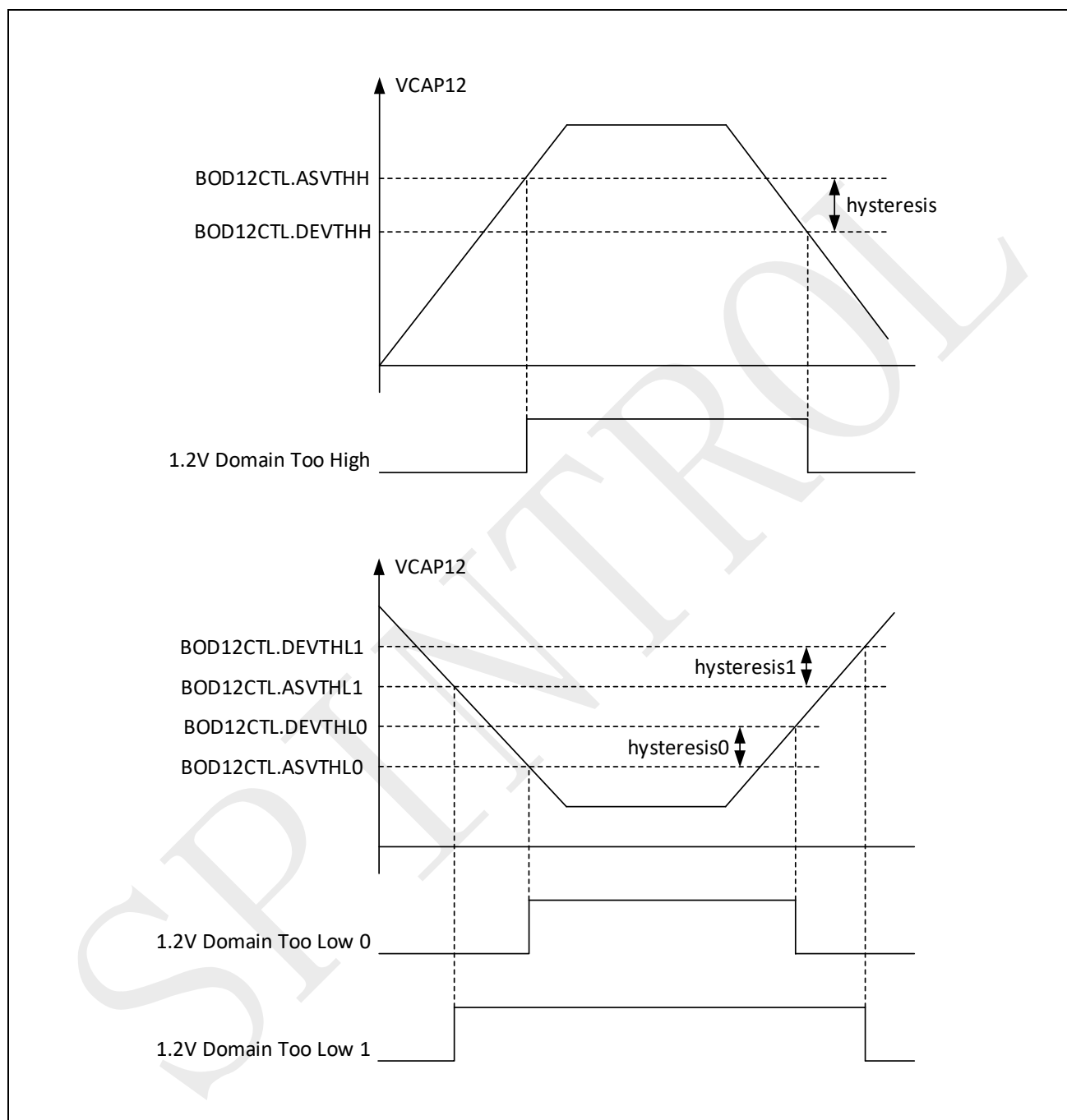
图 2-5: VCAP12 阈值
