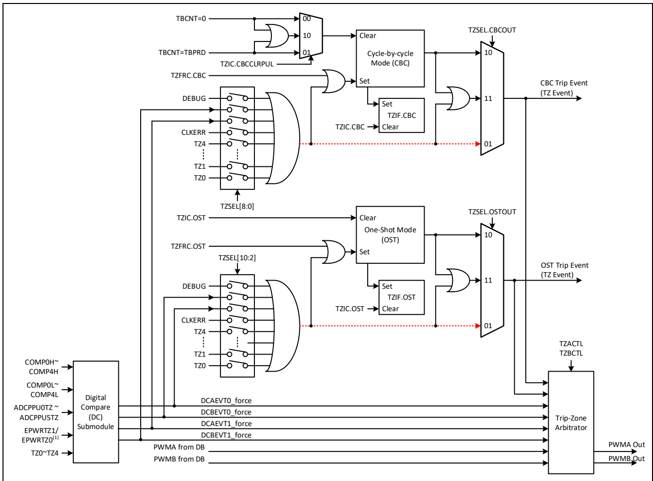
图 10-14：信号封锁子模块结构
