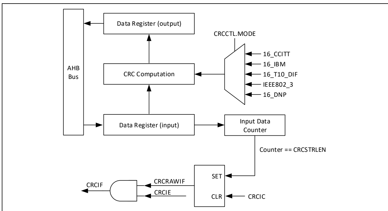
图 7-1：CRC 模块框图
