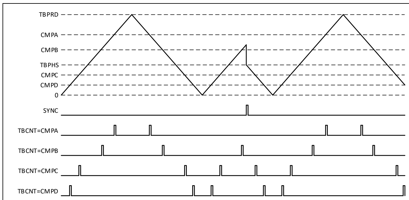
图 10-7：计数比较子模块波形
