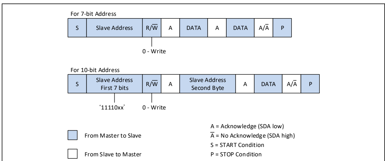
图 18-5: 主机-发送器协议
