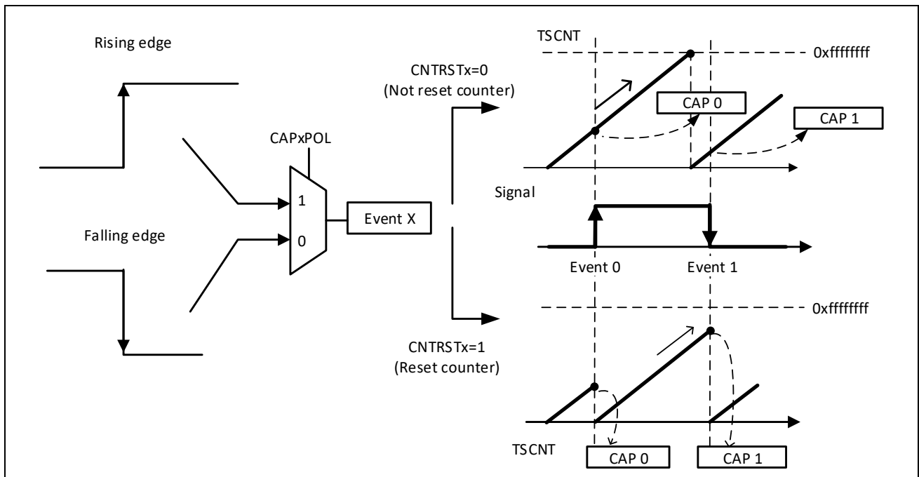
图 11-1: ECAP 基本工作方式
