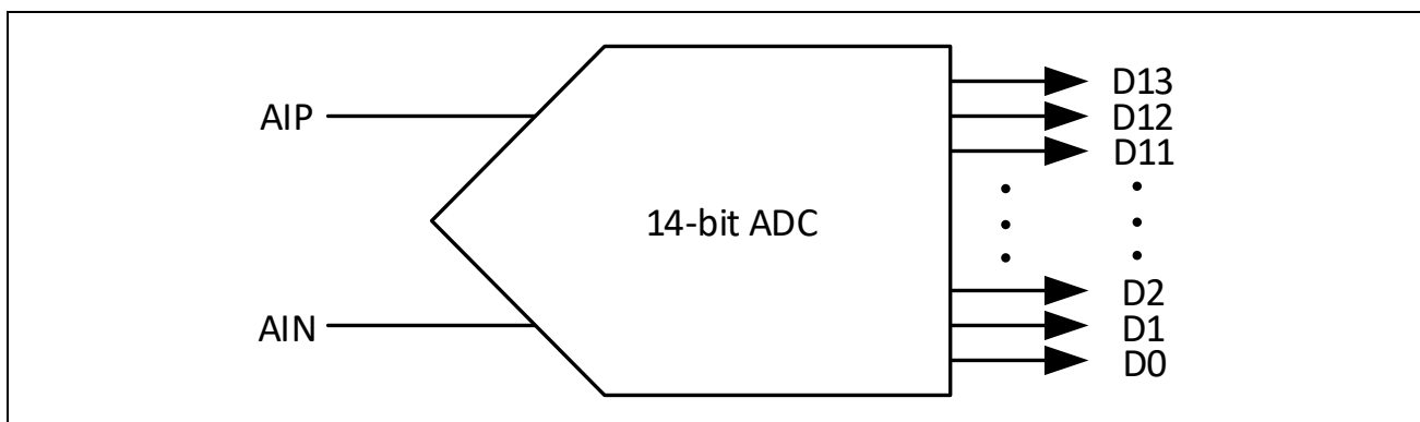
图 12-14：ADC 内核示意图
