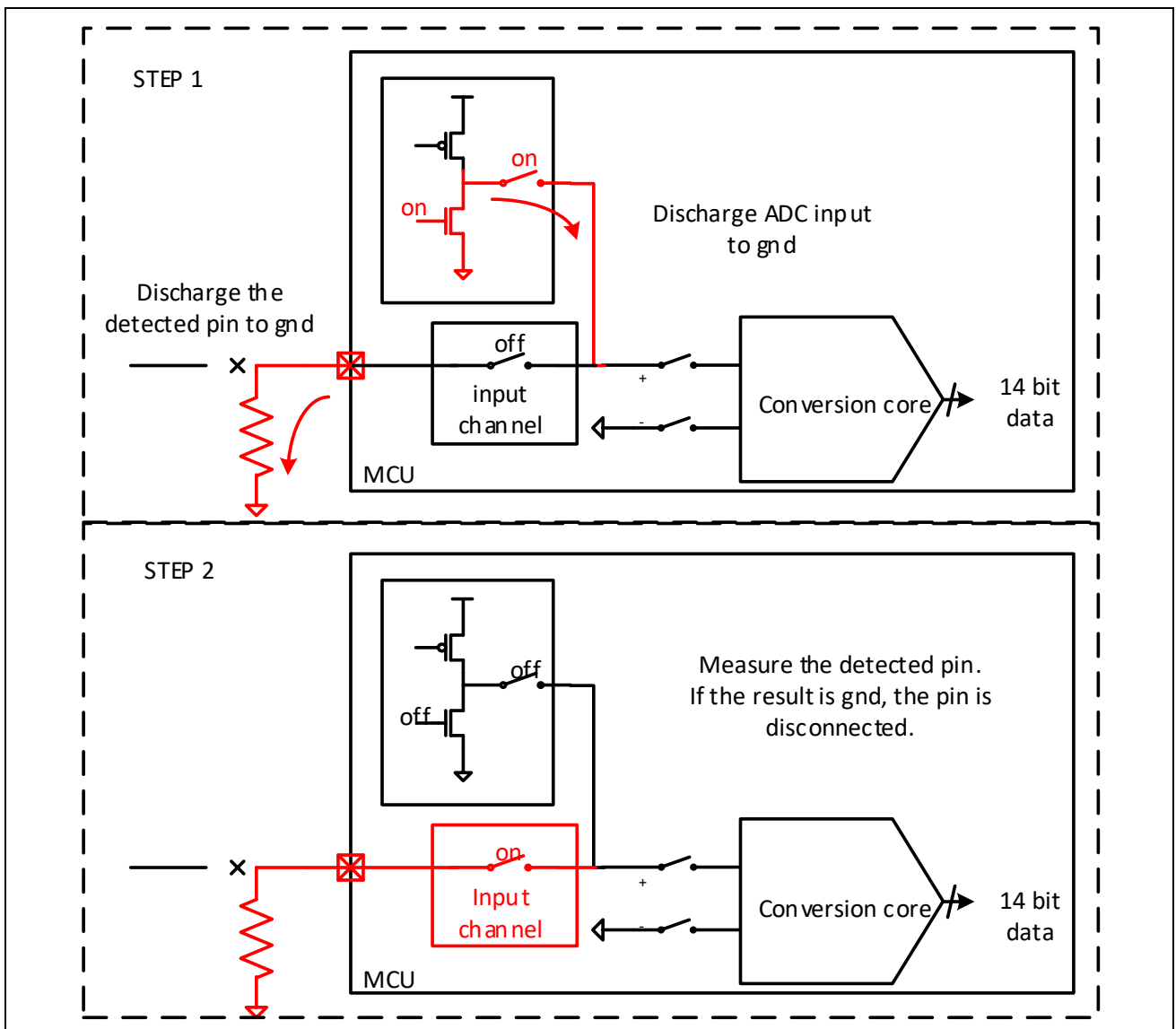
图 12-16：检测 ADC 输入 PIN 脚断路（放电）
