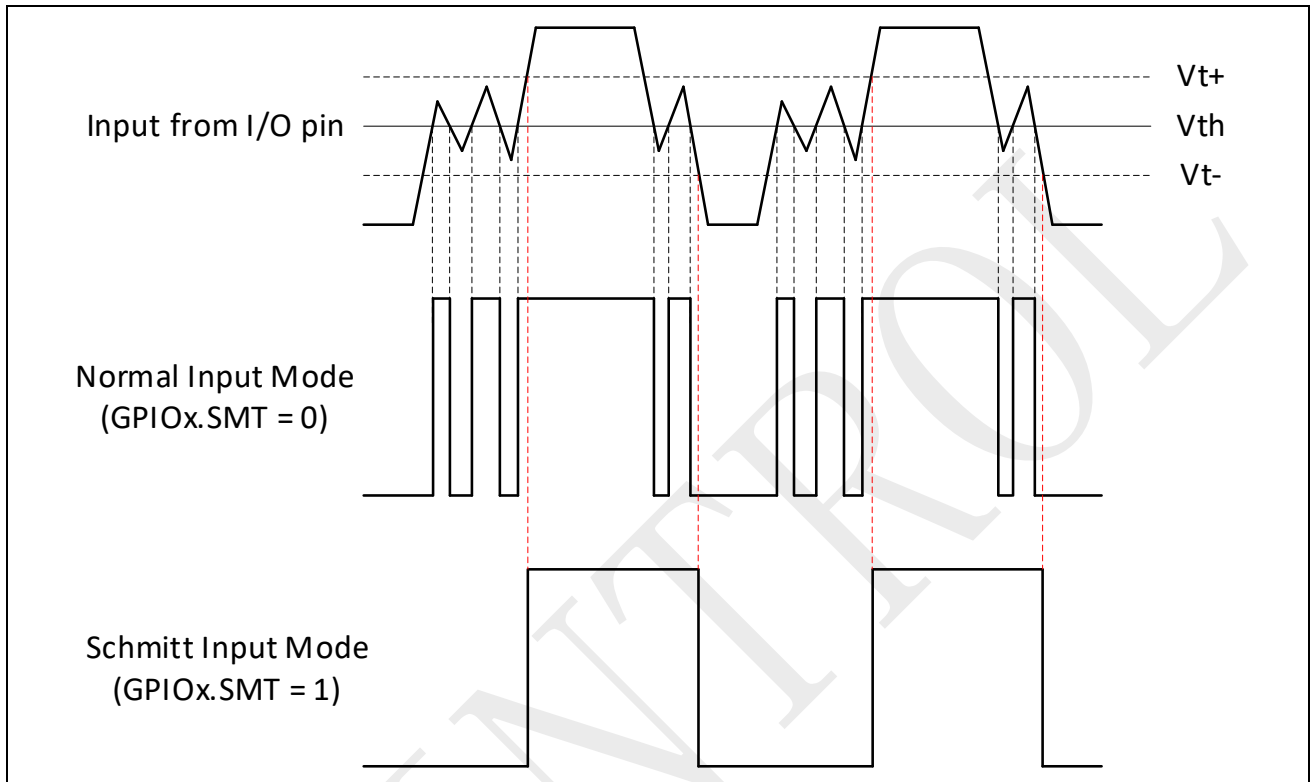
图 4-3：施密特输入模式
