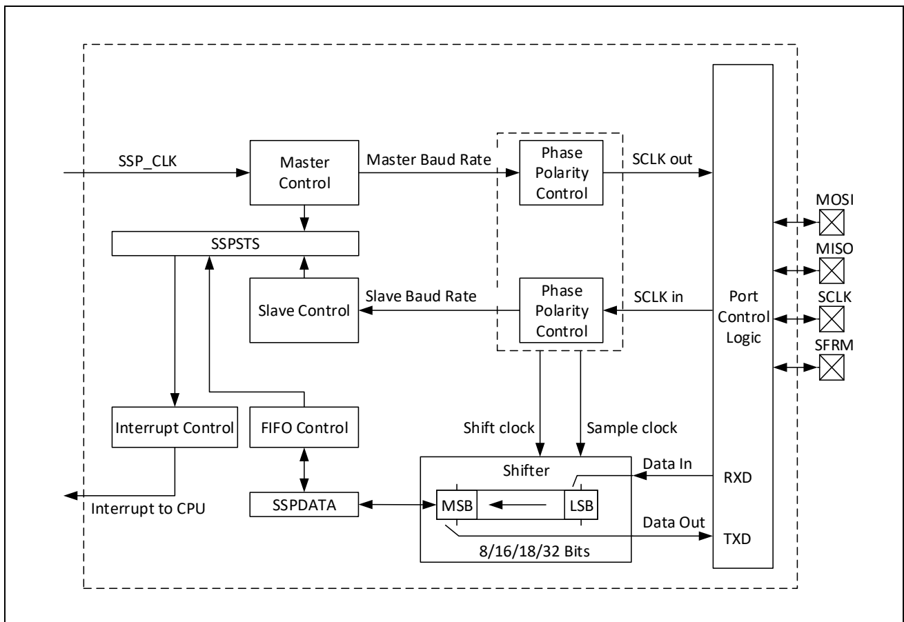
图 19-1: SSP 模块框图
