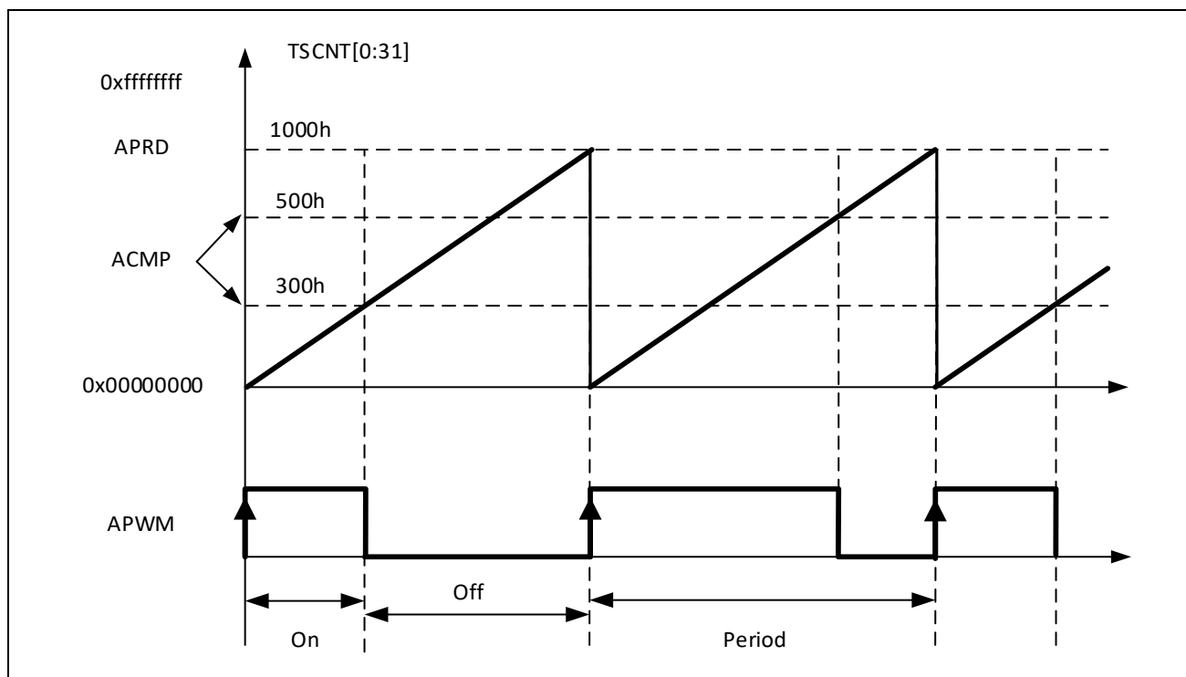
图 11-10: APWM 模式波形（极性为高有效）
