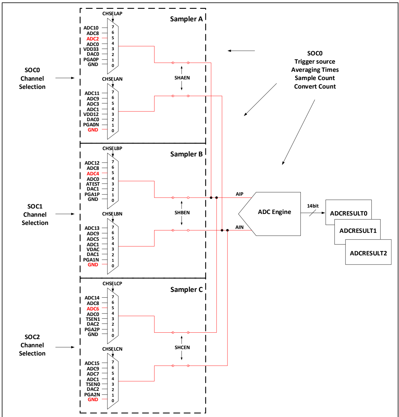
图 12-4: ADC2, ADC4 和 ADC6 三路并行采样
