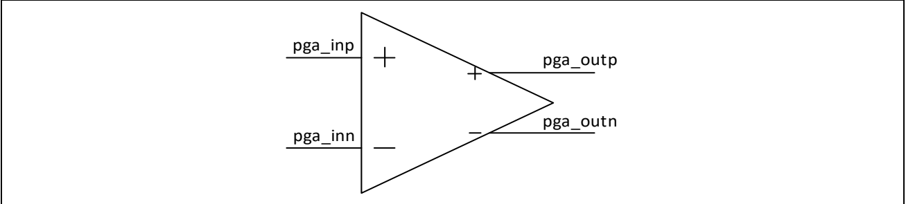
图 14-2: PGA 输入和输出
