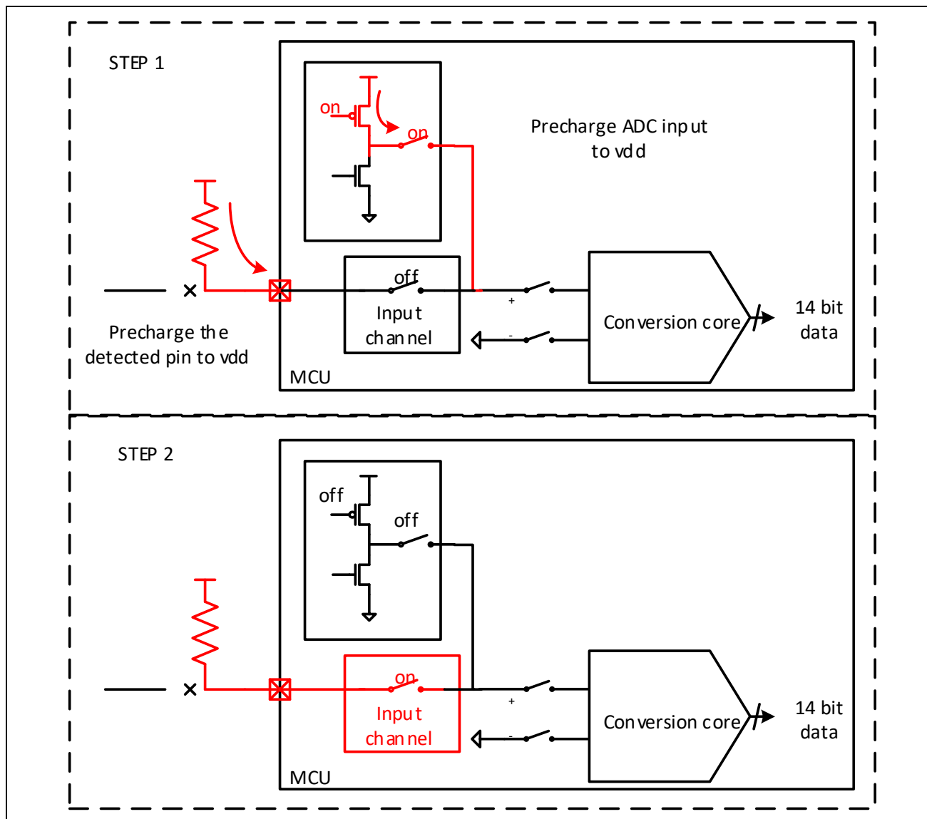
图 12-17: 检测 ADC 输入 PIN 脚断路（预充电）
