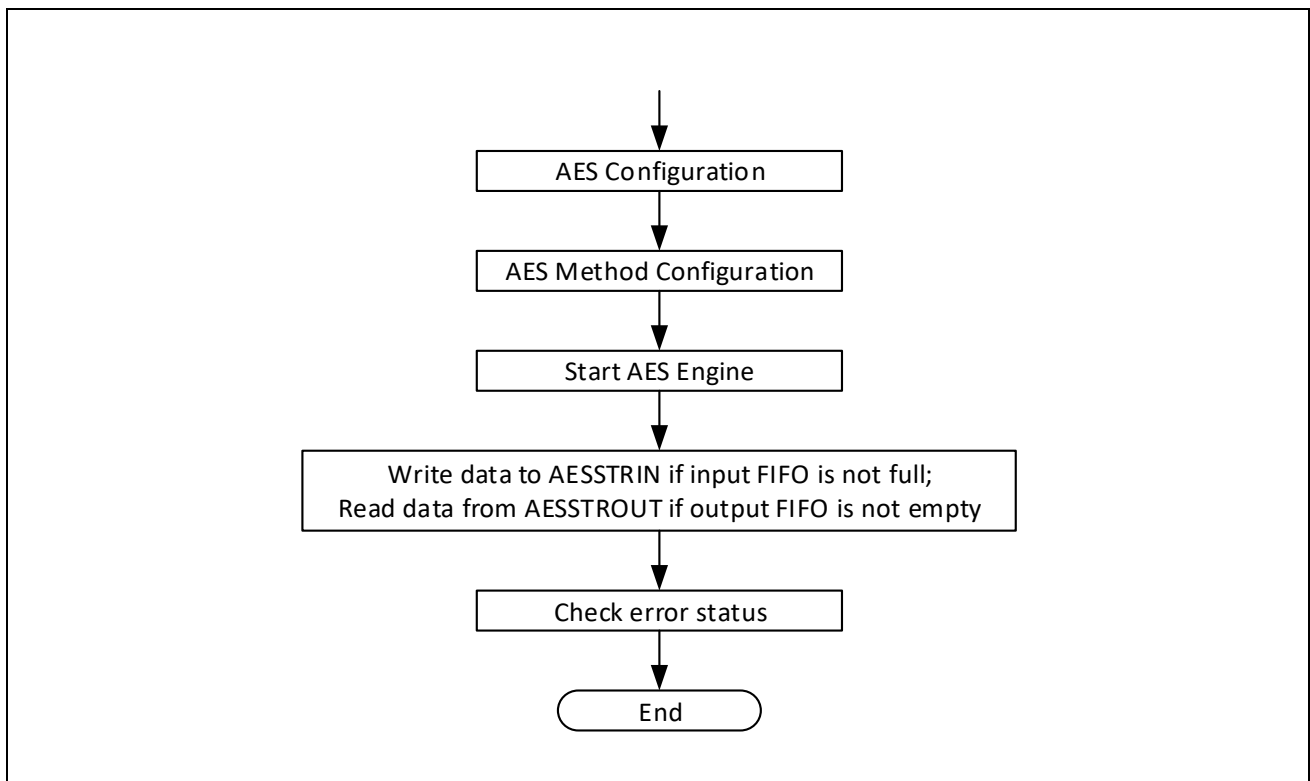
图 6-1: AES 工作流程图
