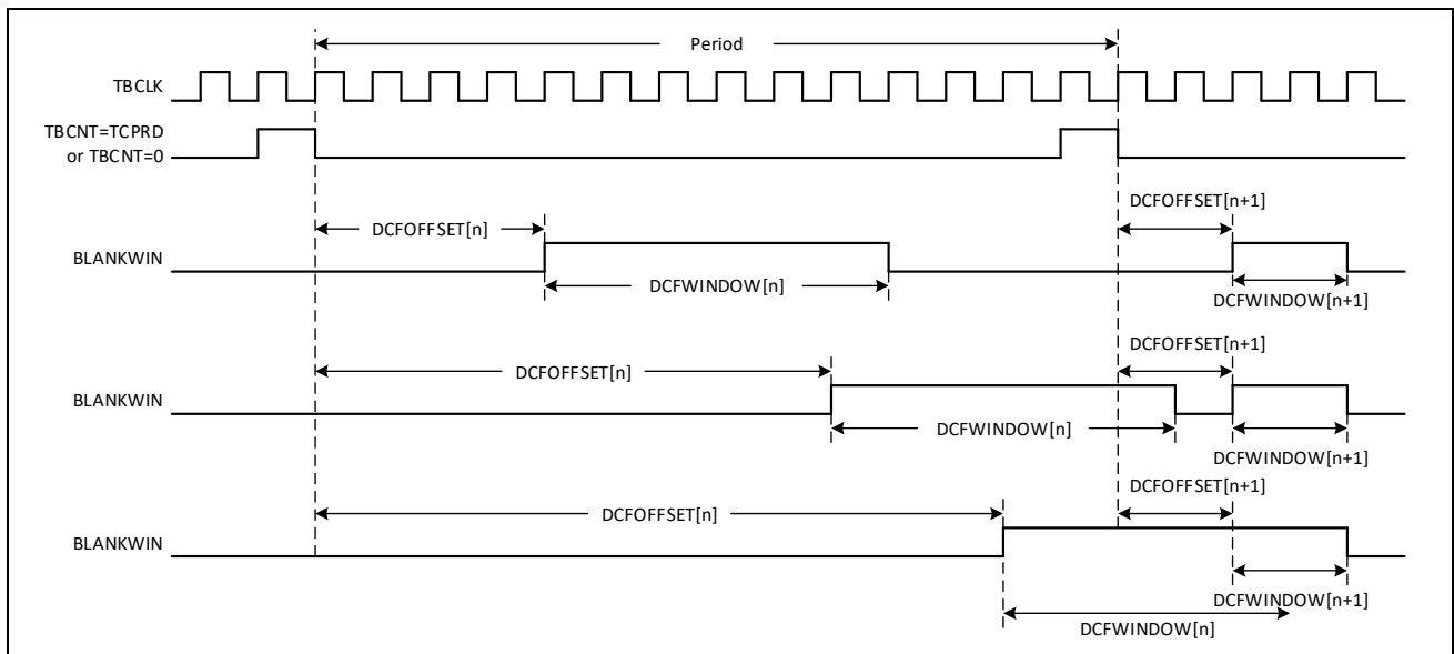
图 10-18: 消隐窗口时序图
