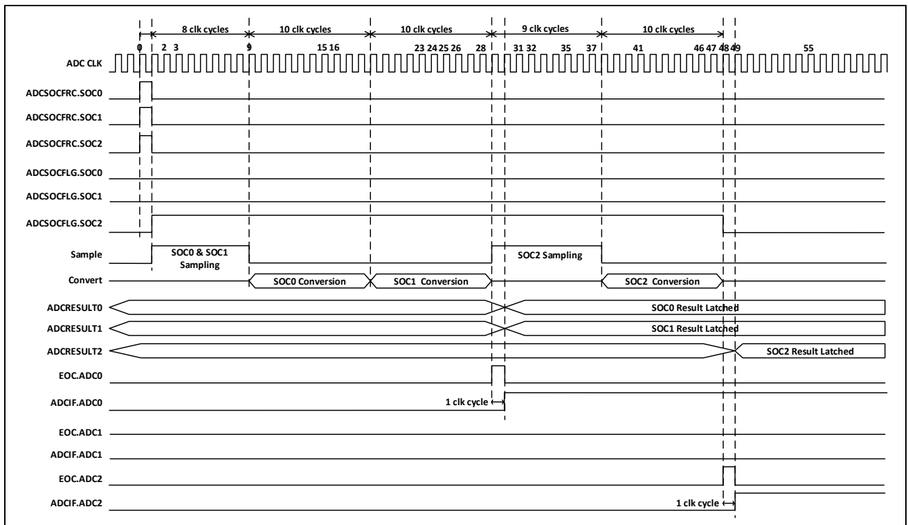
图 12-13: 同时采样模式时序
