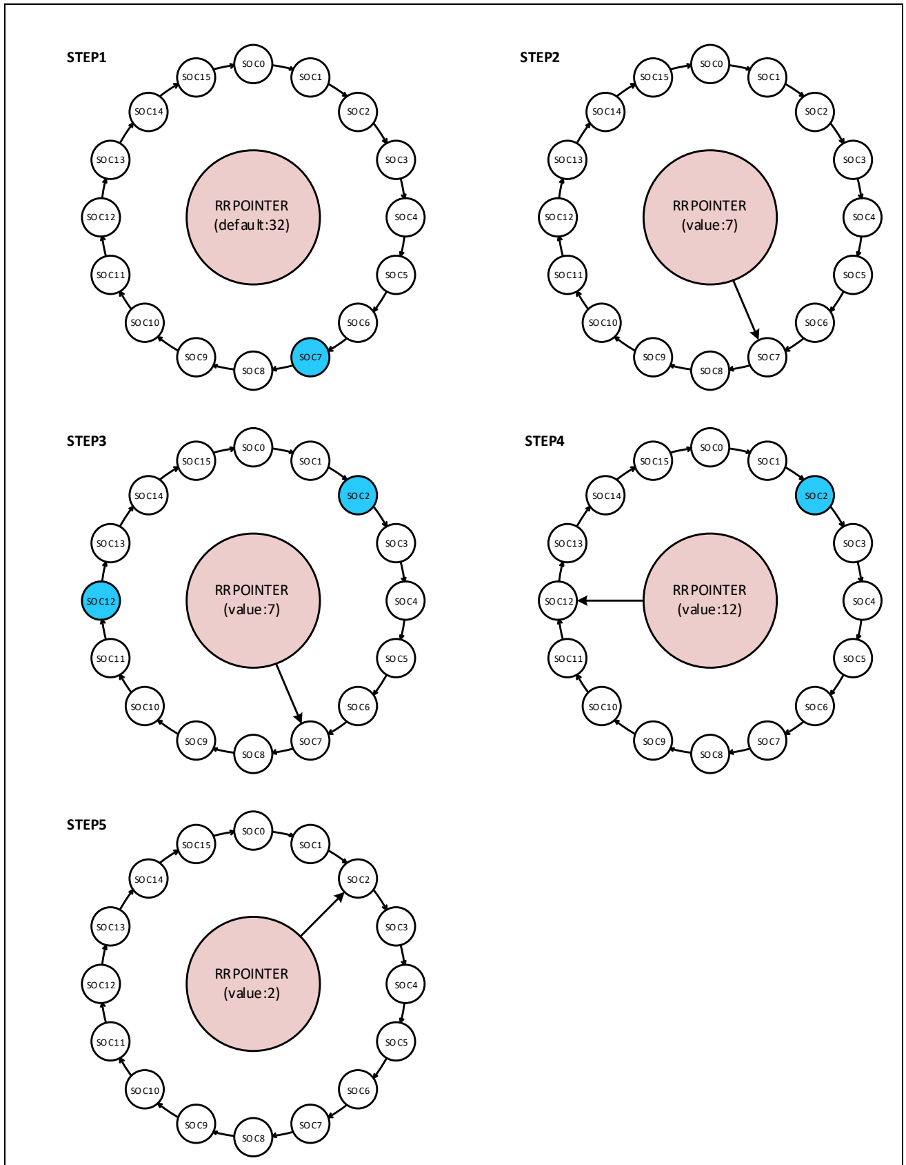
图 12-7: Round-Robin 环优先级示例
