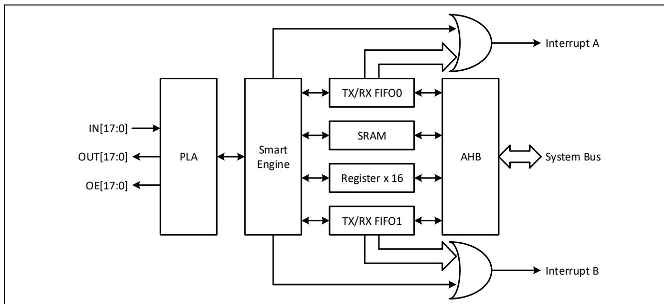
图 21-1: SIO 架构原理图
