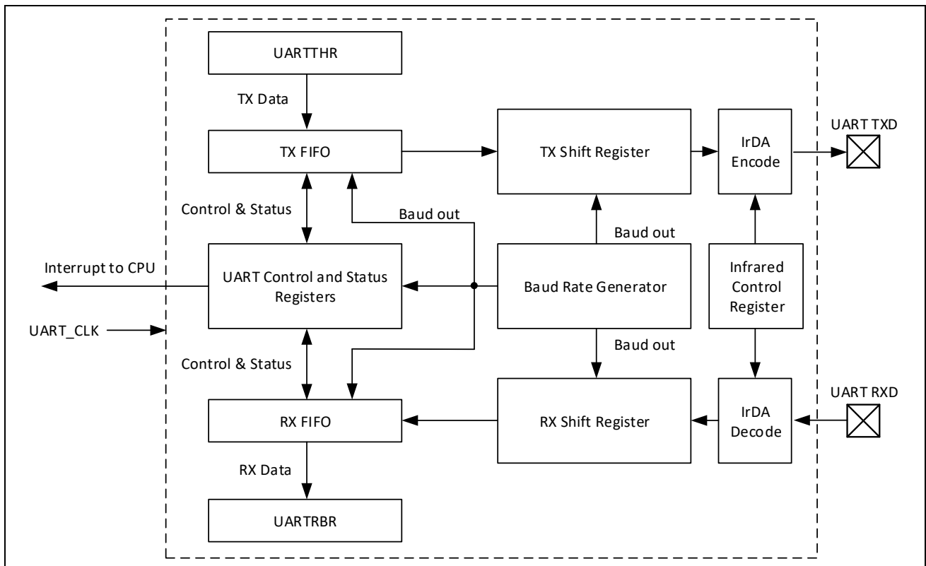
图 17-1: UART 模块框图
