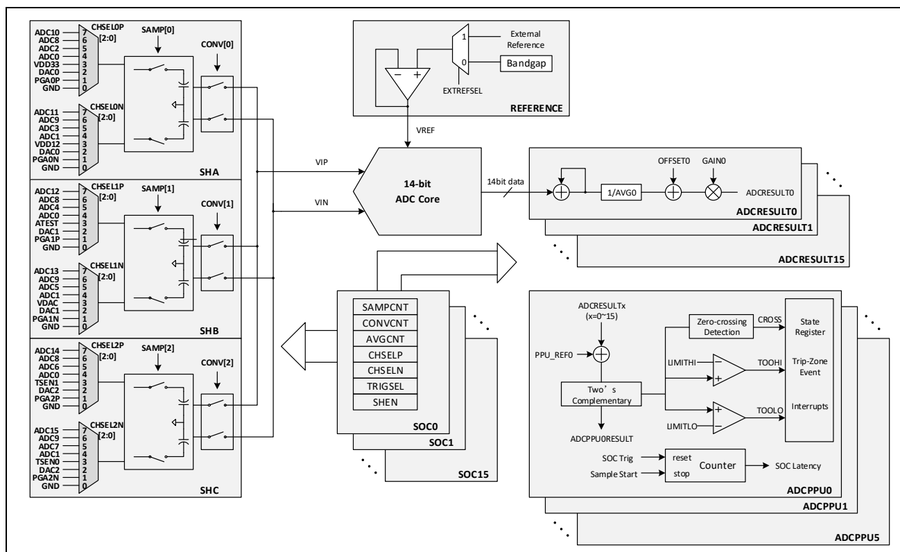
图 12-1: ADC 内部模块框图
