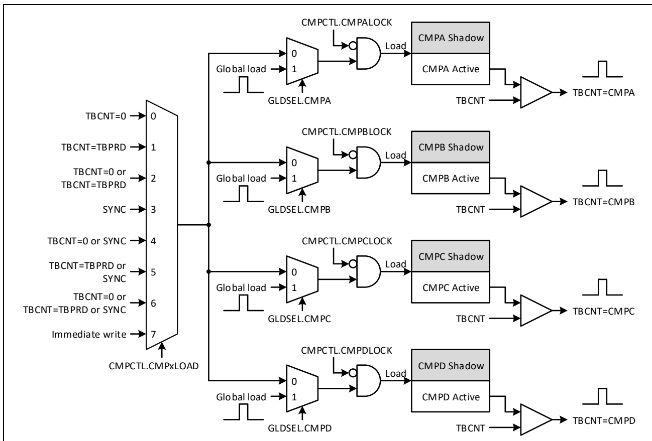
图 10-6：计数比较子模块结构
