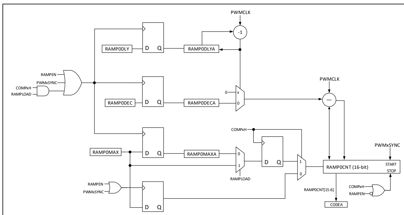
图 16-2: Ramp 发生器框图
