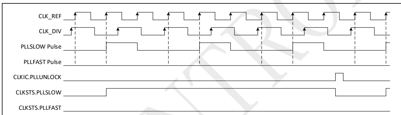
图 3-7: PLL 失锁检测时序图示例（FREF > FDIV）
