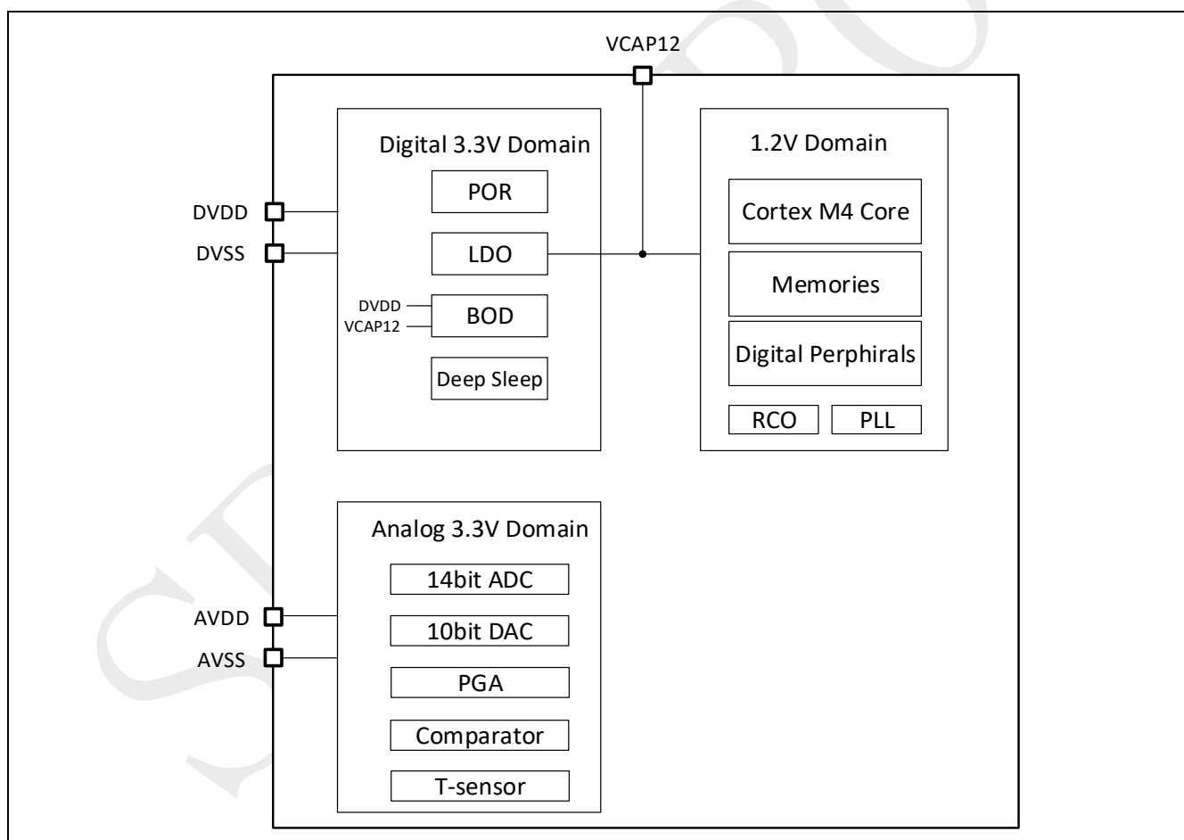
图 2-1: 电源系统总览
