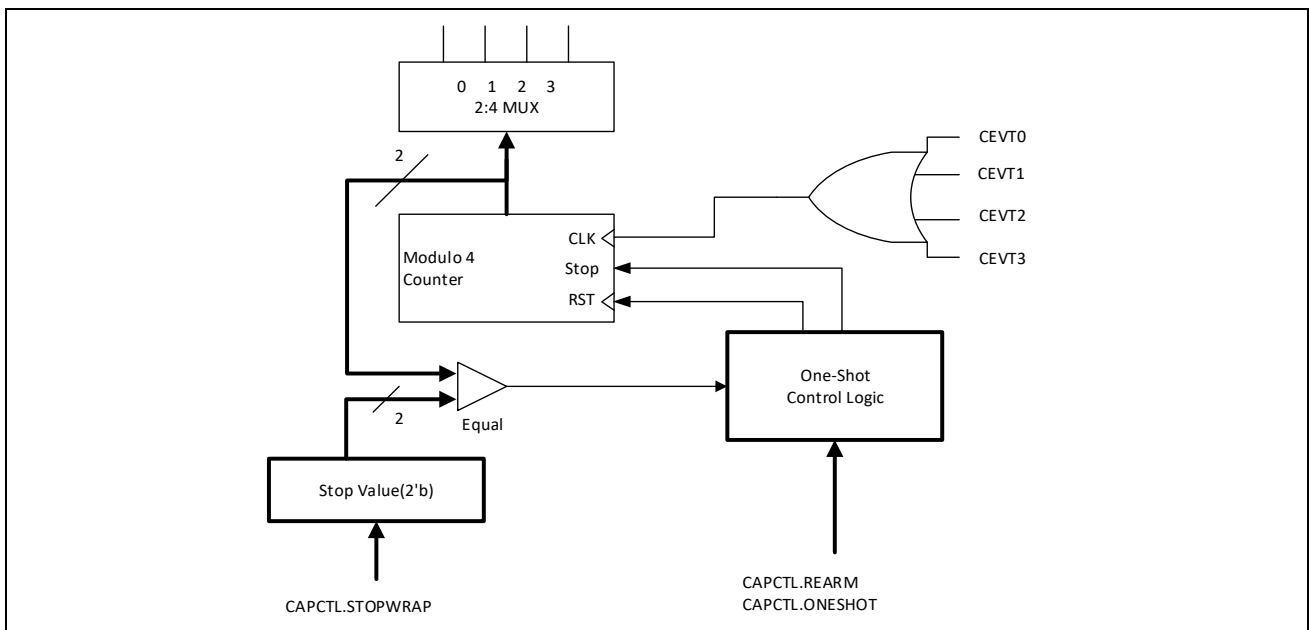
图 11-6: 持续捕获和一次性捕获逻辑
