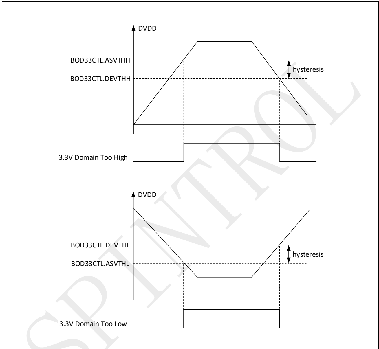
图 2-4: DVDD 阈值
