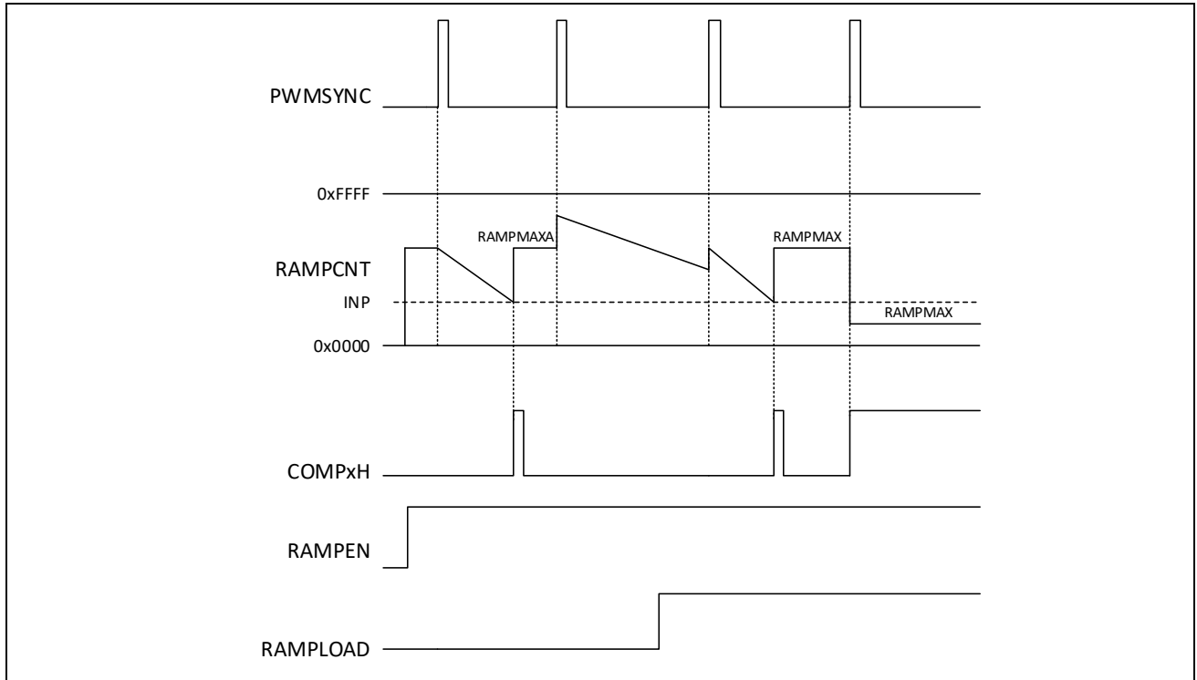
图 16-3: Ramp 发生器波形
