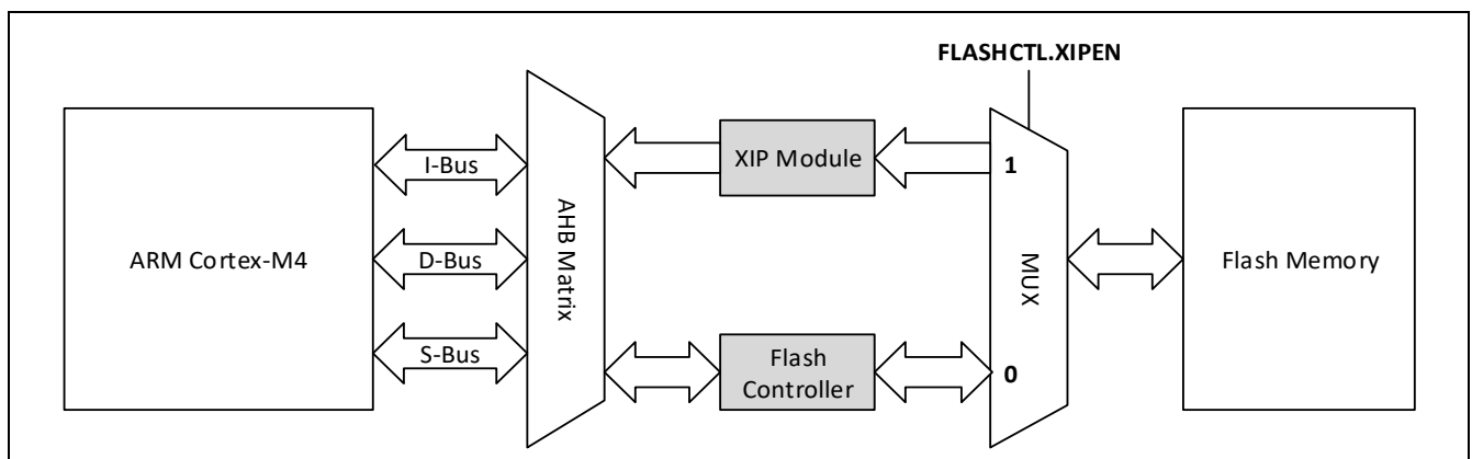
图 20-1：Flash 存储器访问接口
