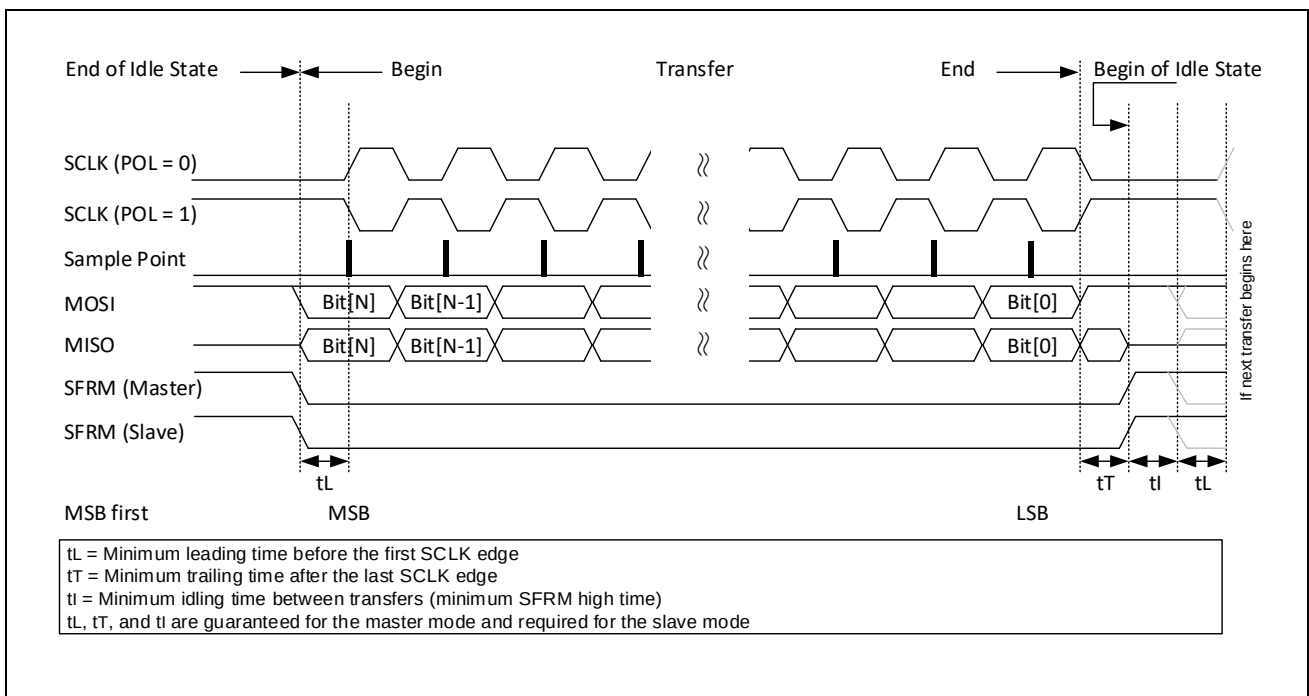
图 19-4：SSP 时钟格式 0（PHS = 0）
