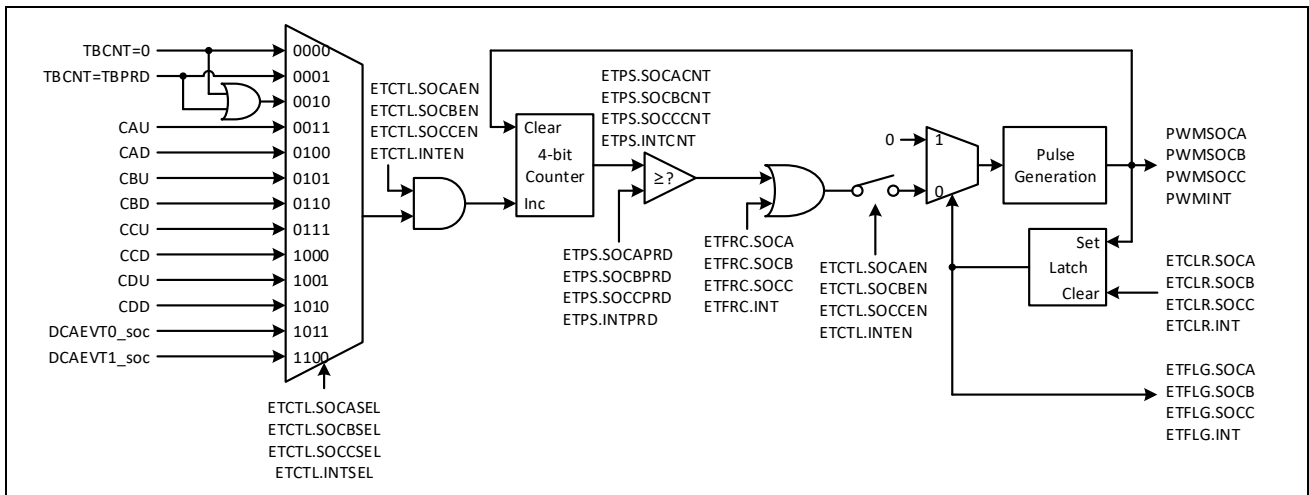
图 10-20：事件触发子模块结构
