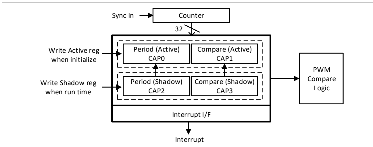
图 11-9：APWM 模式下 PRD 和 CMP 的有效值和影子值
