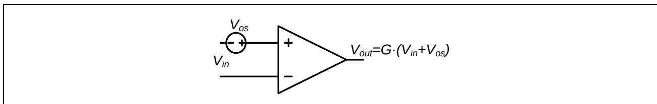
图 14-7: PGA 偏移误差
