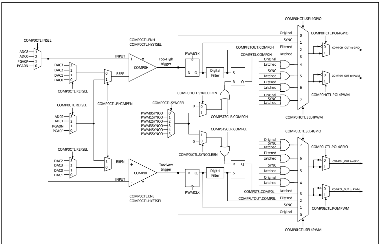
图 15-1：比较器 COMP0 框图
