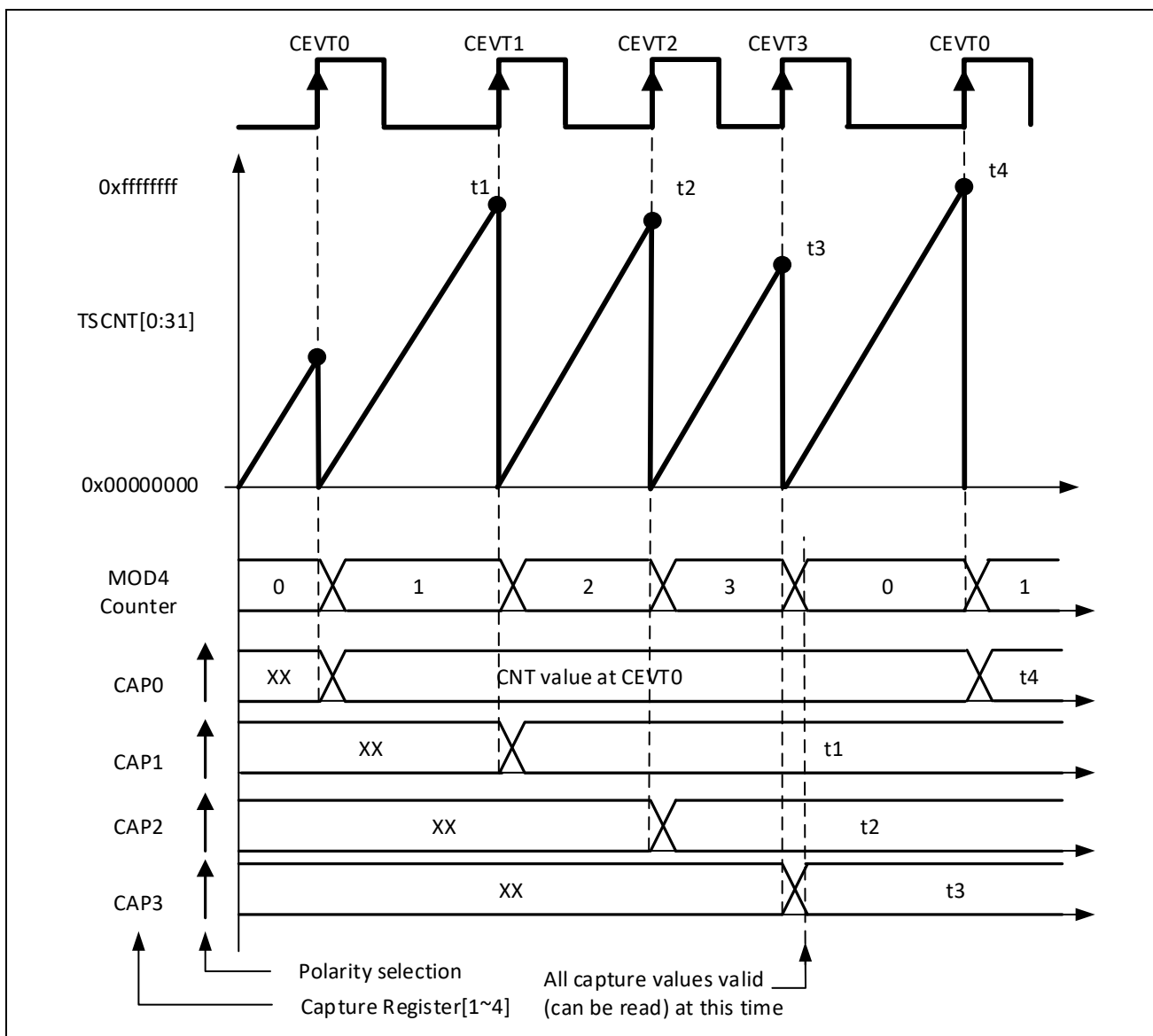
图 11-13：通过计数器复位捕获周期
