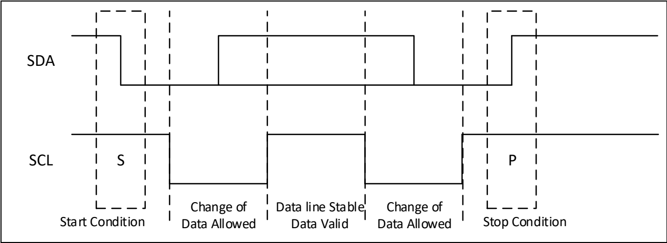
图 18-2: START 和 STOP 信号
