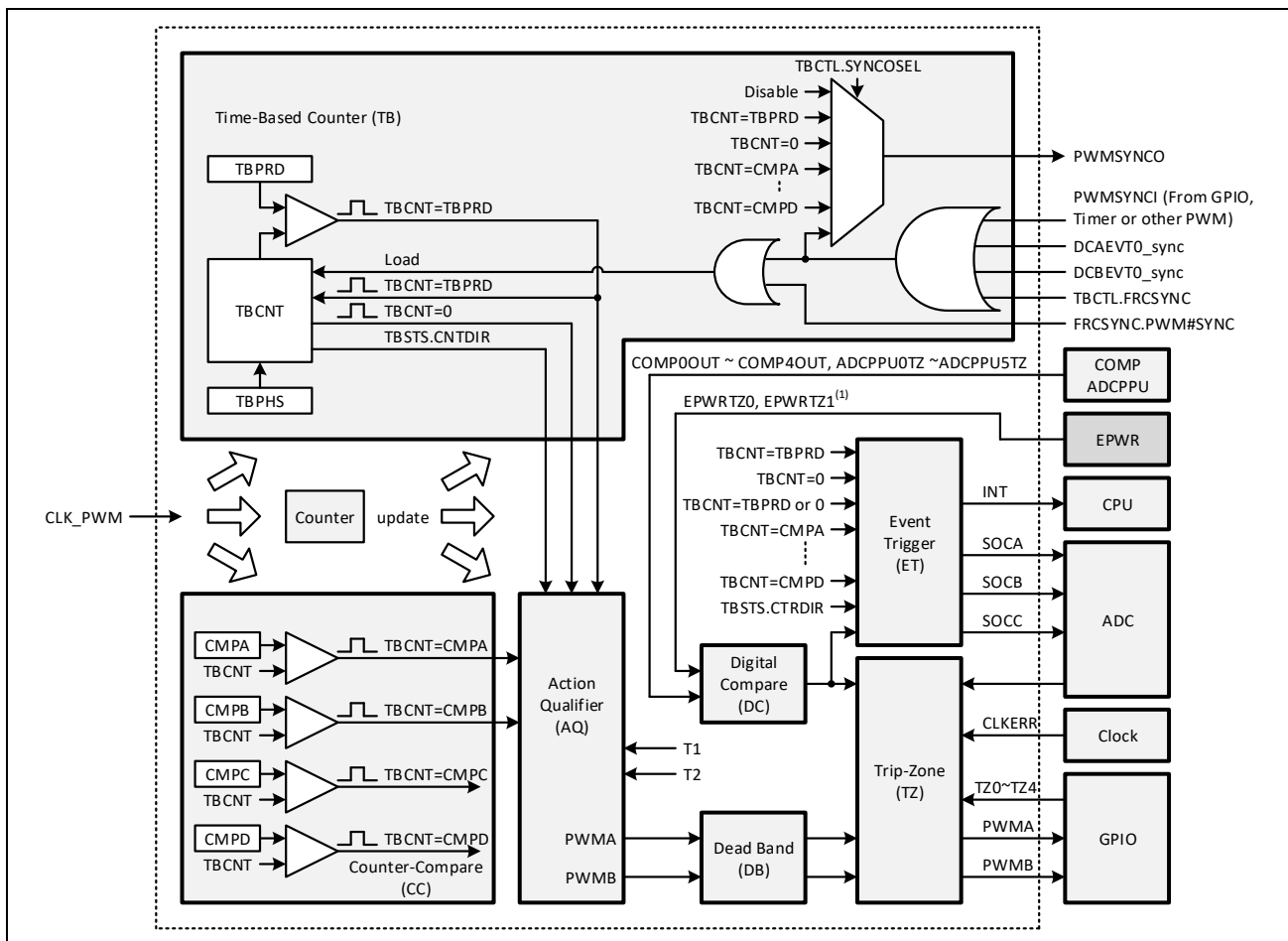
图 10-2: PWM 内部结构
