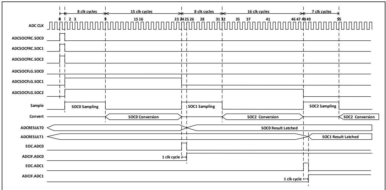
图 12-12: 顺序转换模式时序
