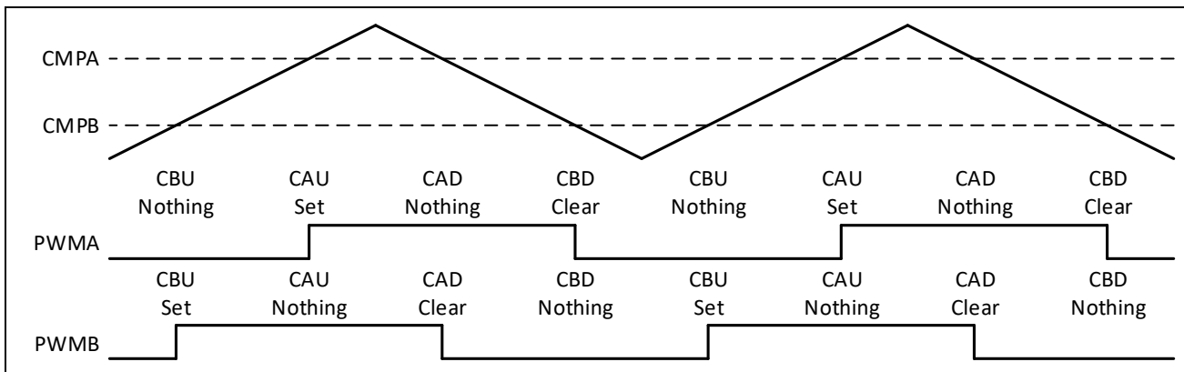
图 10-10: 上下计数时的 PWM 双边沿非对称波形
