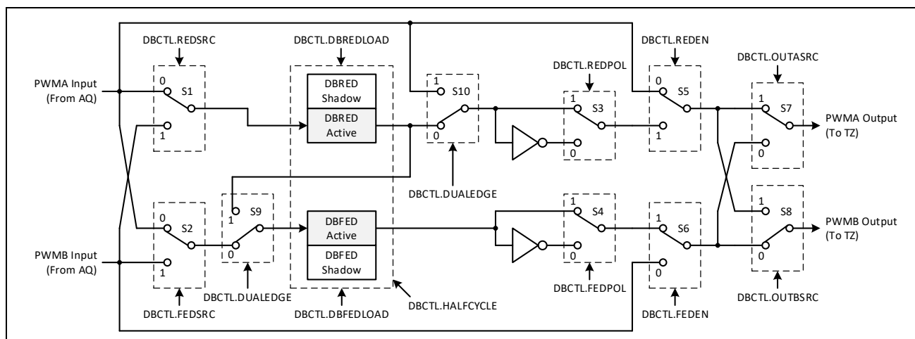
图 10-11: 死区控制子模块结构
