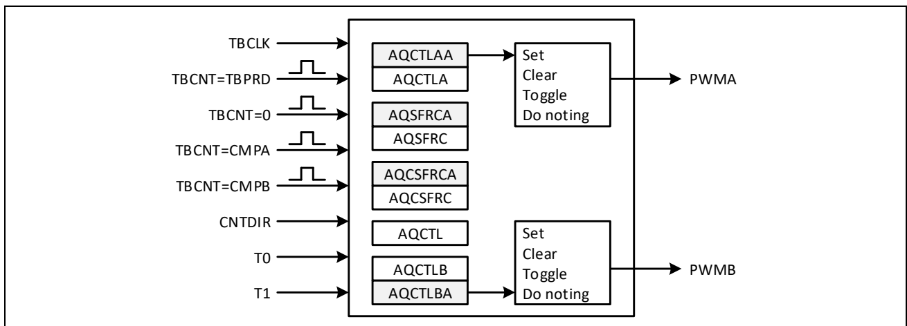
图 10-8：行为限定子模块输入输出
