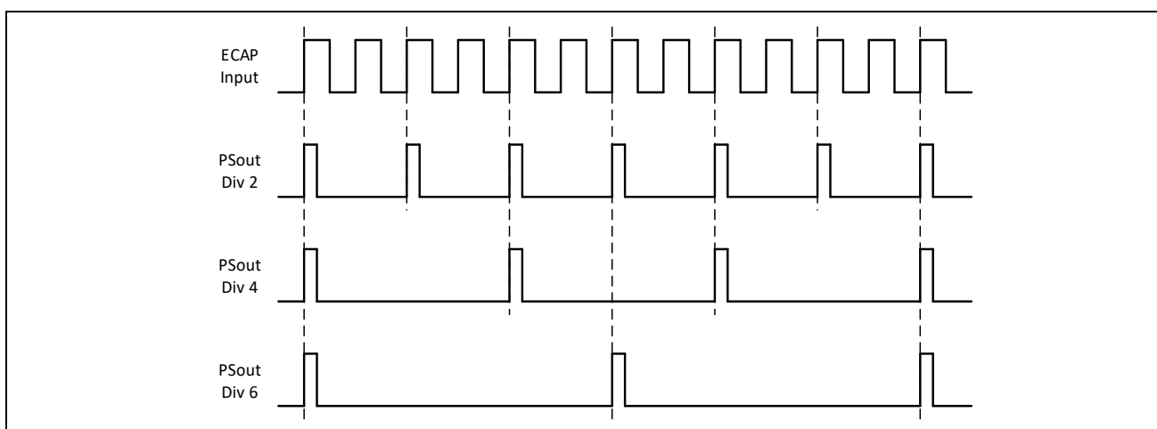
图 11-5: 事件预分频波形
