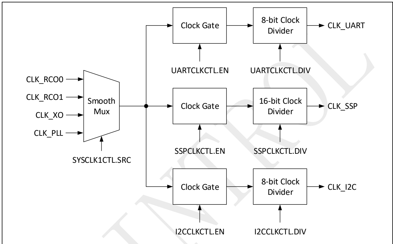
图 3-11：通讯外设时钟控制框图
