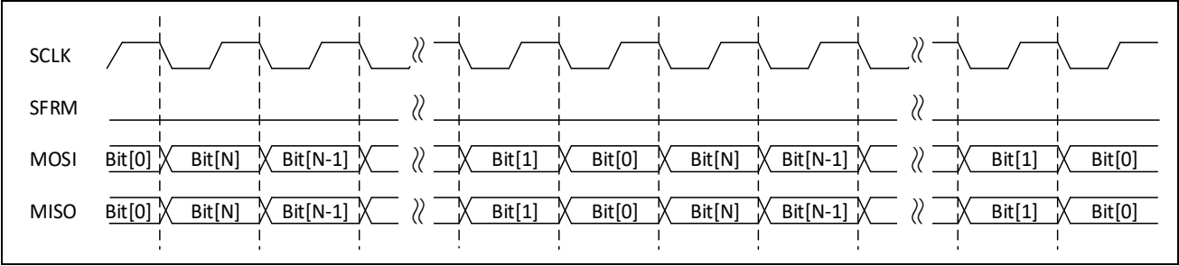
图 19-6: Motorola SPI 帧协议（多帧传输）
