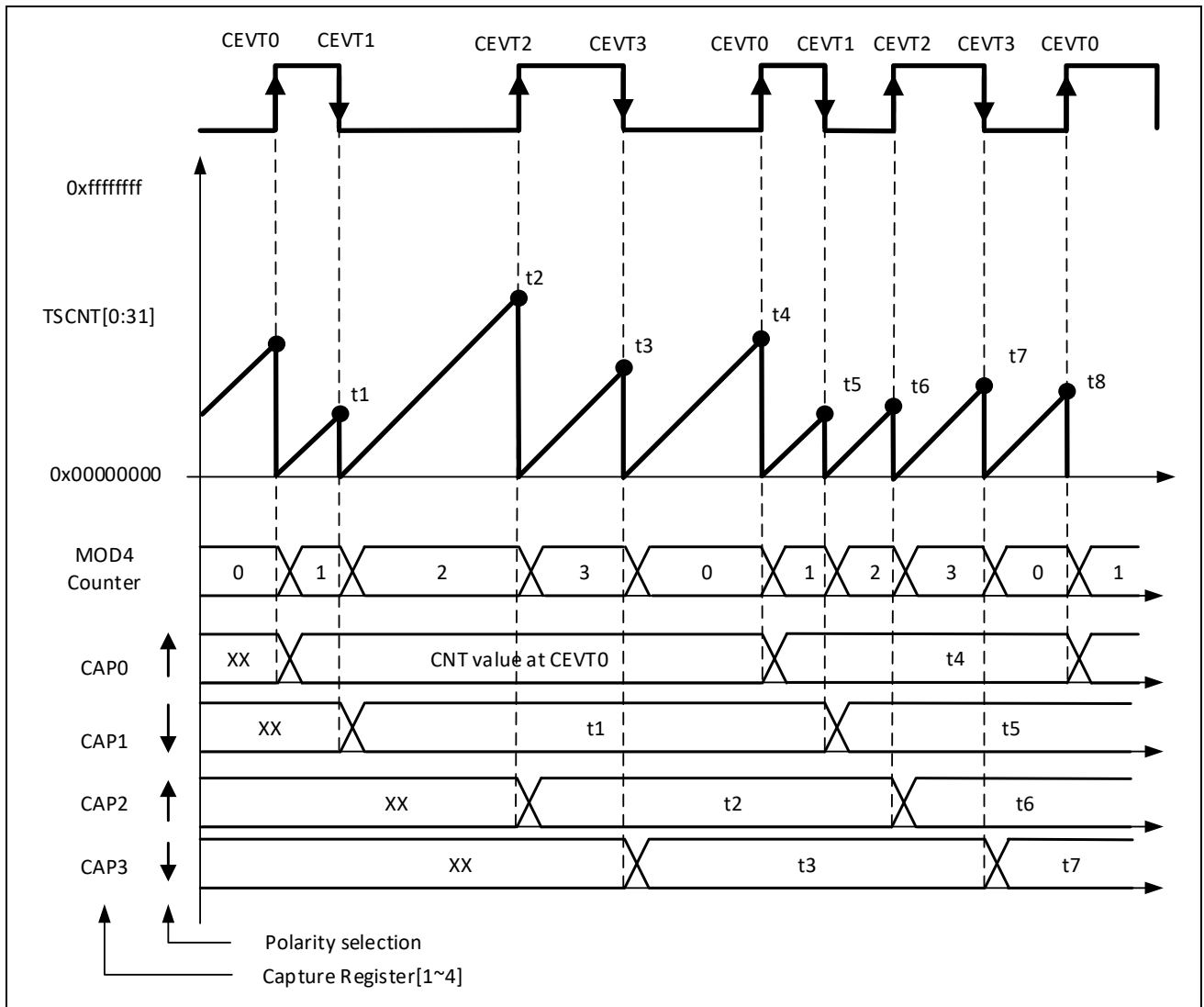
图 11-14：通过相对时间模式计数器复位捕获周期和占空
