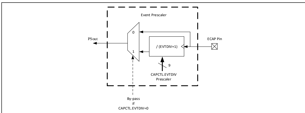
图 11-4: 事件预分频控制
