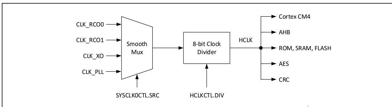
图 3-8: HCLK 控制框图
