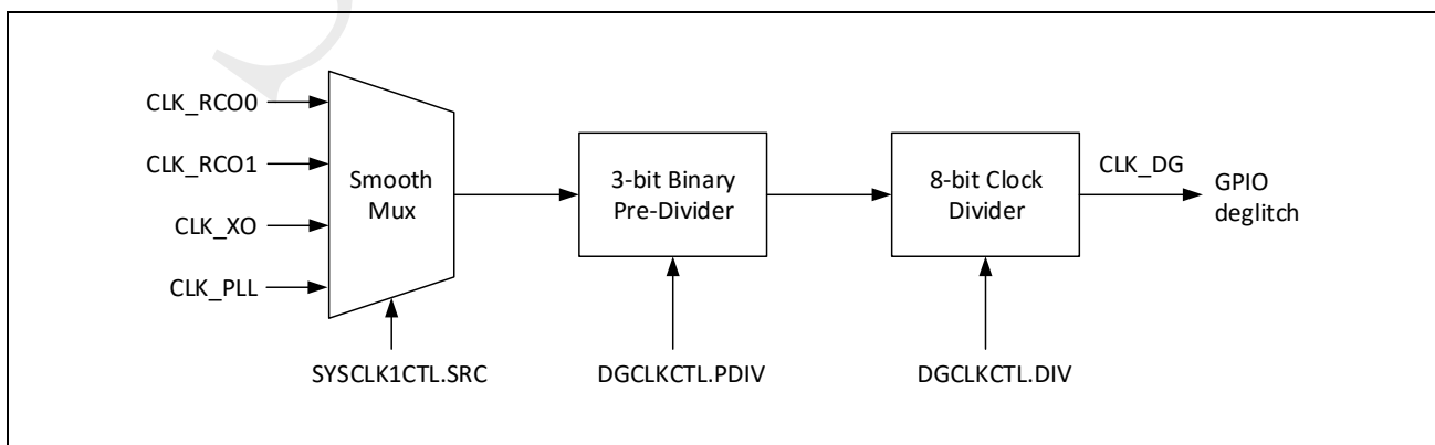
图 3-10: GPIO 消抖时钟控制框图
