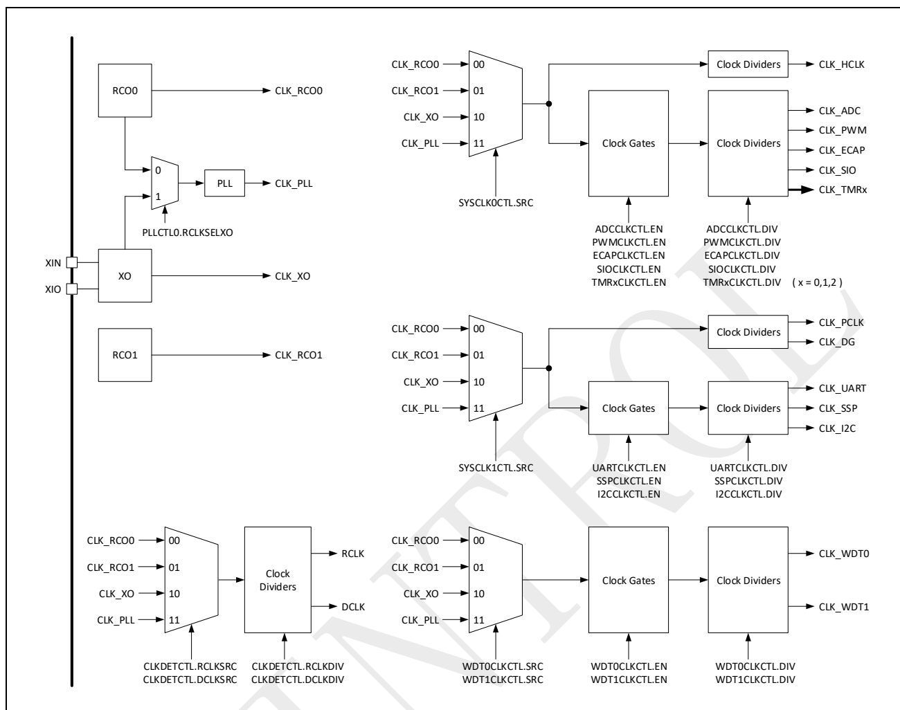
图 3-3: 时钟结构图
