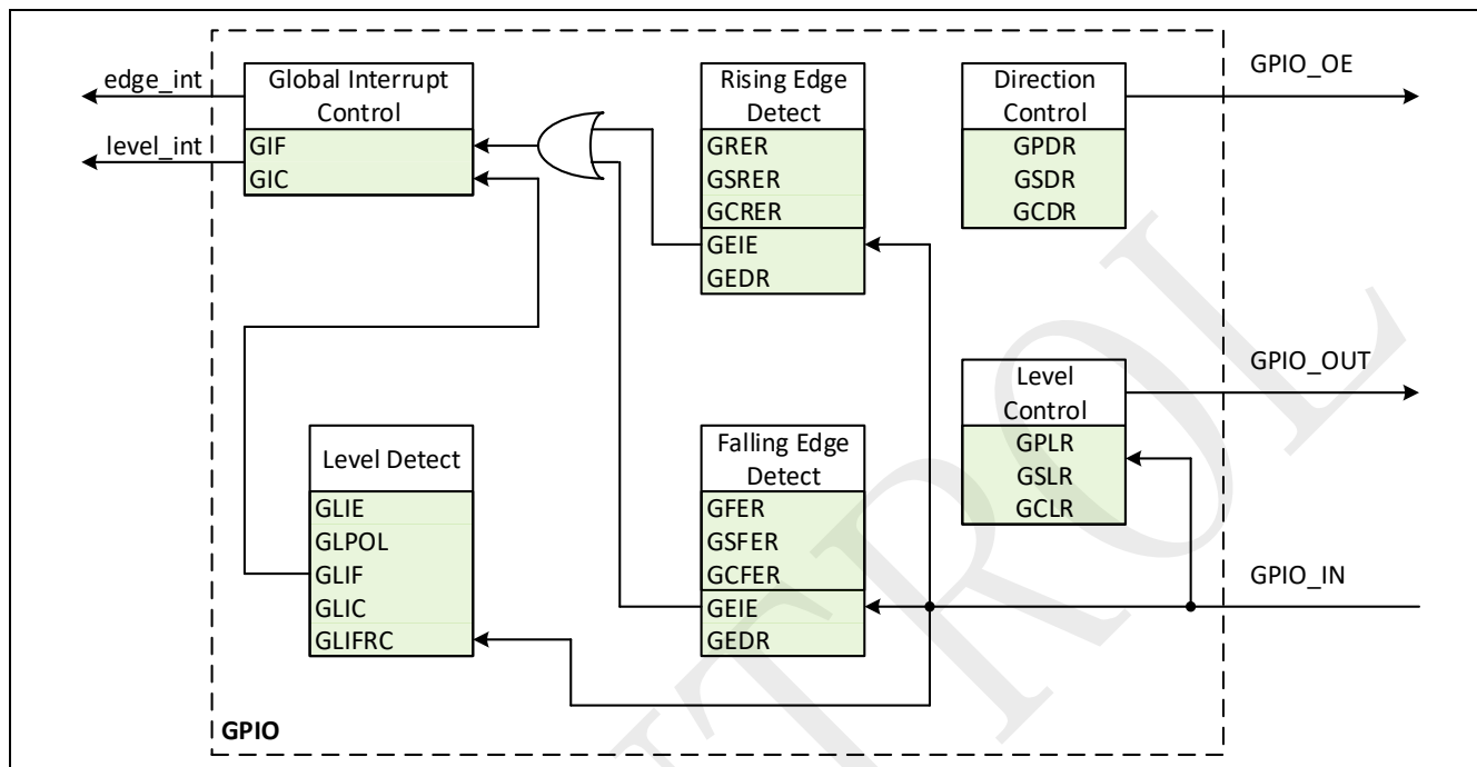
图 4-5: GPIO 结构框图
