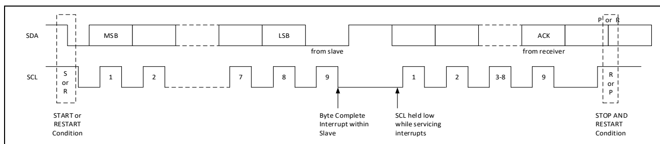
图 18-1: I2C 总线数据传输
