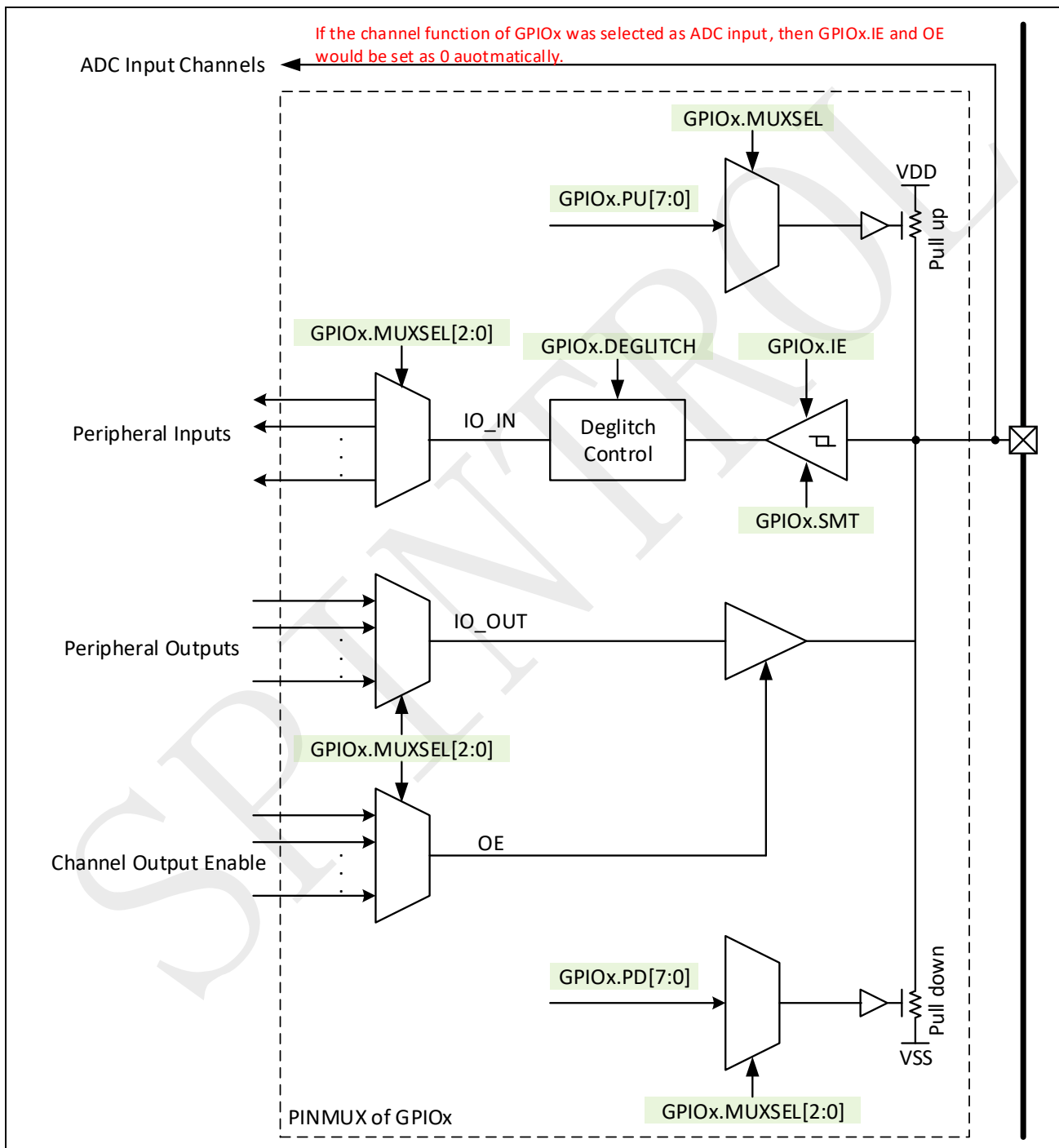
图 4-2: PINMUX 结构框图
