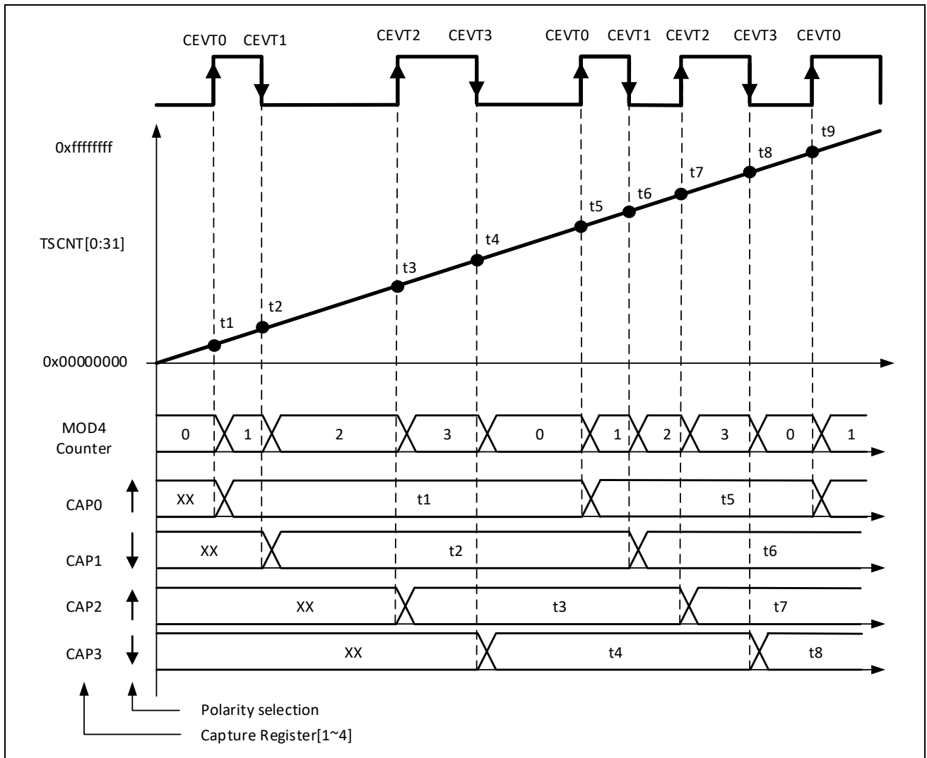
图 11-12：通过绝对时间戳捕获计算周期和占空
