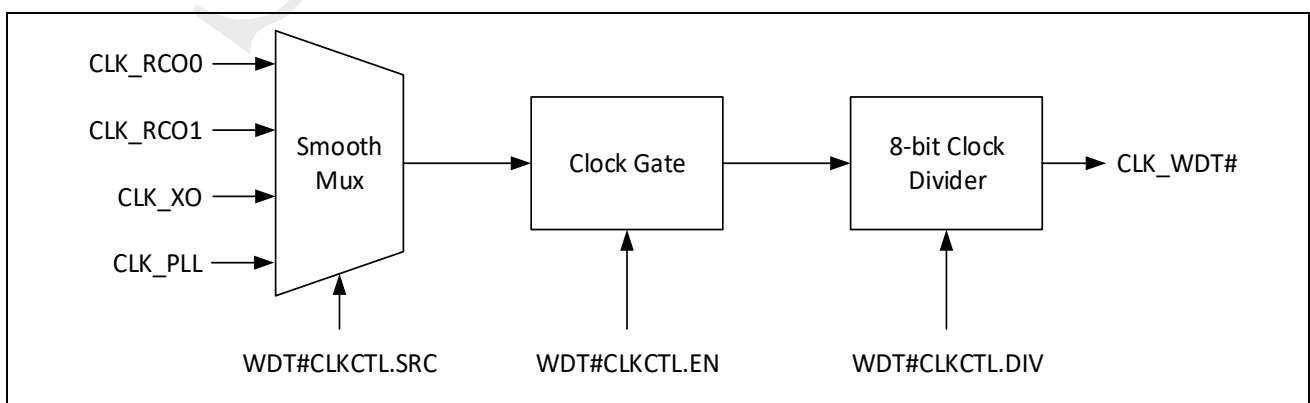
图 3-12：WDT 时钟控制框图
