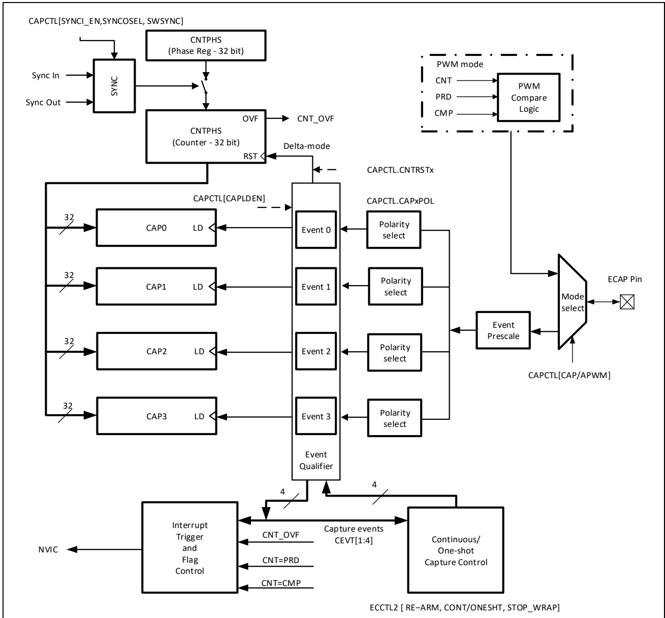
图 11-3: 捕获模式功能框图
