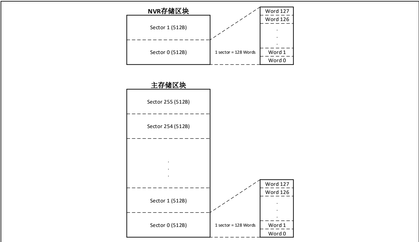
图 20-2: Flash 模块逻辑结构
