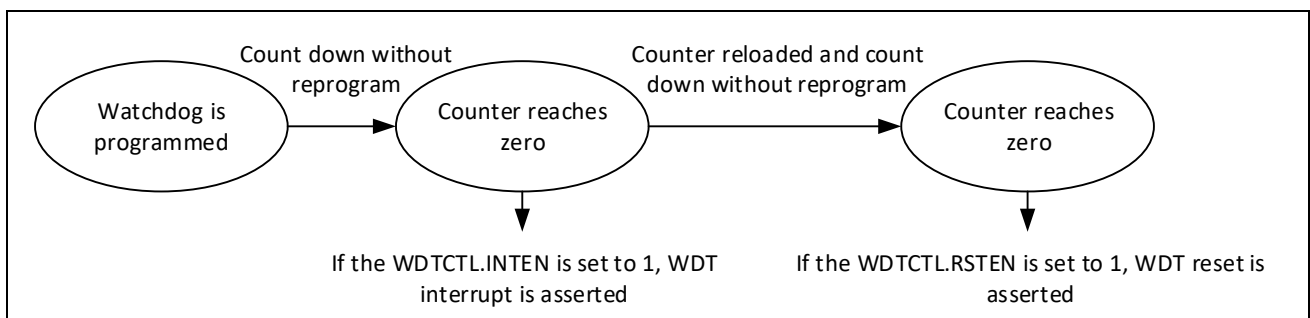
图 9-1：看门狗工作流程
