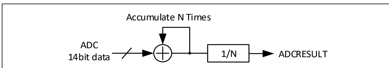
图 12-5: ADC 转换结果的平均化处理
