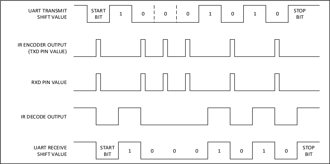
图 17-4：IR 发送和接收示例
