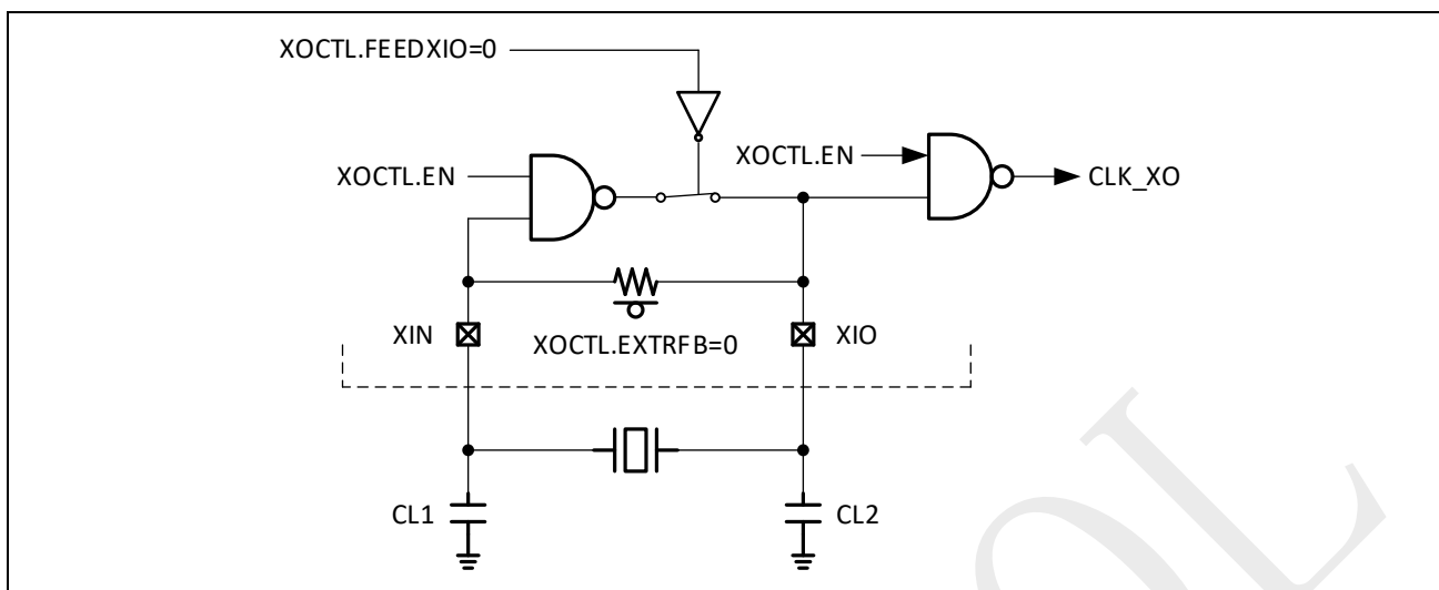
图 3-4：内部晶振模式
