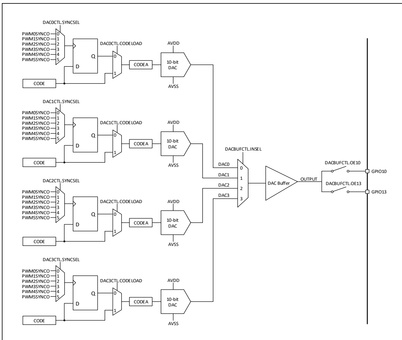
图 16-1: DAC 和 DAC Buffer 框图
