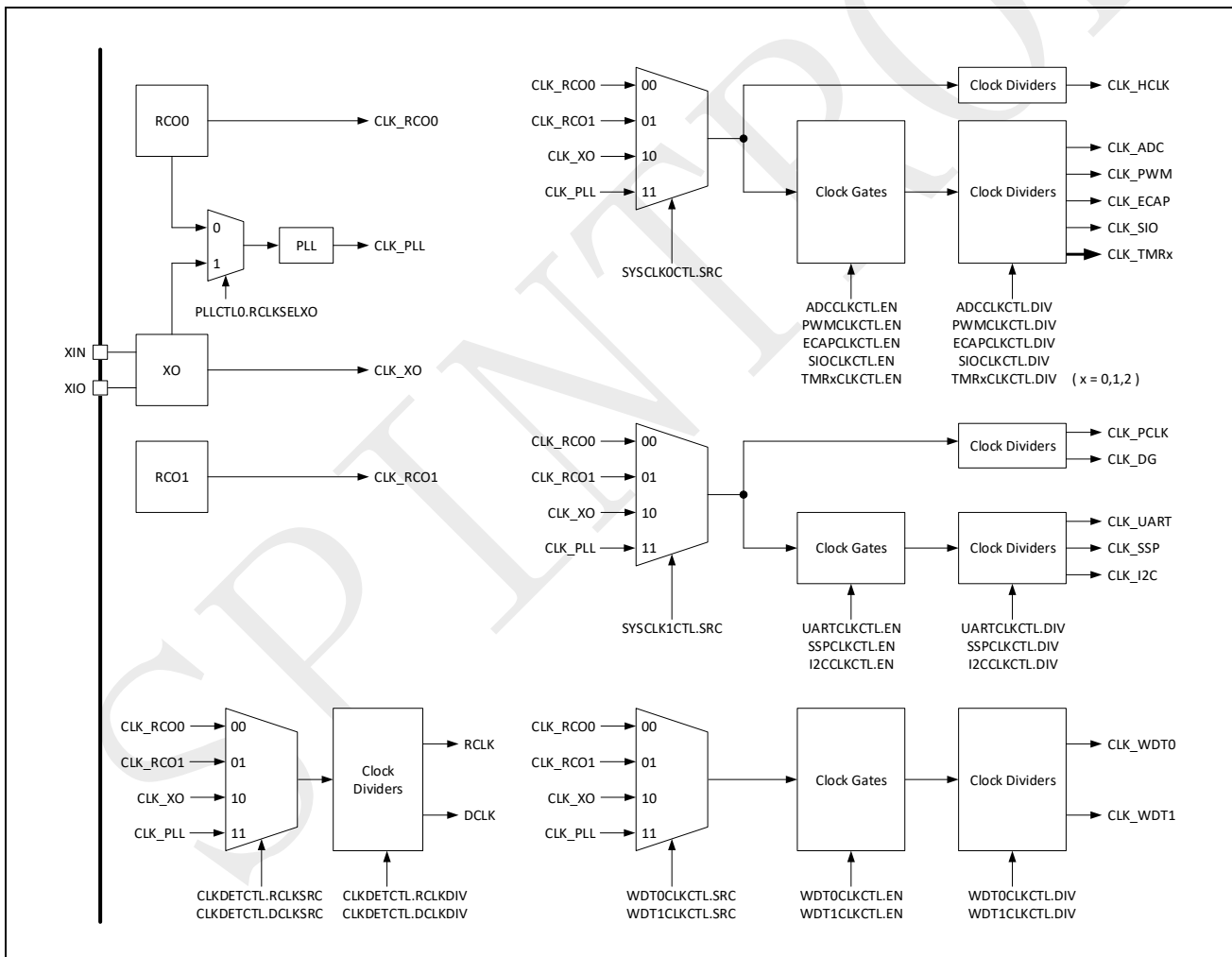
图 1-2：SPC1168 时钟树
