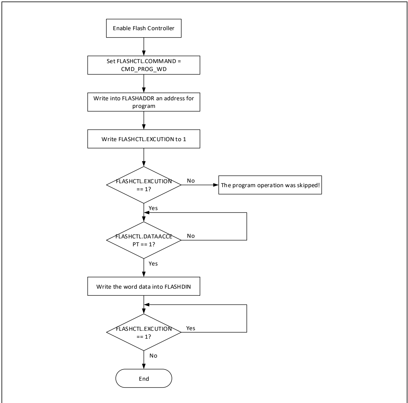
图 20-4: Flash 存储器编程操作流程
