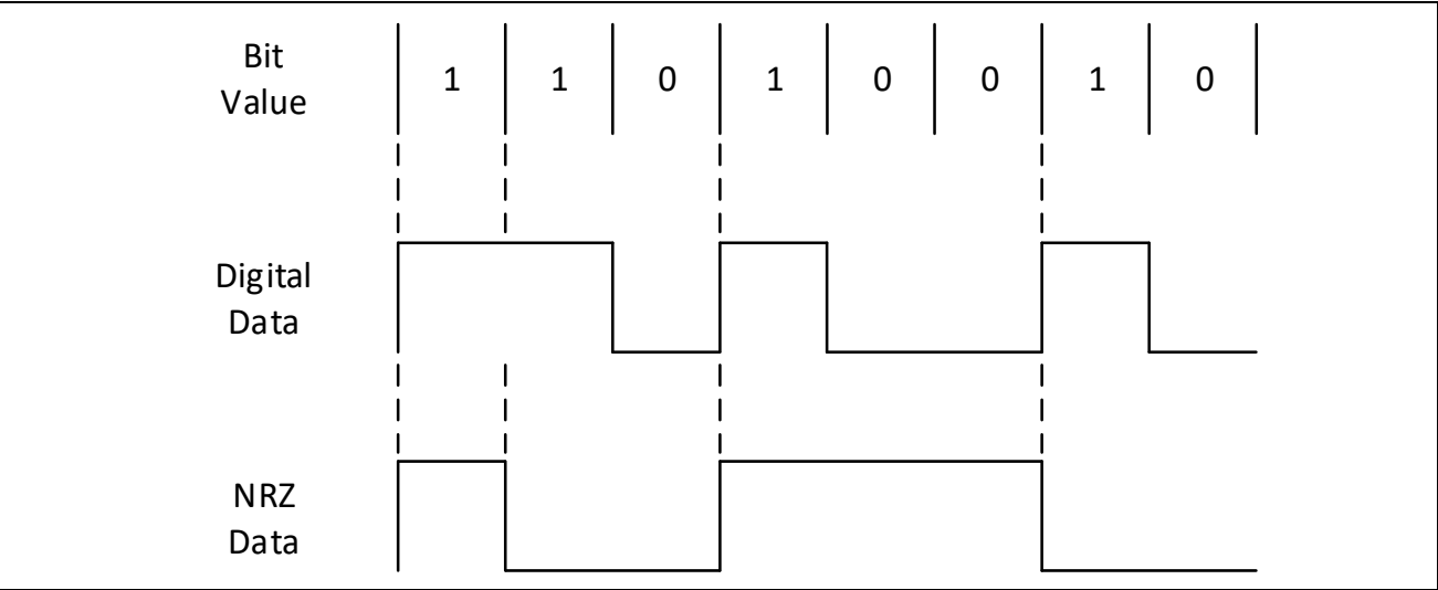
图 17-3: NRZ 编码示例 – 0b0100_1011
