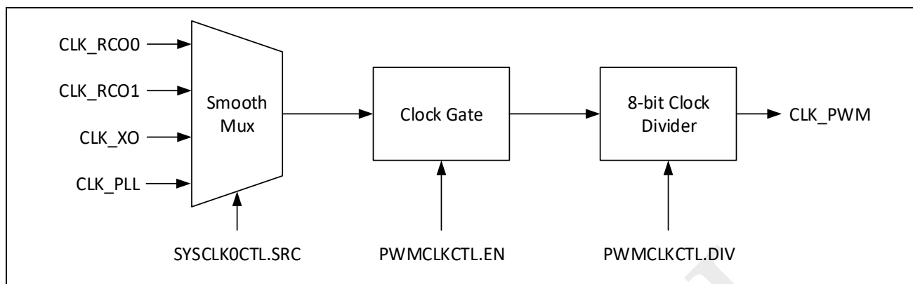
图 3-15: PWM 时钟控制框图
