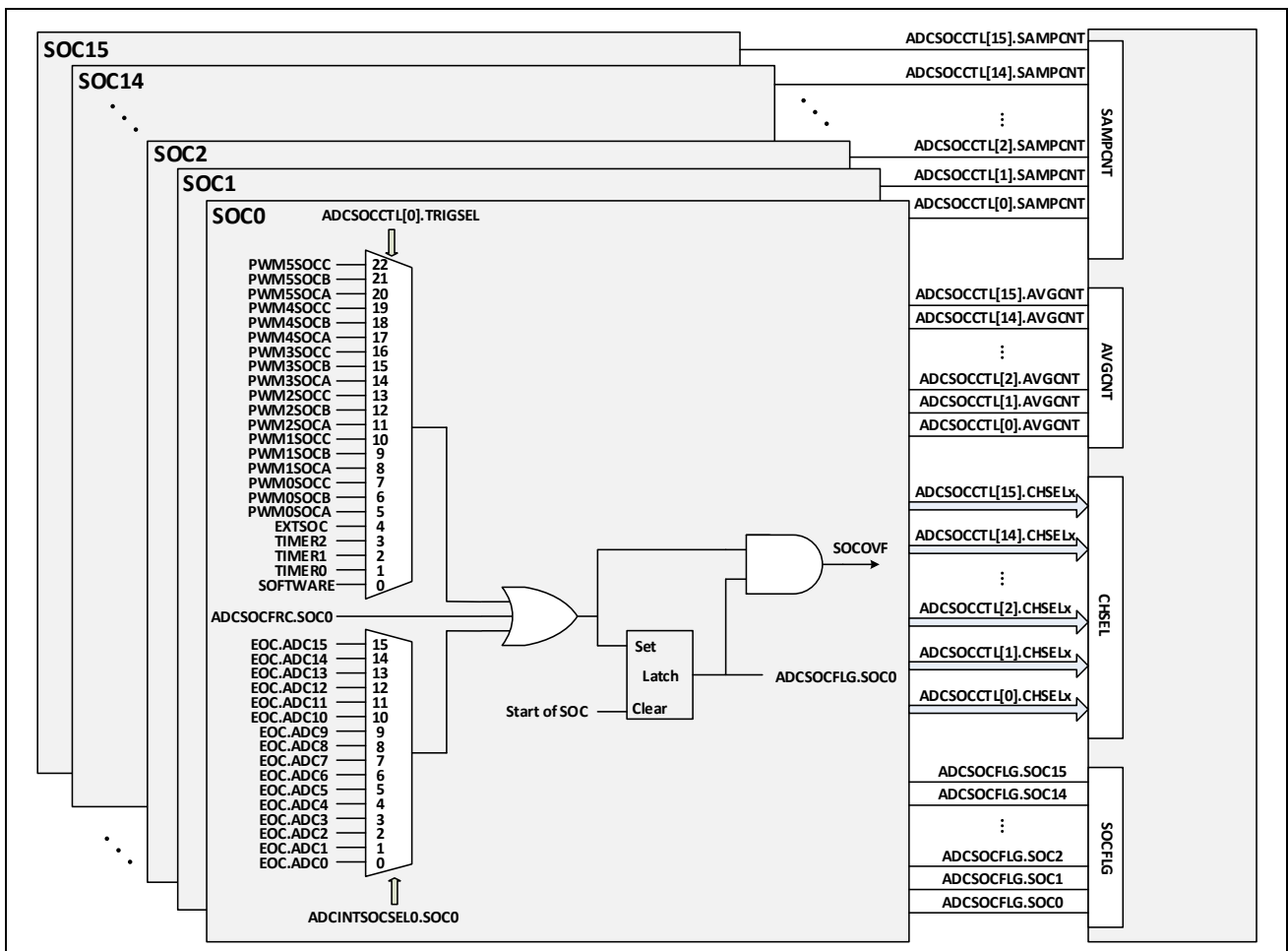
图 12-2: SOC 配置框图
