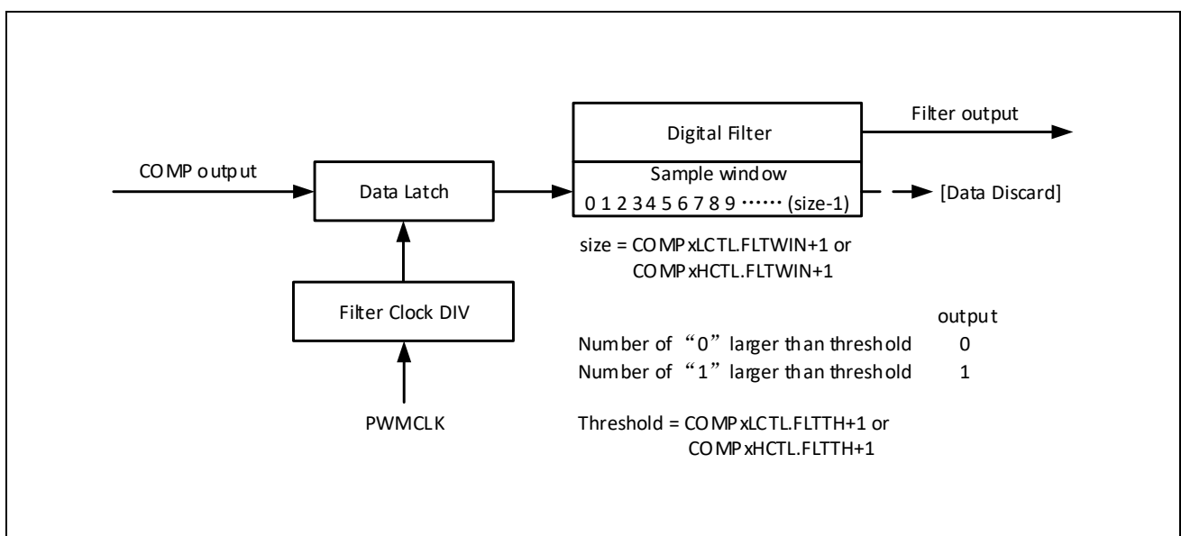
图 15-2: 数字滤波器行为描述
