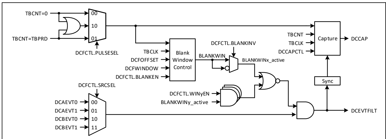
图 10-17: 事件过滤逻辑
