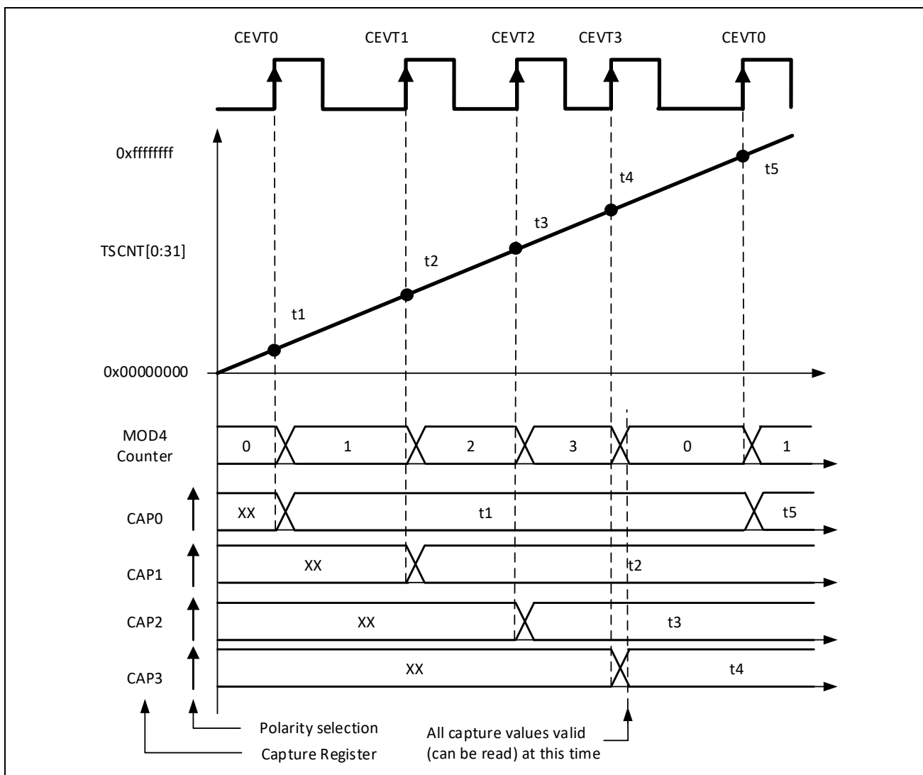
图 11-11：上升沿检测和绝对时间戳捕获
