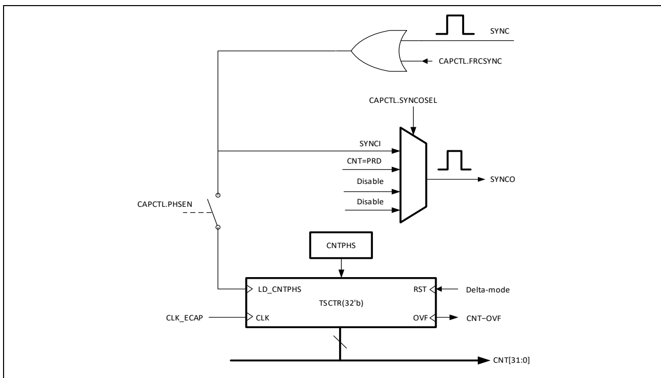
图 11-7：时间戳计数器及其同步
