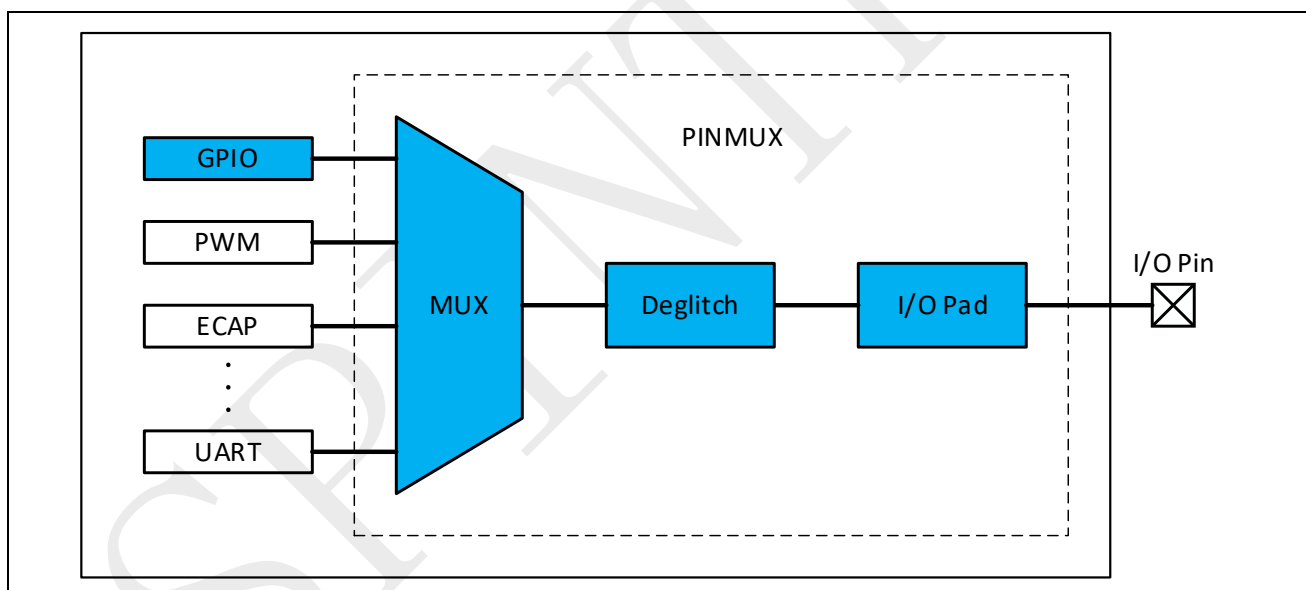
图 4-1：I/O 控制结构框图
