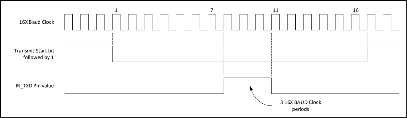
图 17-5：零值比特位的脉冲
