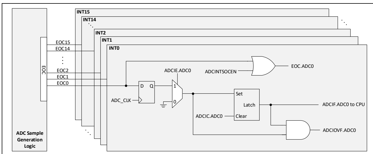
图 12-10: ADC 中断结构框图
