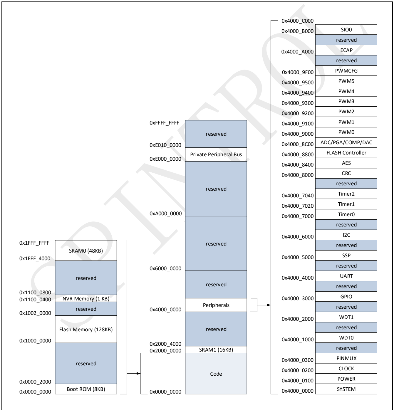
图 1-3：SPC1168 存储空间地址映射
