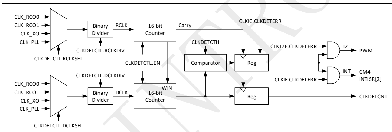
图 3-18：时钟交叉检测
