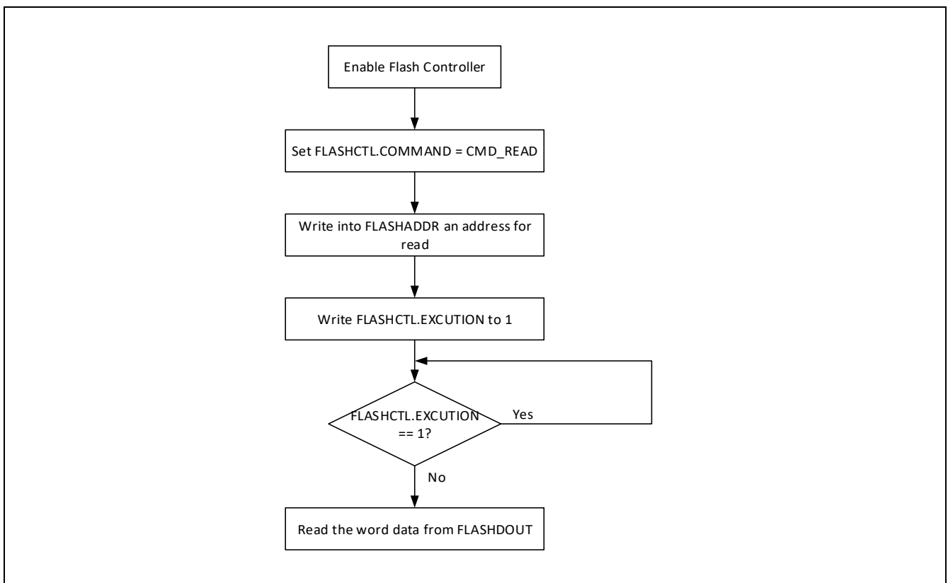
图 20-3: Flash 存储器读操作流程
