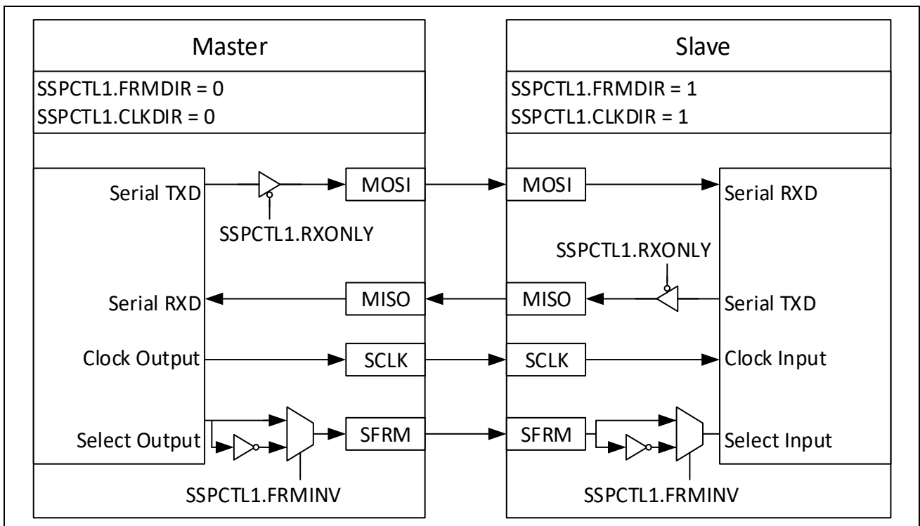
图 19-2: SSP 主机-从机连接示意图
