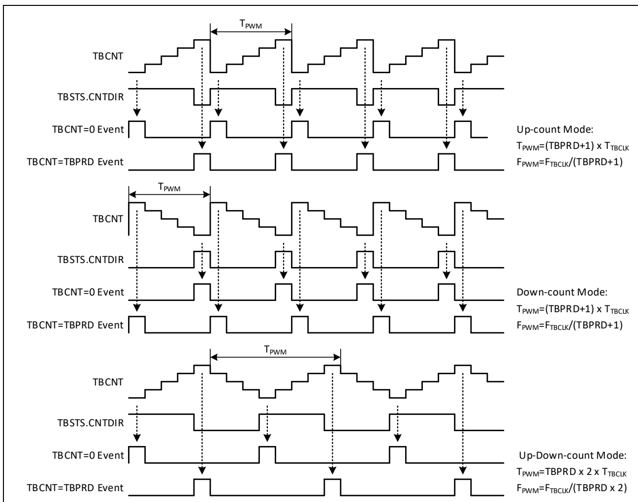
图 10-4：时基计数波形
