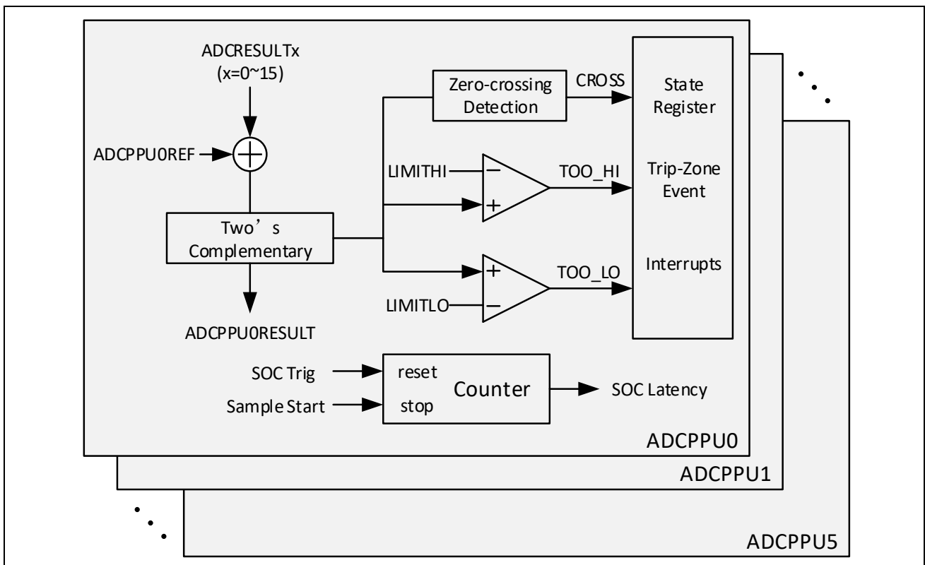
图 12-11：后处理单元构架
