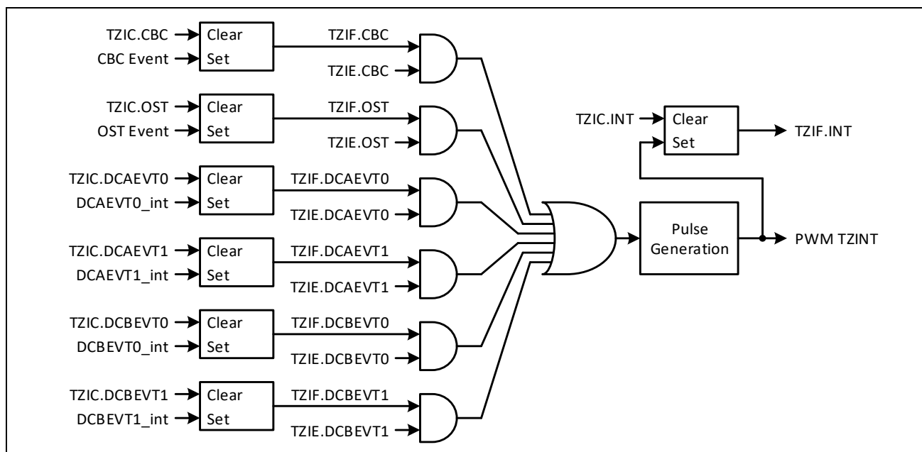
图 10-15: 信号封锁中断产生
