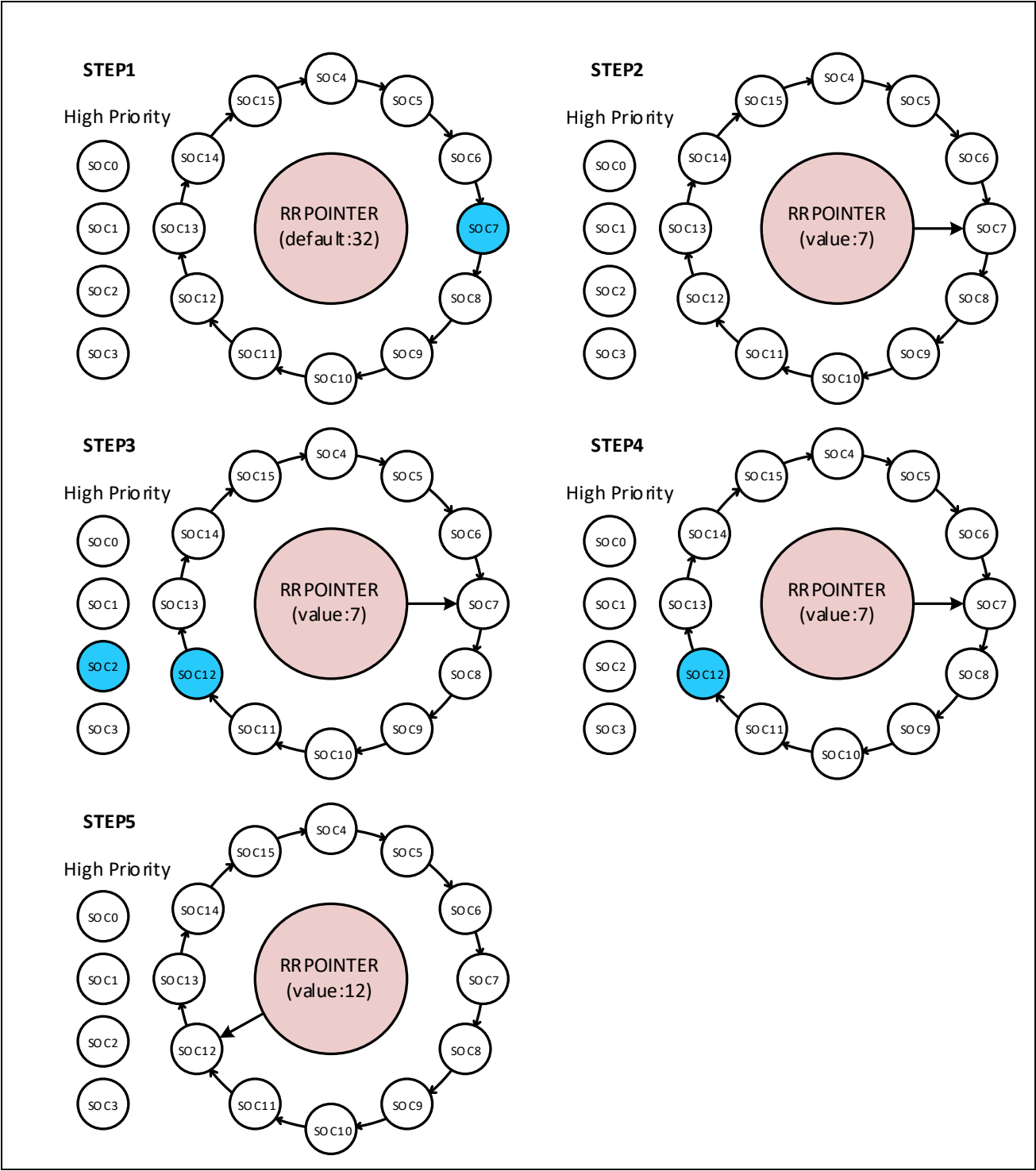
图 12-8：高优先级示例
