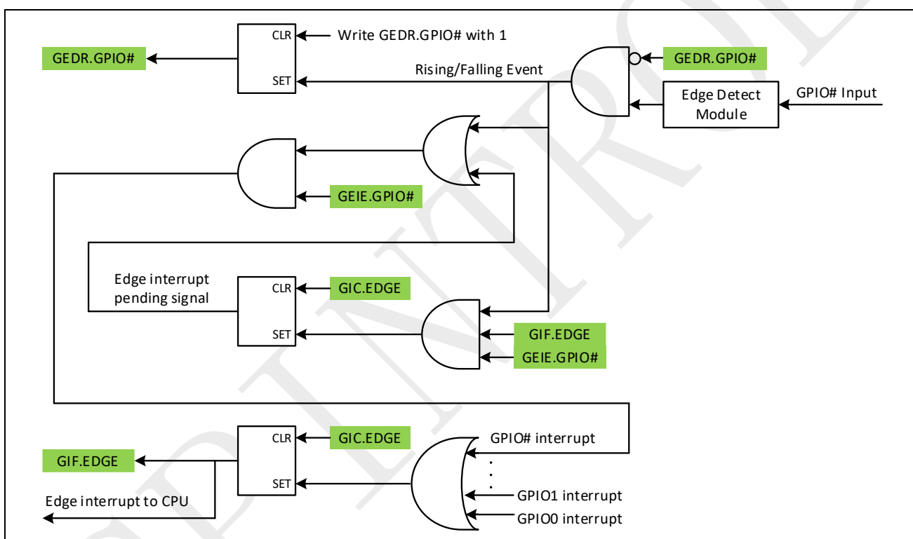
图 4-6: GPIO 边沿触发中断
