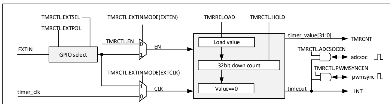
图 8-1：通用定时器结构
