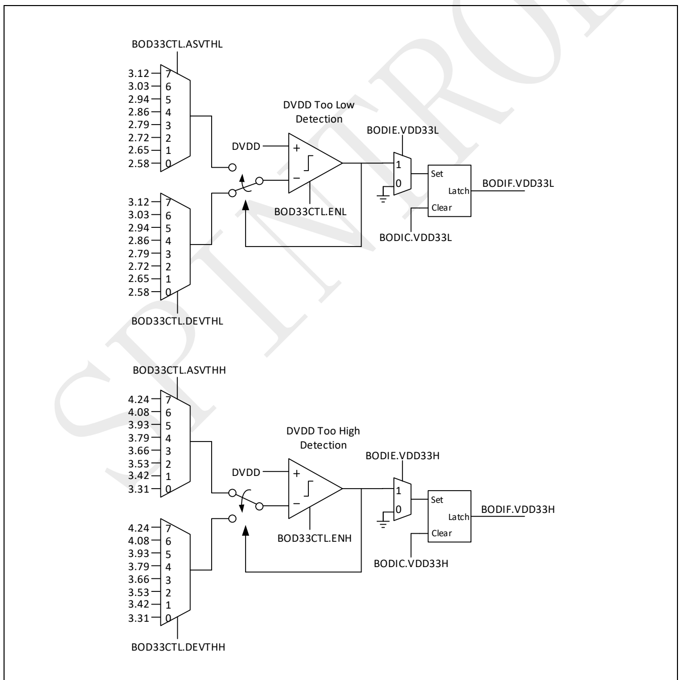
图 2-2: 3.3V 额定电压域检测电路框图
