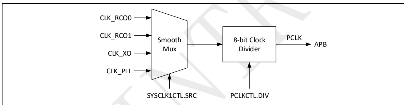
图 3-9: PCLK 控制框图
