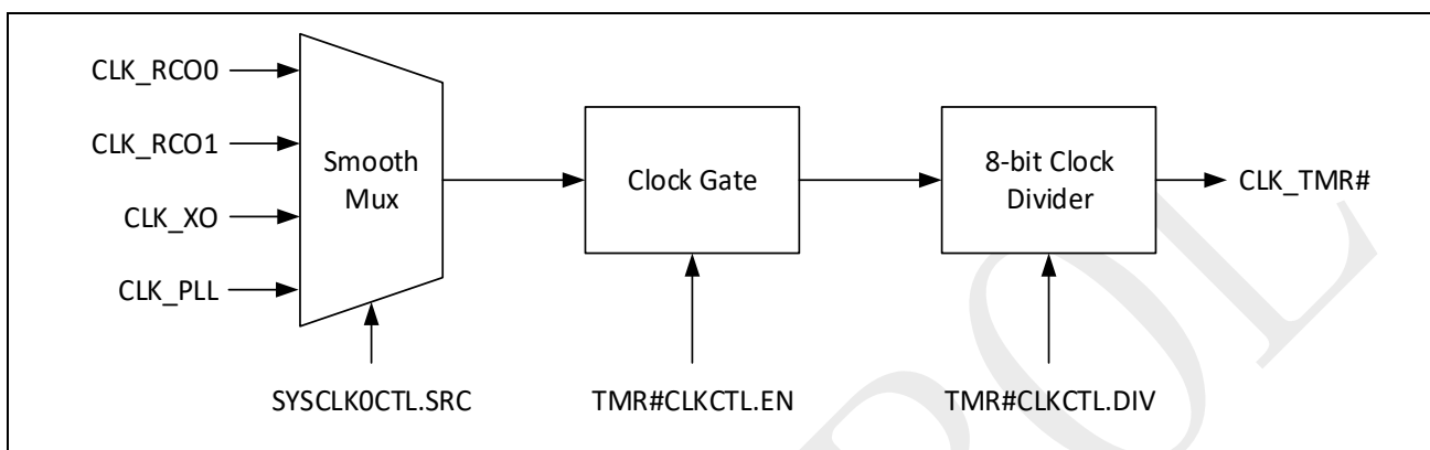
图 3-13：通用定时器时钟控制框图
