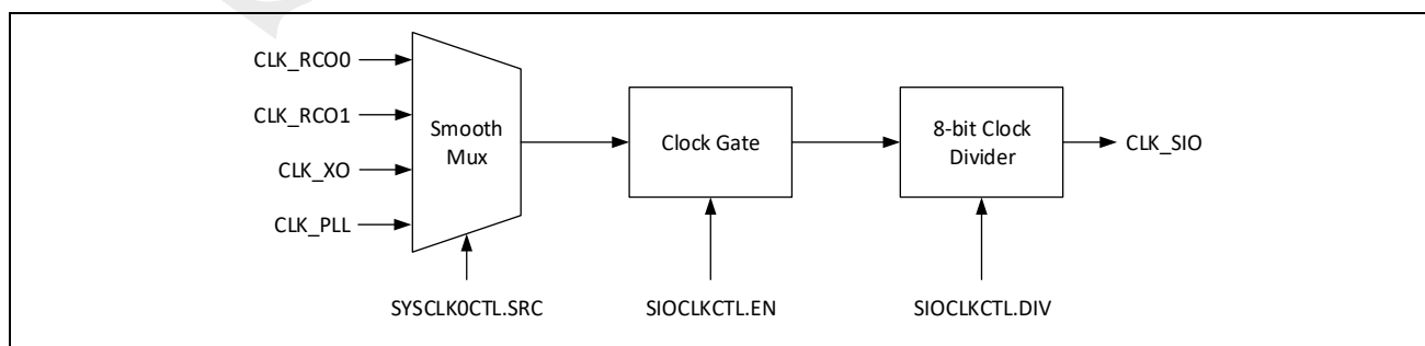
图 3-17: SIO 时钟控制框图
