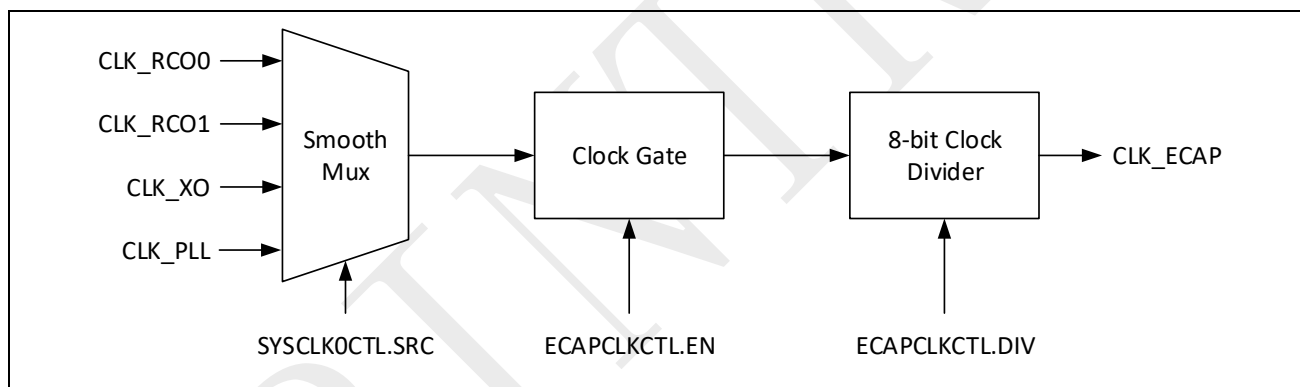
图 3-16: ECAP 时钟控制框图
