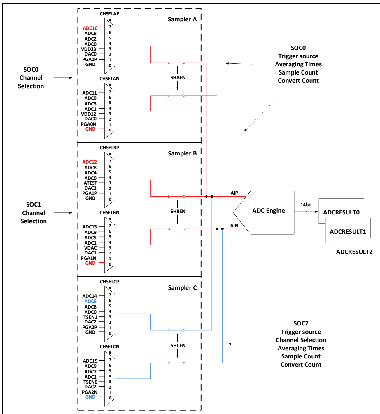
图 12-9: SOC0 同时采样的信号流和配置说明
