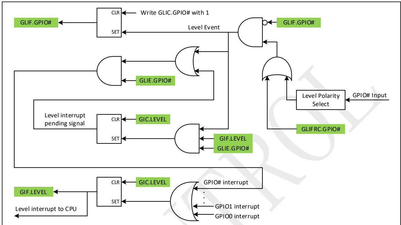
图 4-7：GPIO 电平触发中断
