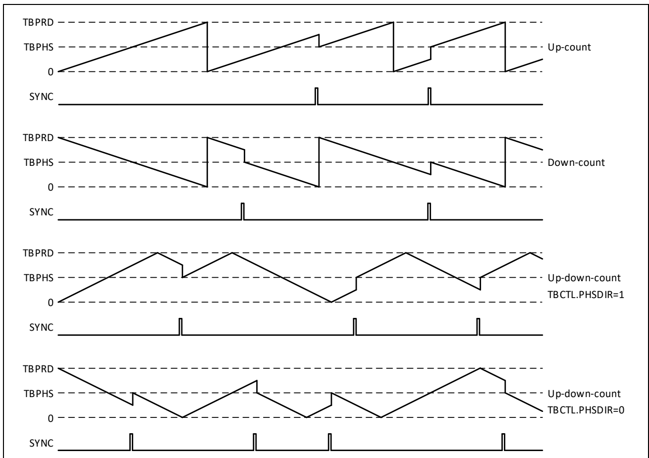
图 10-5：时基相位同步波形
