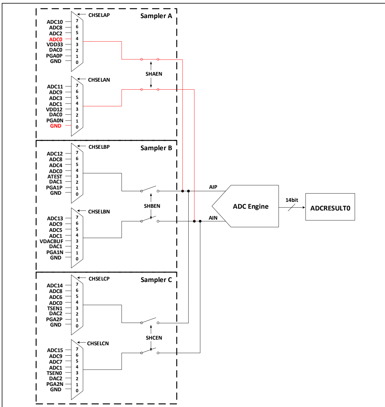
图 12-3: 示例 12.3.1 的 ADC 通道选择
