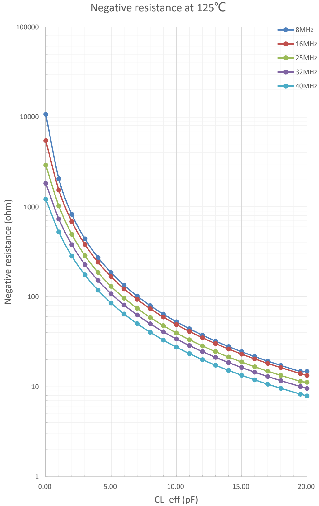
图 5-7：内部晶振负阻值（125℃）
