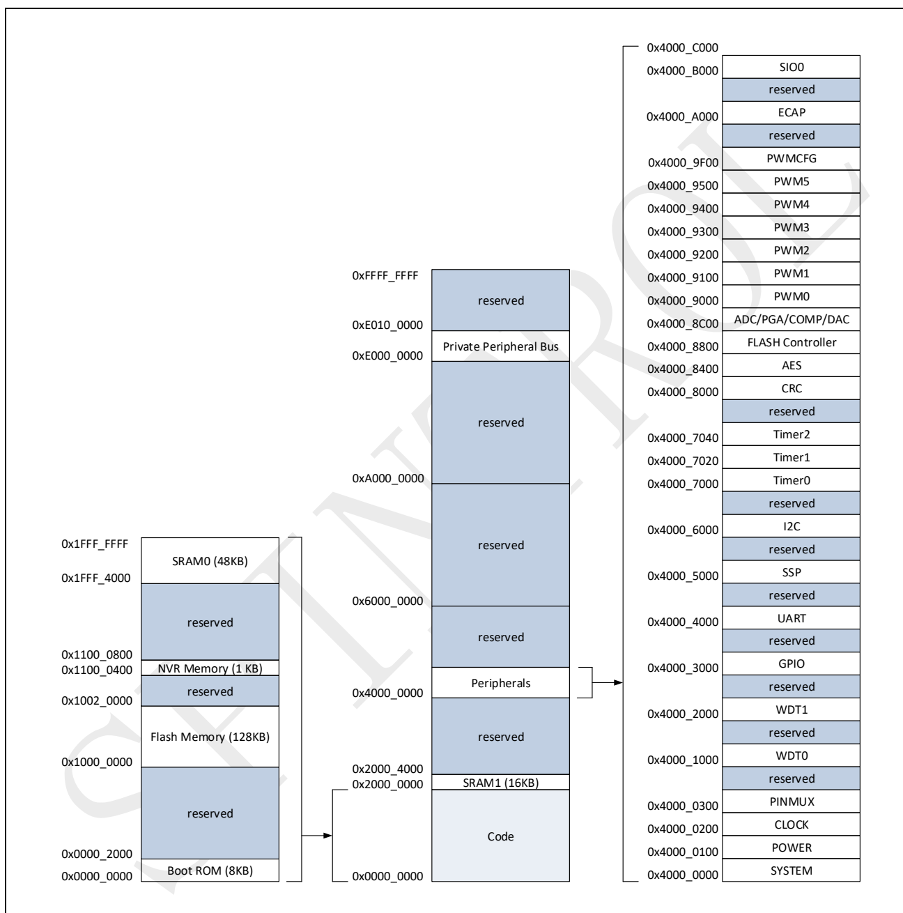
图 4-1: 存储器映射
