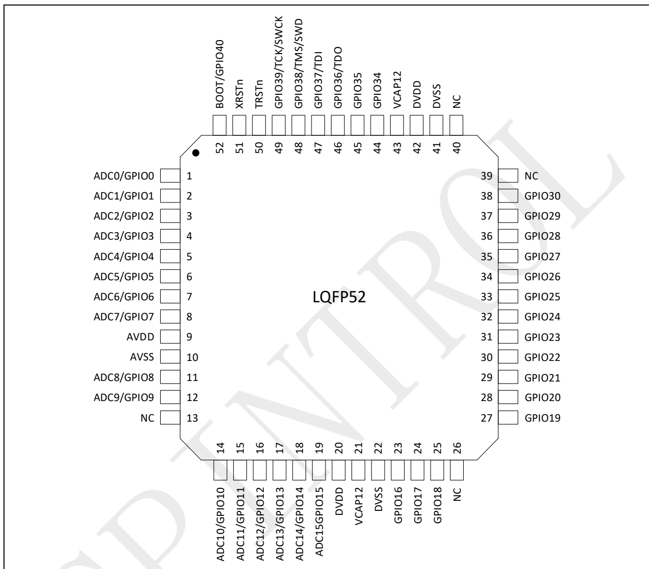
图 3-2: SPC1168 LQFP52 引脚排列
