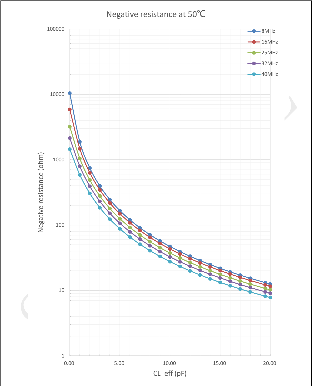
图 5-4：内部晶振负阻值（50℃）
