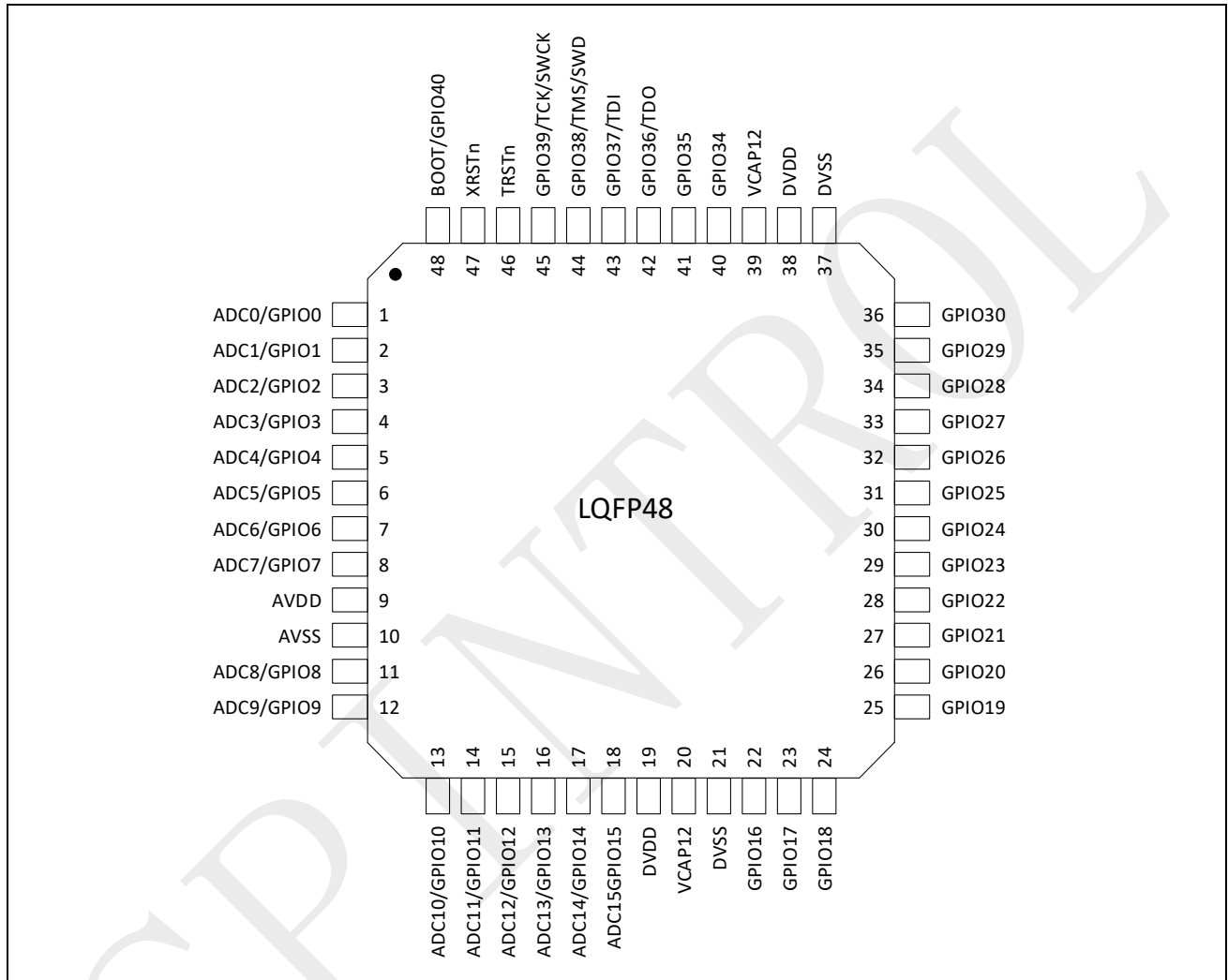
图 3-1: SPC1168 LQFP48 引脚排列
