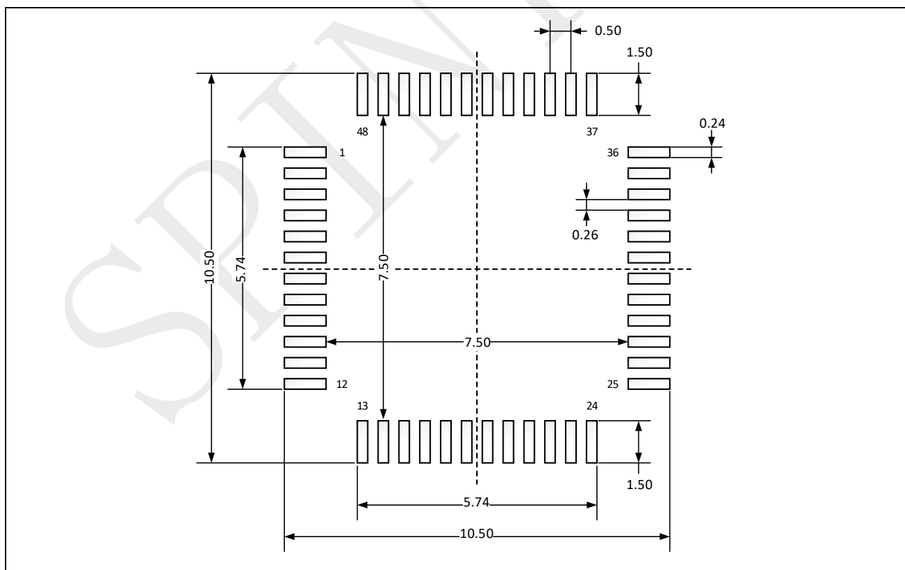
图 6-2: LQFP48-48 脚, 7 x 7 mm 薄型正方扁平封装建议尺寸
