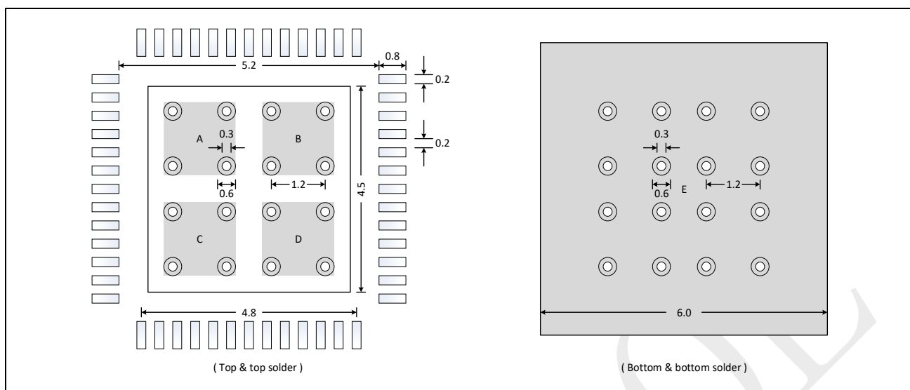
图 6-10: QFN52-52 脚, 6 x 6 mm 方形扁平无引脚封装推荐尺寸
