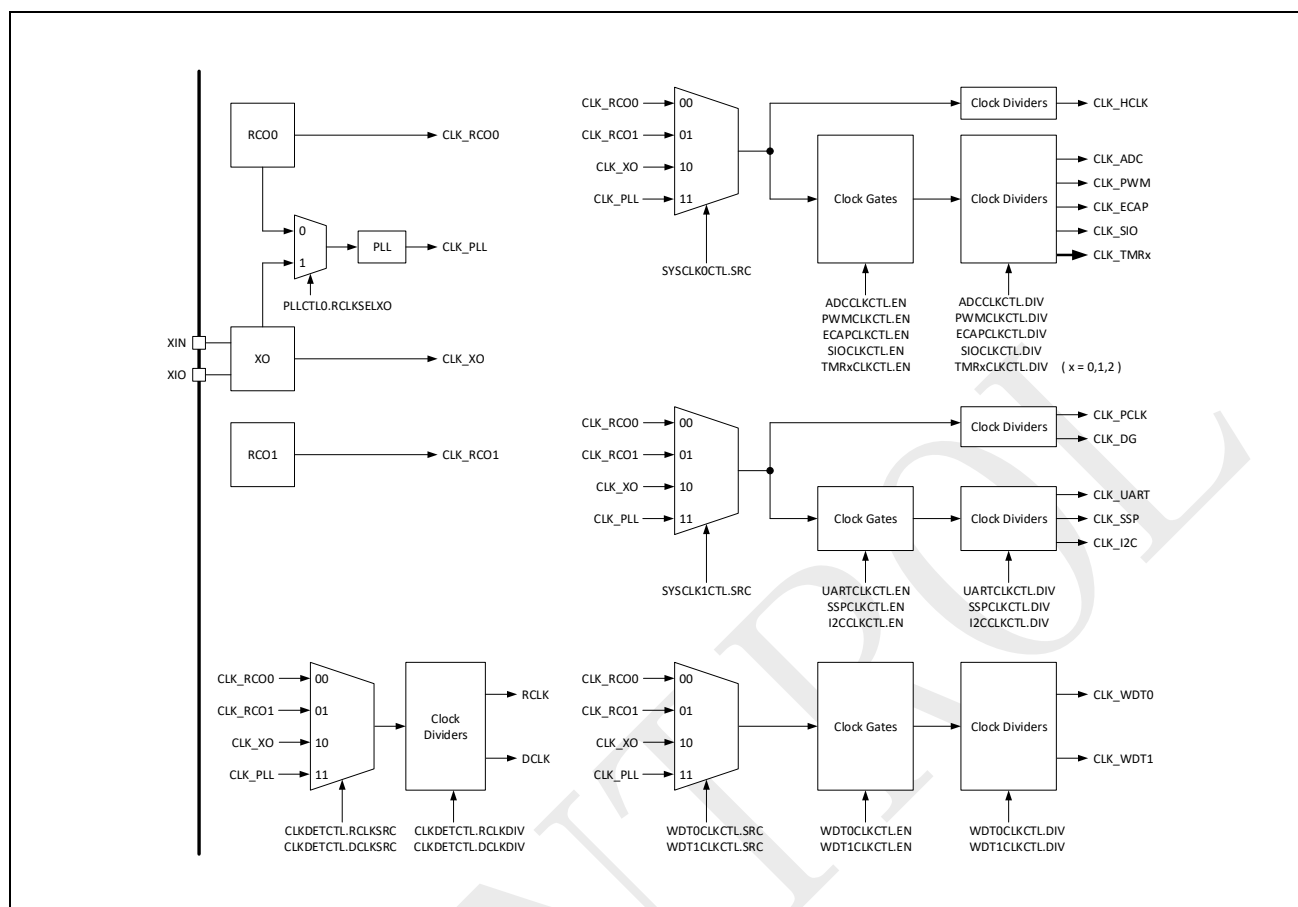
图 1-2: 时钟树
