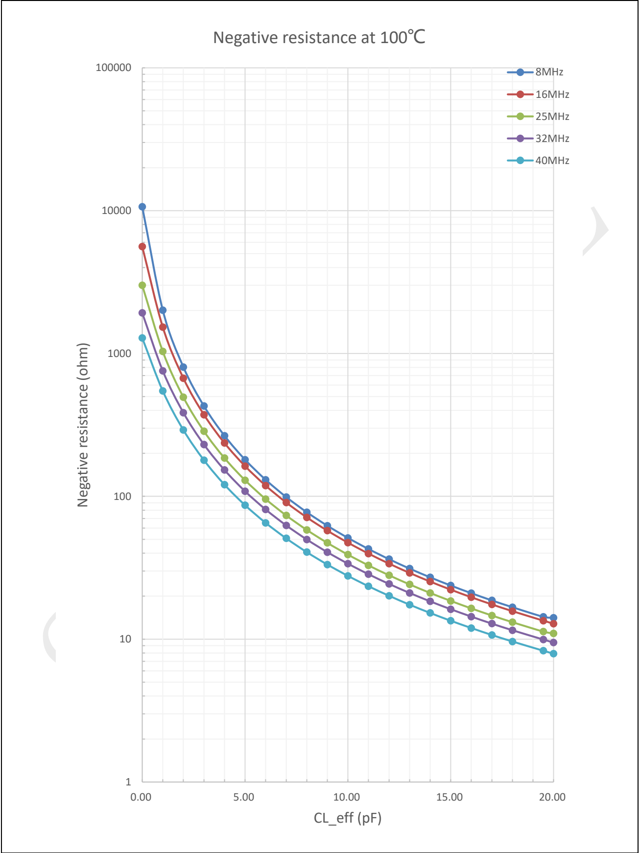
图 5-6：内部晶振负阻值（100℃）
