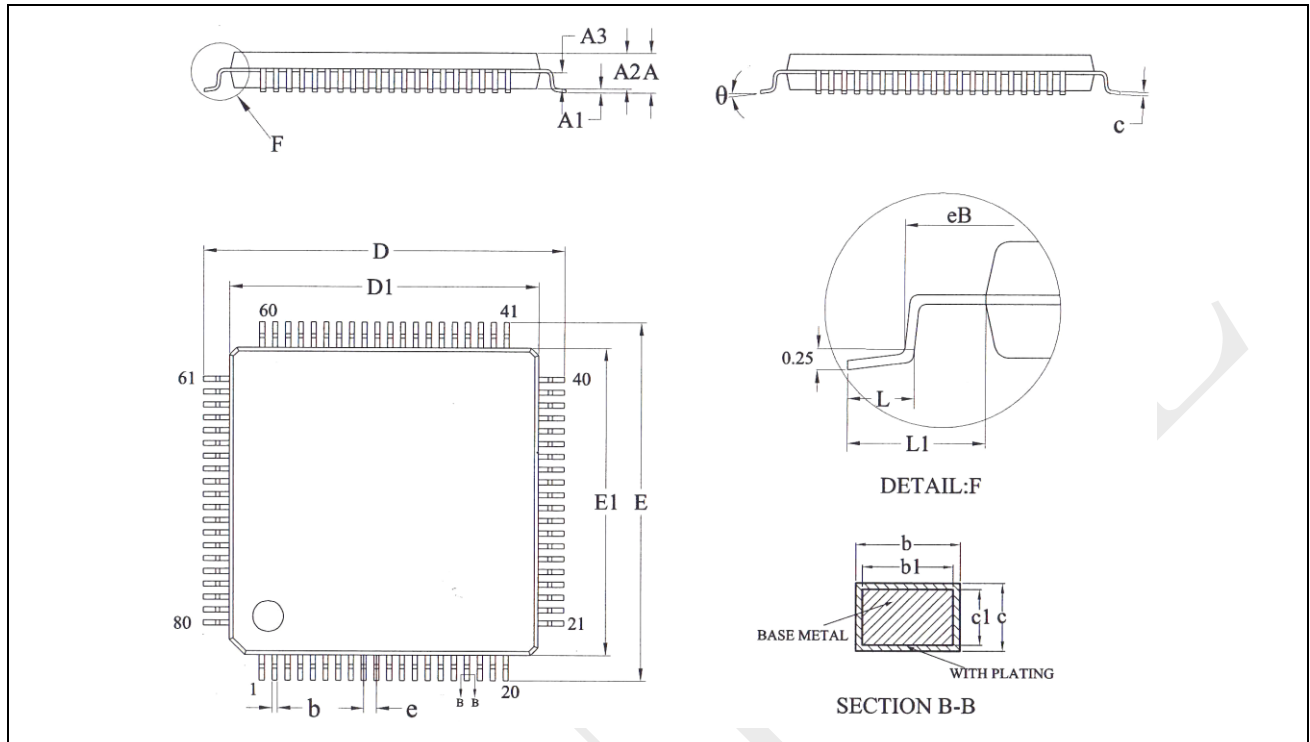
图 6-5: LQFP64 – 64 脚, 10 x 10 mm 薄型正方扁平封装图
