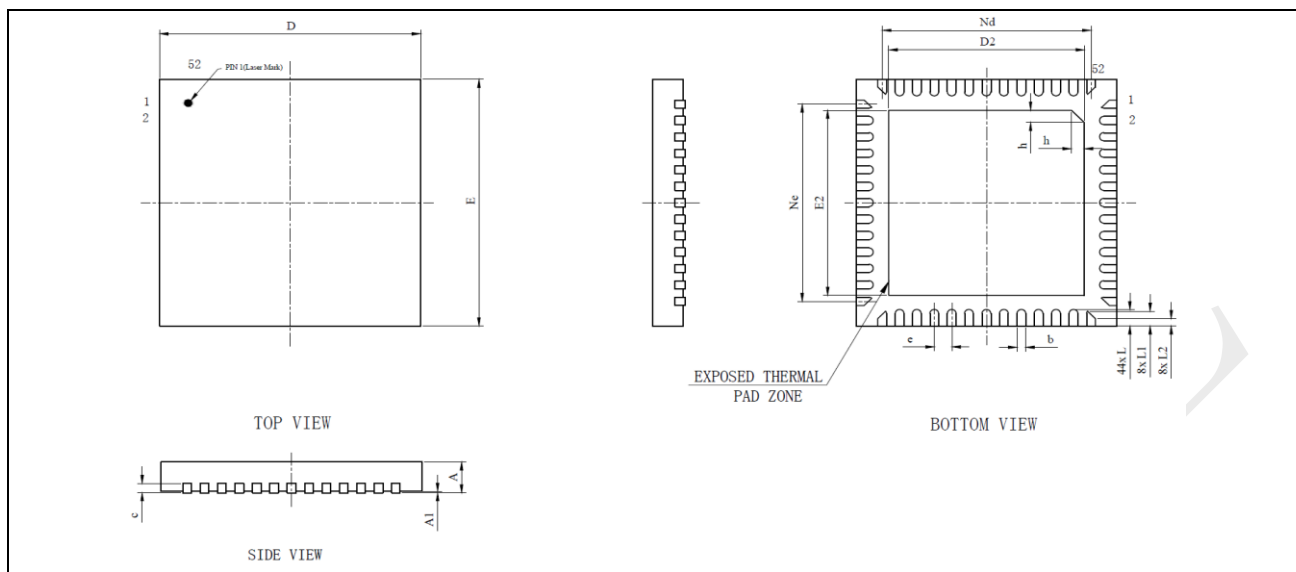
图 6-9: QFN52-52 脚, 6 x 6 mm 方形扁平无引脚封装
