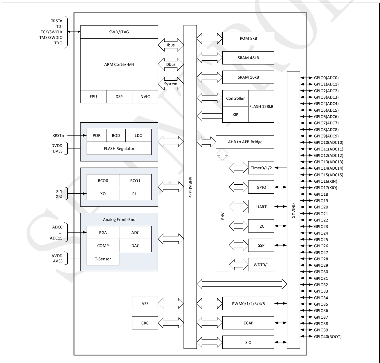
图 1-1: SPC1168 功能框图
