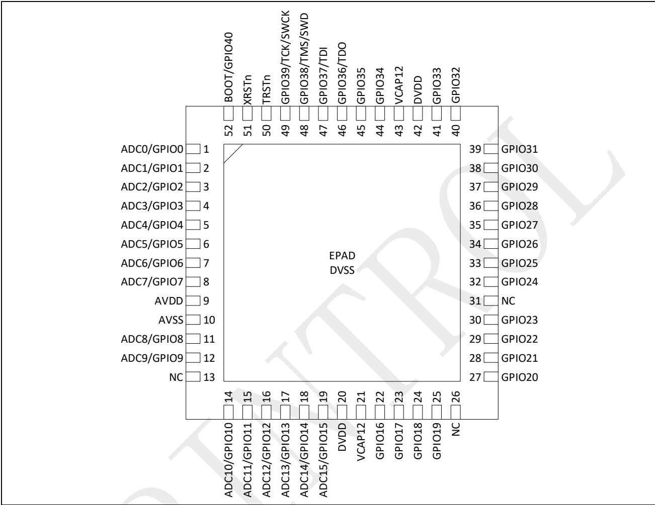
图 3-5：SPC1168 QFN52 引脚排列
