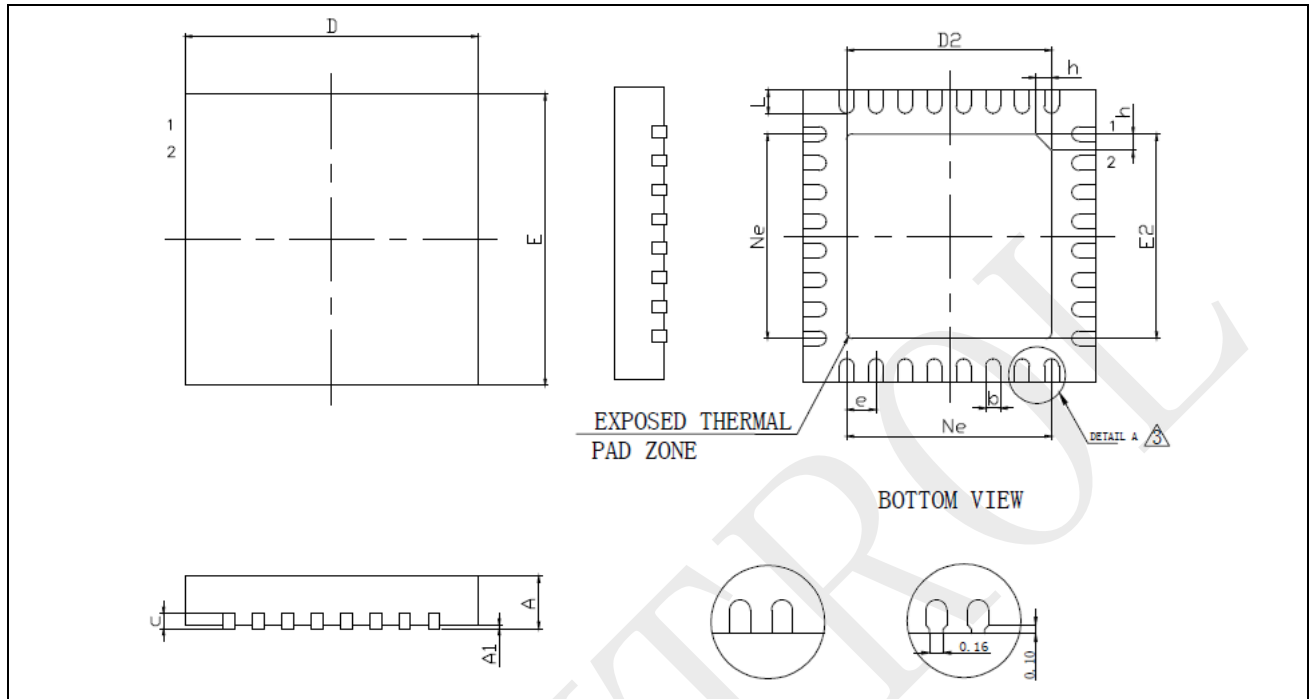
图 6-7: QFN32–32 脚, 5 x 5 mm 方形扁平无引脚封装
