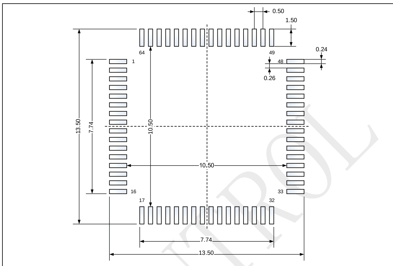
图 6-6: LQFP64 - 64 脚, 10 x 10 mm 薄型正方扁平封装建议焊垫尺寸
