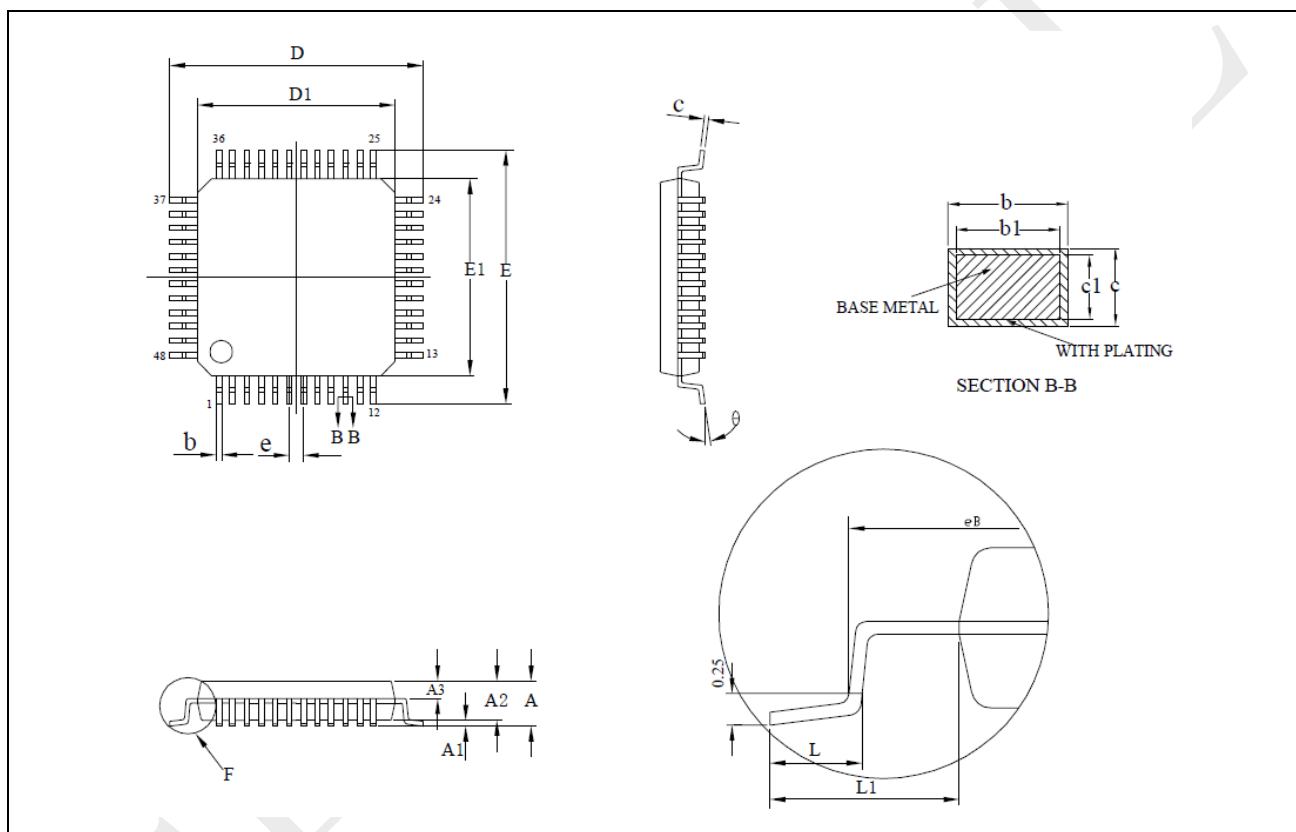
图 6-1: LQFP48-48 脚, 7 x 7 mm 薄型正方扁平封装图
