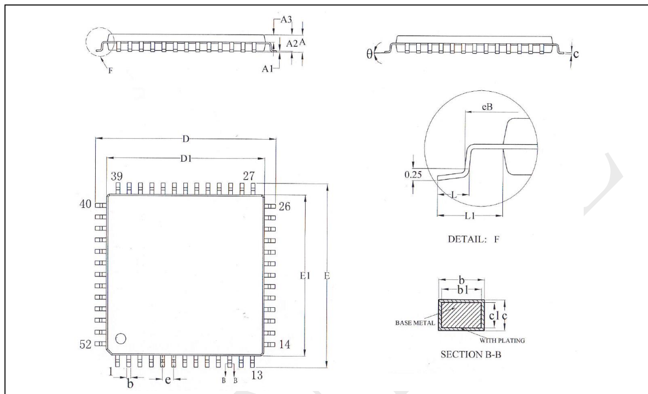
图 6-3: LQFP52-52 脚, 14 x 14 mm 薄型正方扁平封装图
