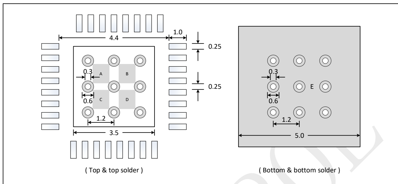
图 6-8: QFN32-32 脚, 5 x 5 mm 方形扁平无引脚封装推荐尺寸
