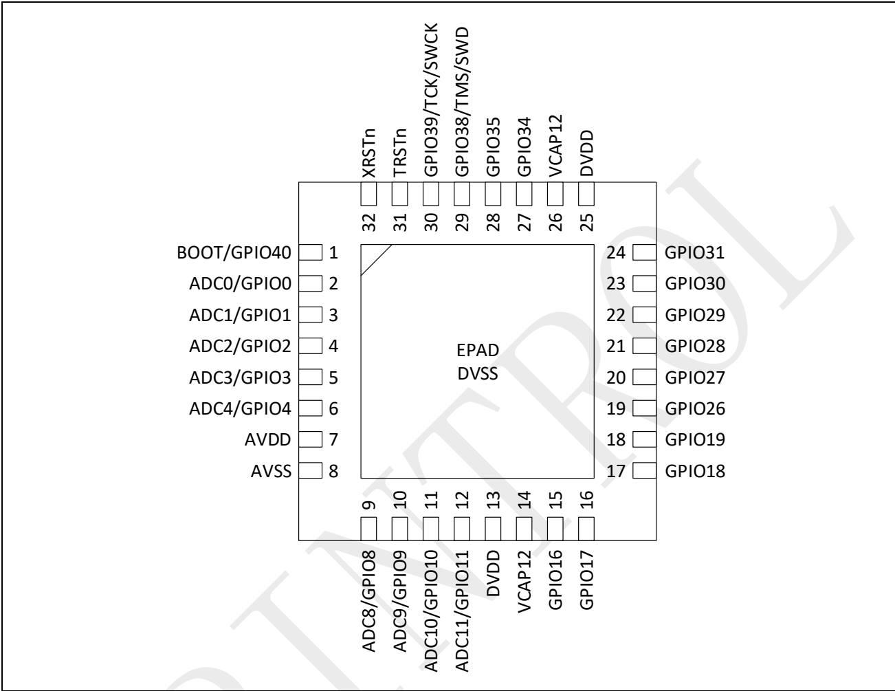
图 3-4： SPC1168 QFN32 引脚排列
