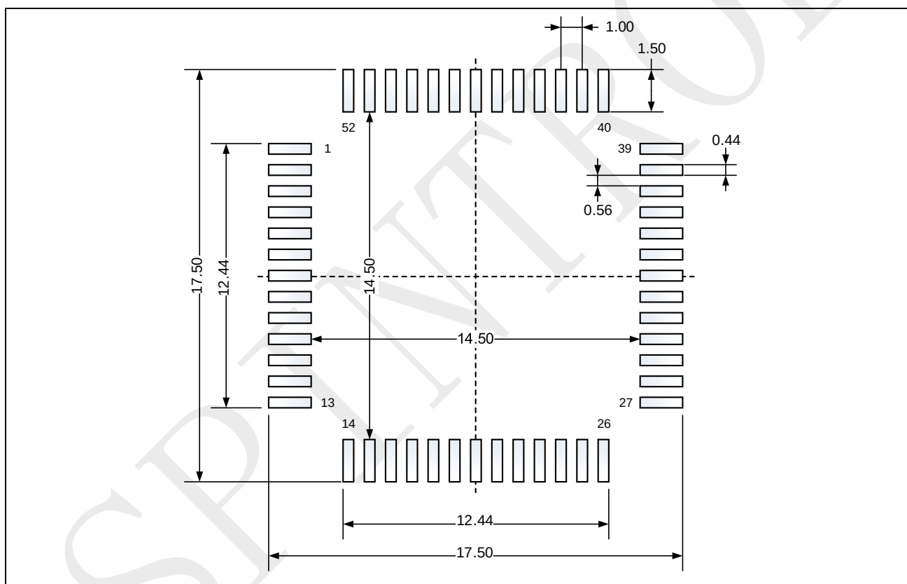
图 6-4: LQFP52-52 脚, 14 x 14 mm 薄型正方扁平封装建议尺寸
