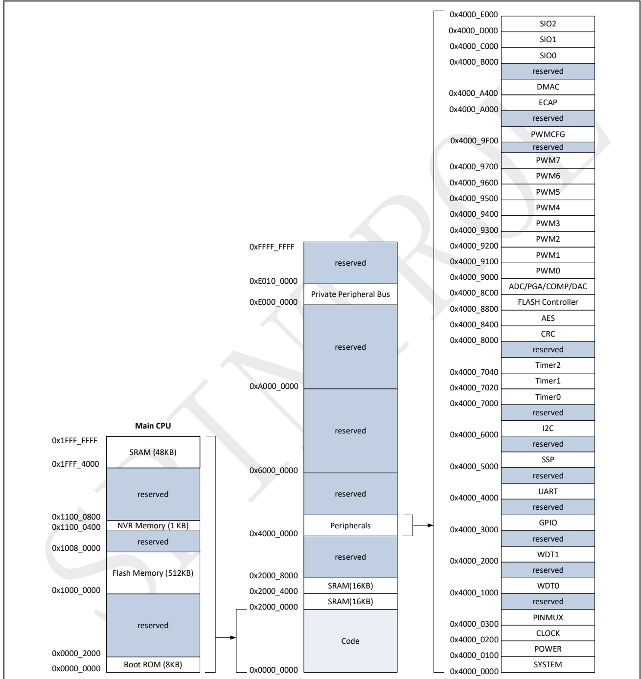
图 4-1: SPC2168 在 Cache 禁用且 CAU 停用下的存储器映射（单核模式）
