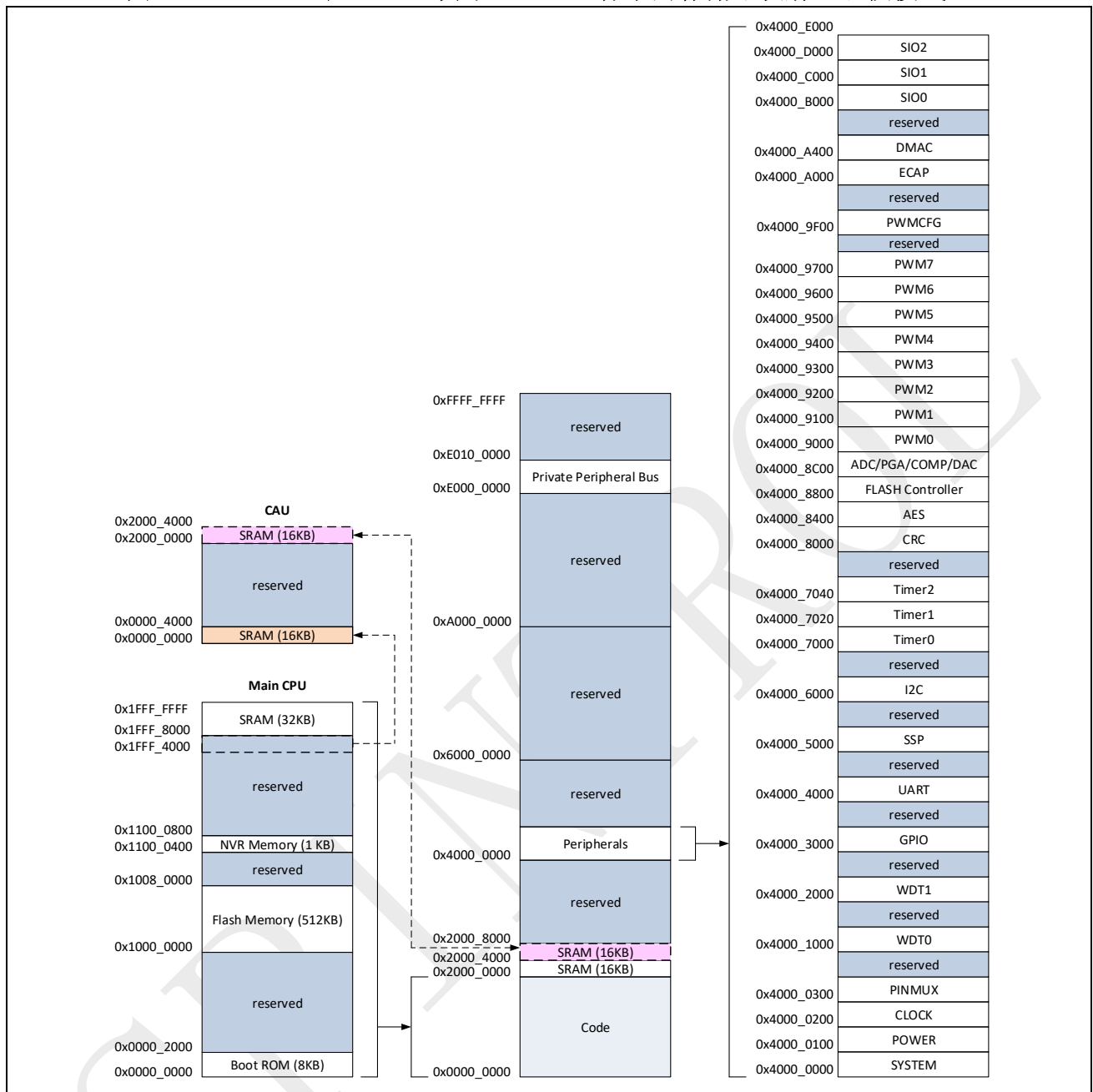
图 4-3: SPC2168 在 Cache 禁用且 CAU 运行下的存储器映射（双核模式）
