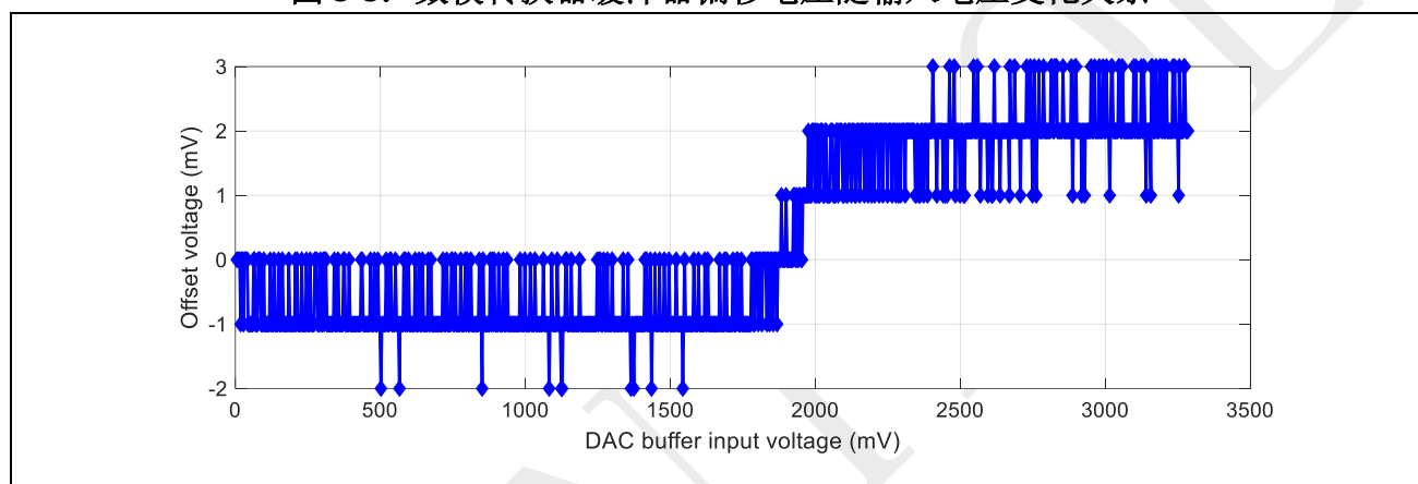
图 5-8: 数模转换器缓冲器偏移电压随输入电压变化关系
