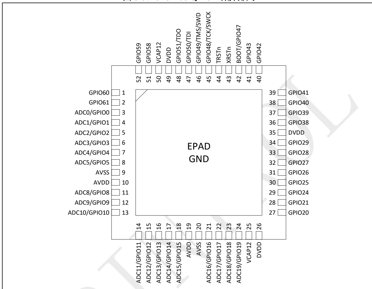
图 3-5: SPC2168 QFN52 引脚排列
