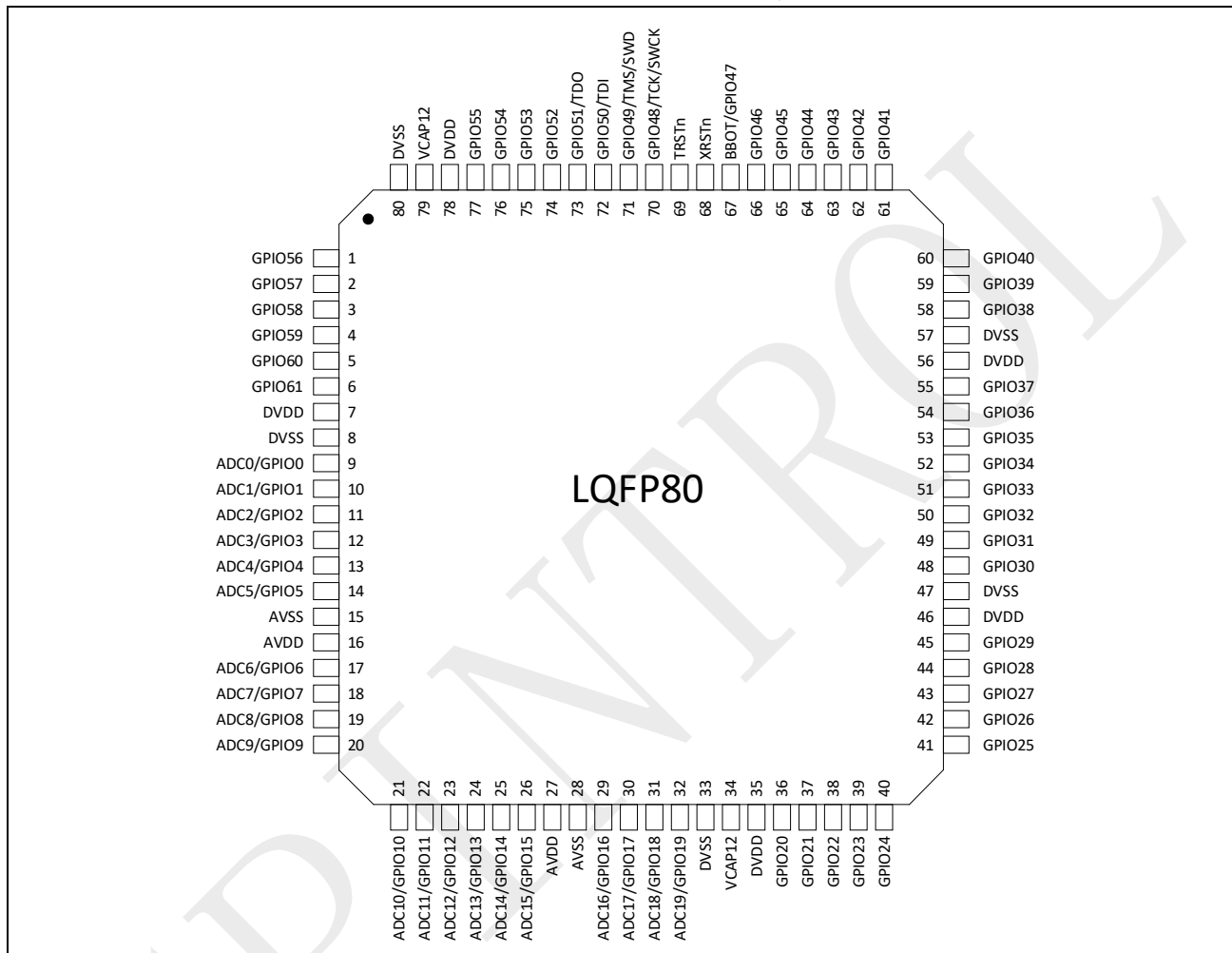
图 3-1: SPC2168 LQFP80 引脚排列
