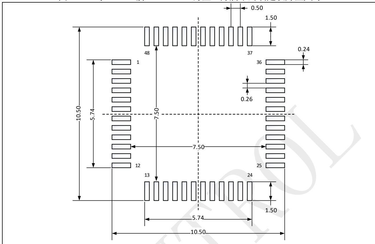
图 6-8: LQFP48-48 脚, 7 x 7 mm 薄型正方扁平封装建议焊垫尺寸
