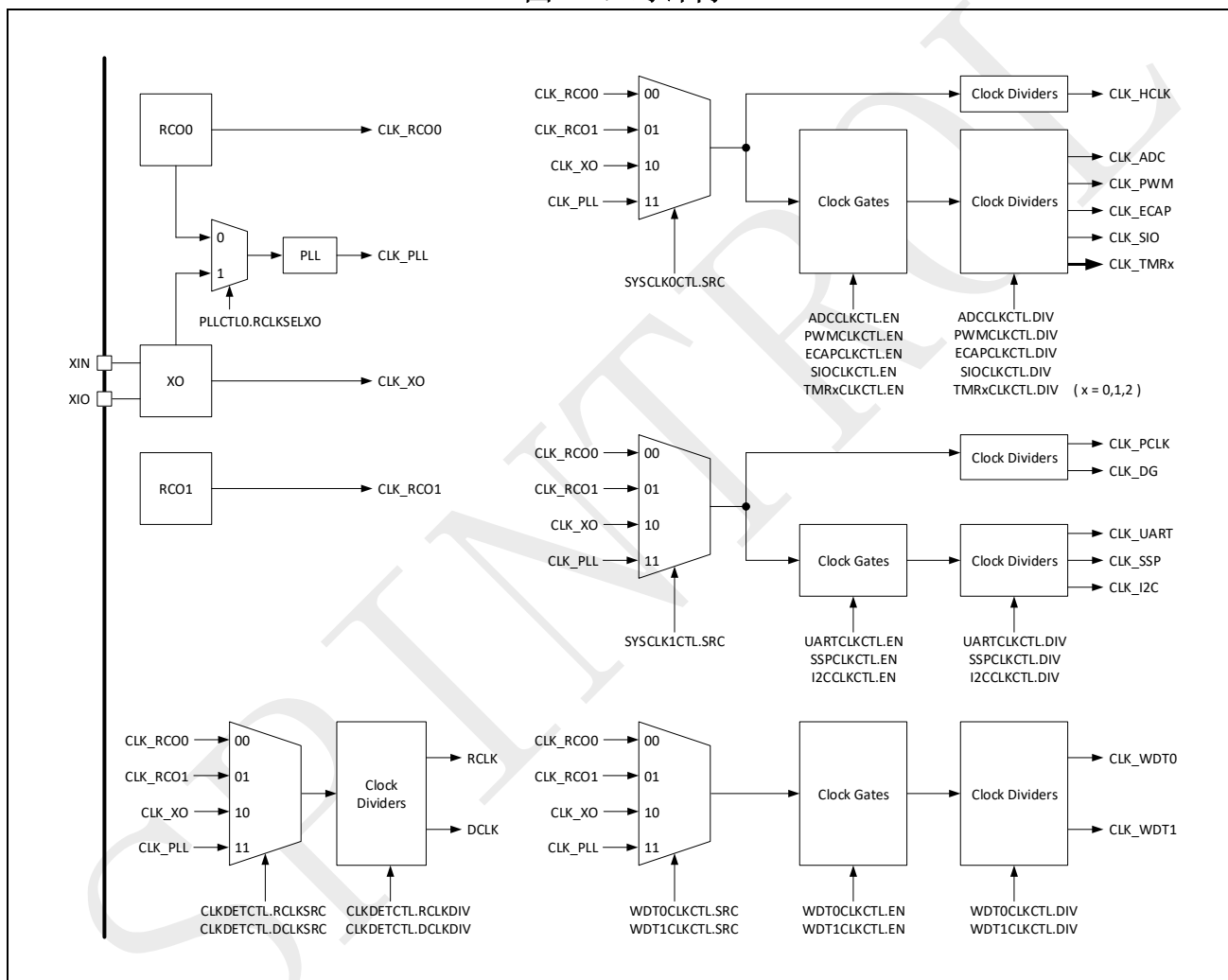
图 1-2: 时钟树
