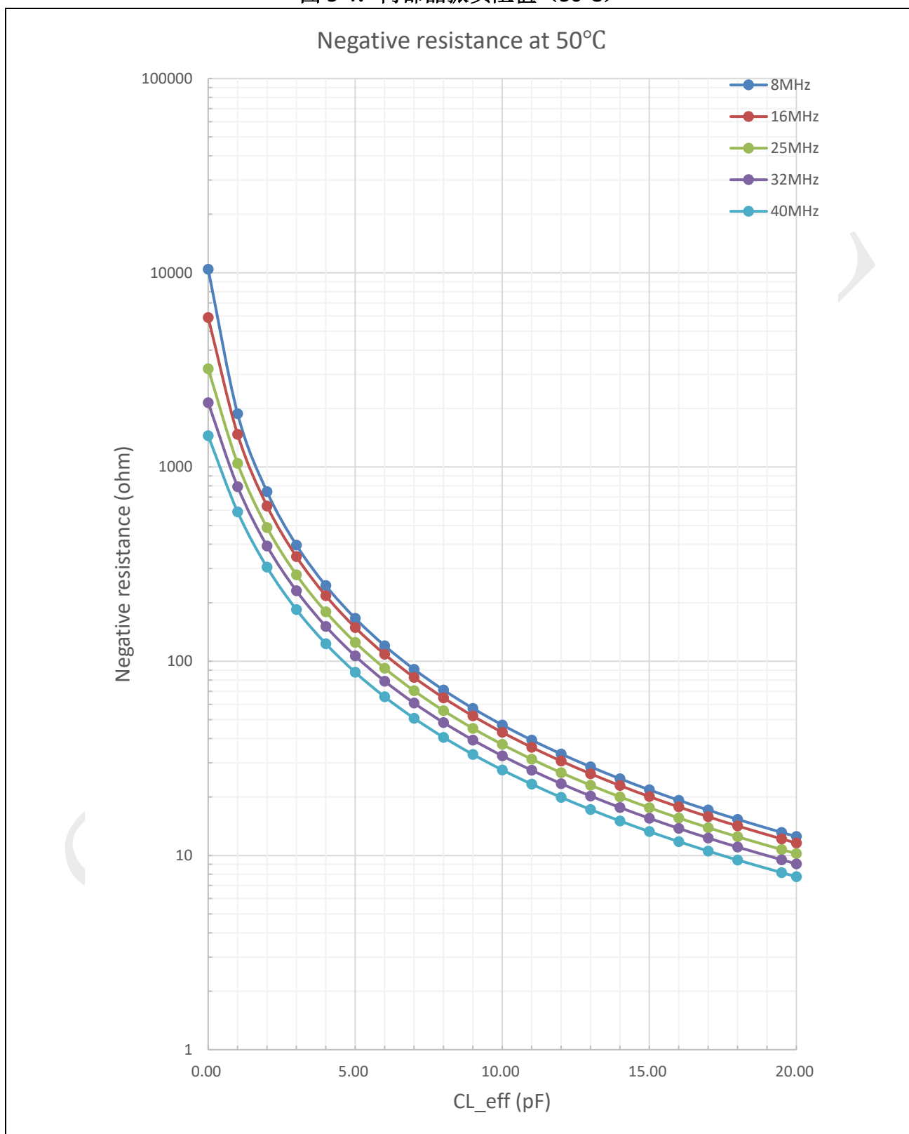
图 5-4: 内部晶振负阻值 (50°C)
