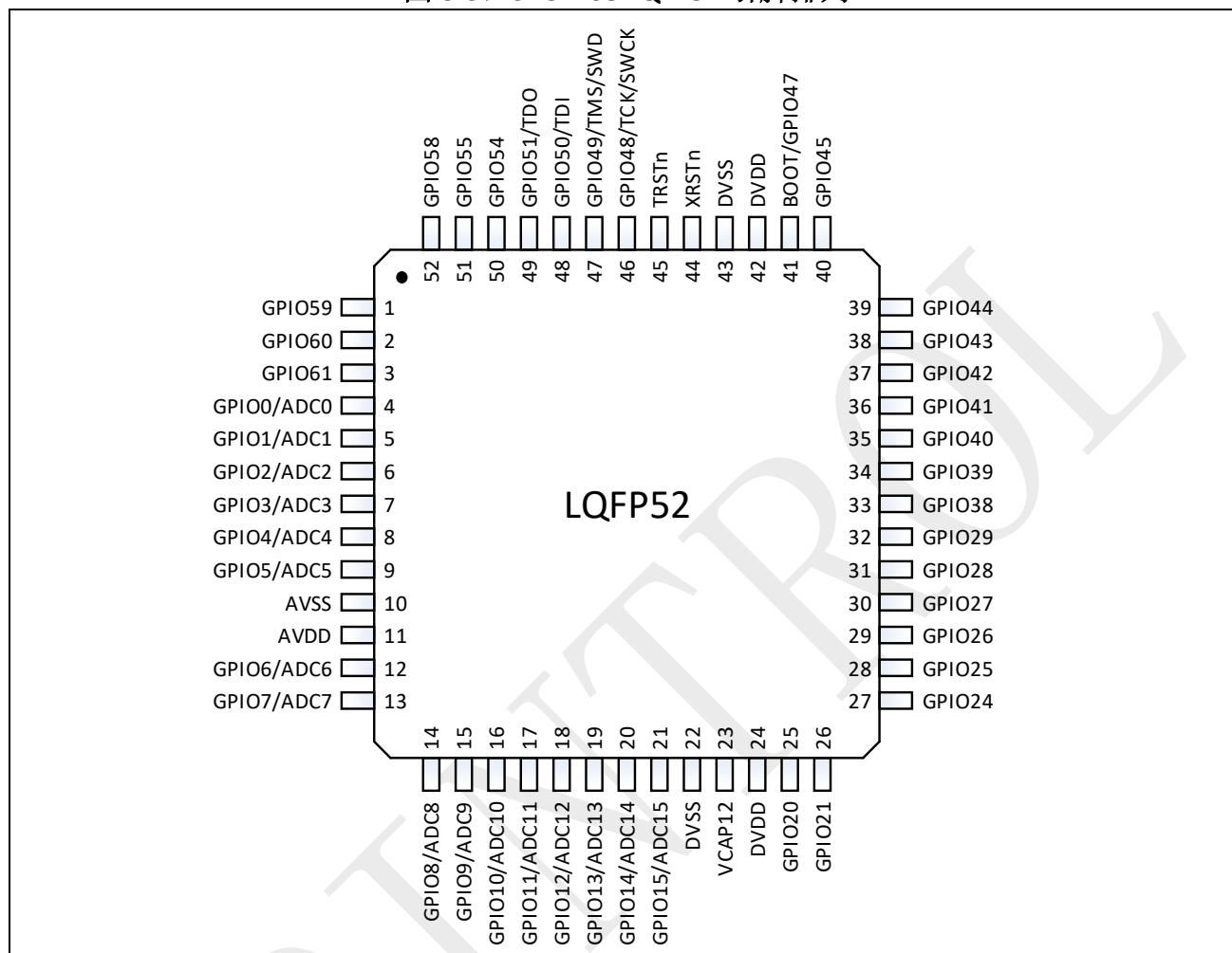
图 3-3：SPC2168 LQFP52 引脚排列
