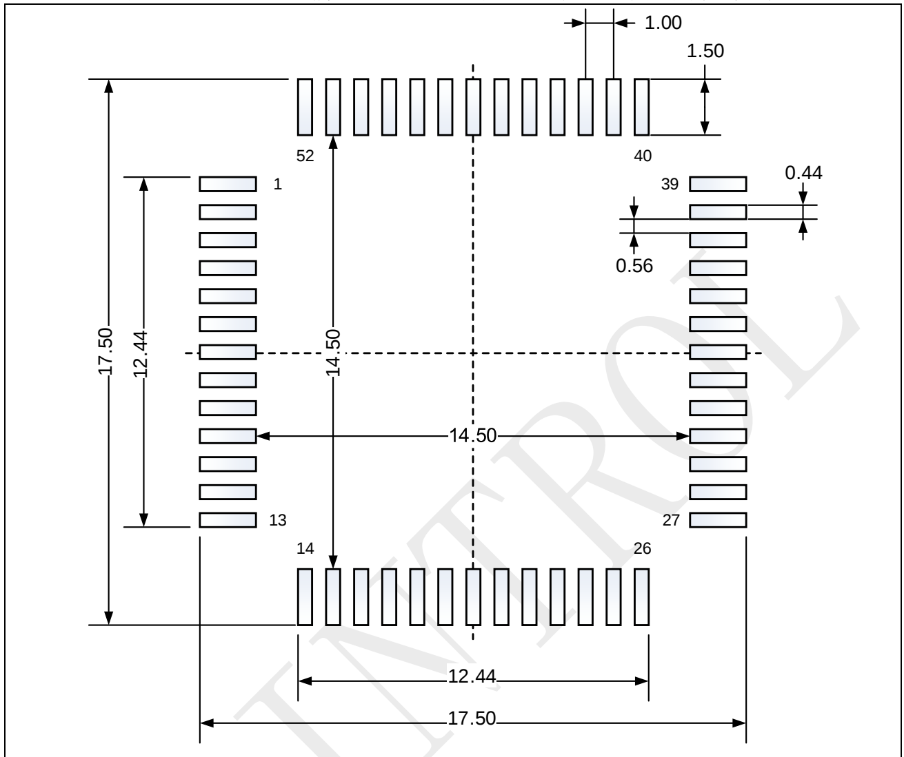
图 6-6: LQFP52-52 脚, 14 x 14 mm 薄型正方扁平封装建议焊垫尺寸
