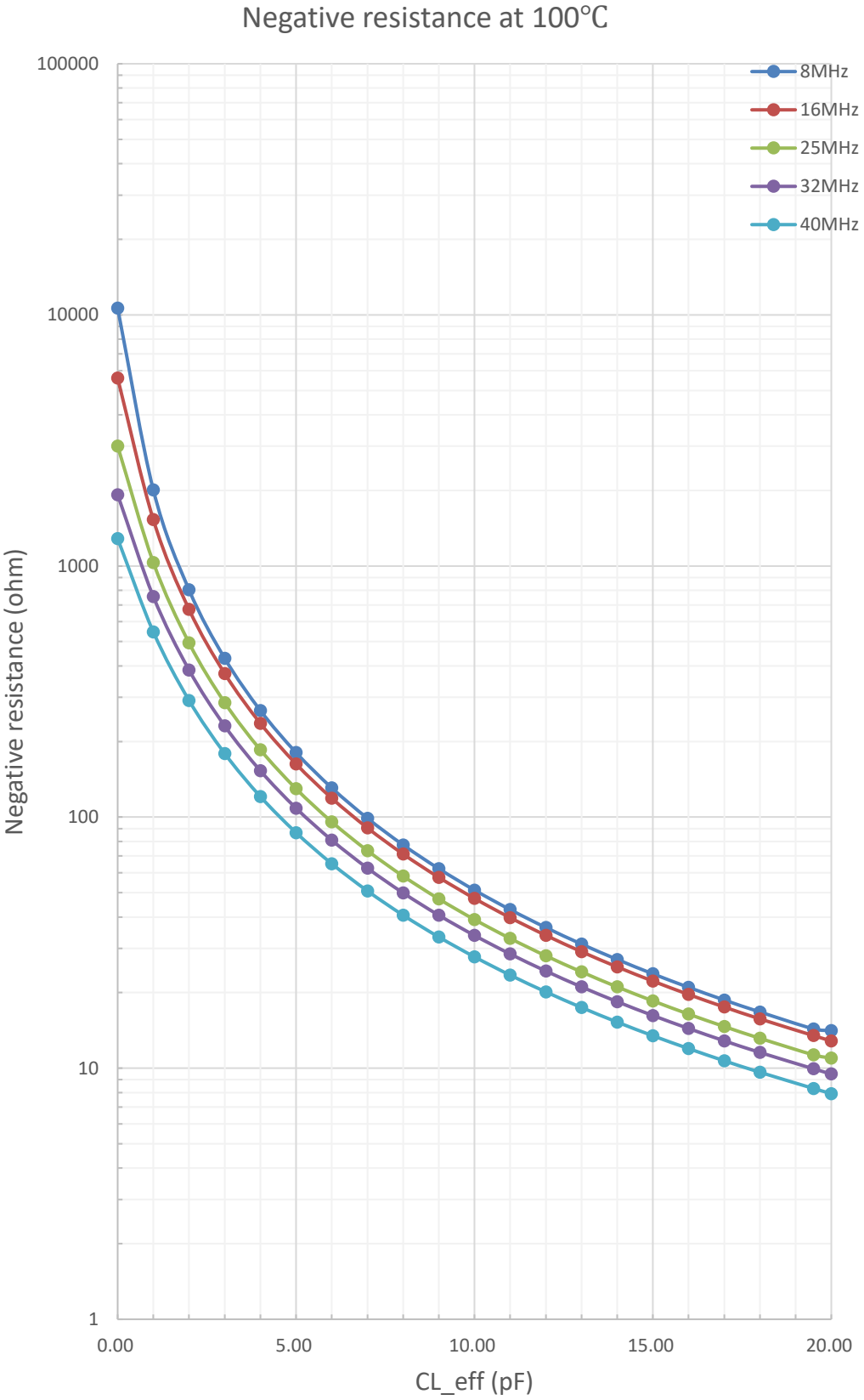
图 5-6：内部晶振负阻值（100℃）
