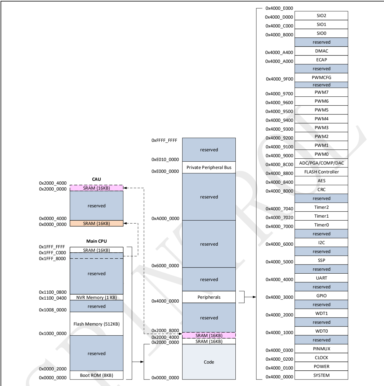
图 4-4： SPC2168 在 Cache 使能且 CAU 运行下的存储器映射（双核模式）
