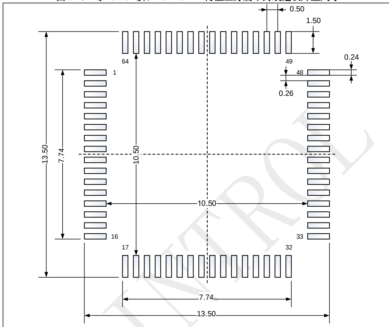
图 6-4: LQFP64—64 脚, 10 x 10 mm 薄型正方扁平封装建议焊垫尺寸
