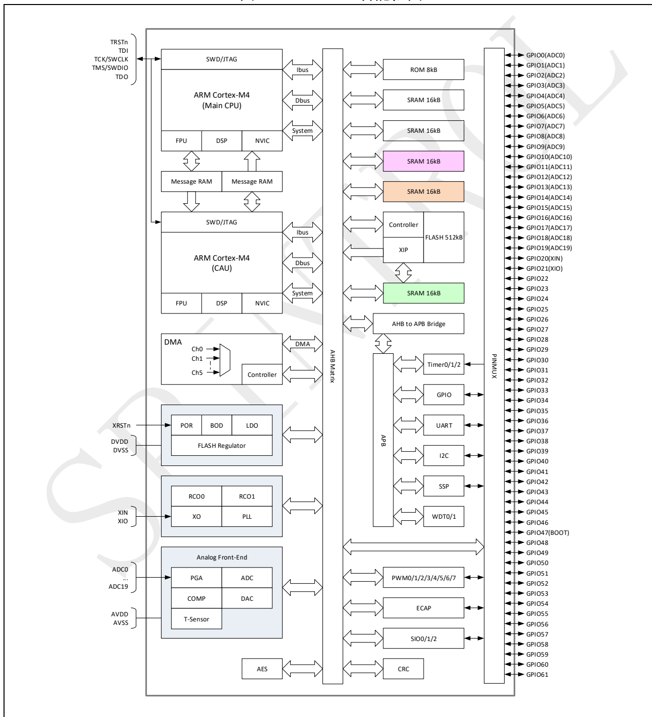
图 1-1: SPC2168 功能框图
