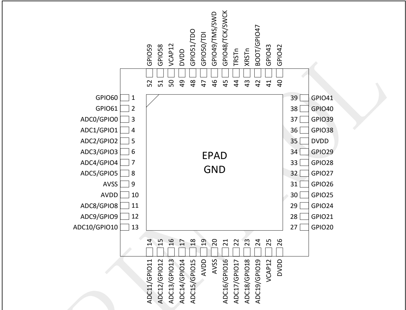
图 3-5: SPC1198 QFN52 引脚排列
