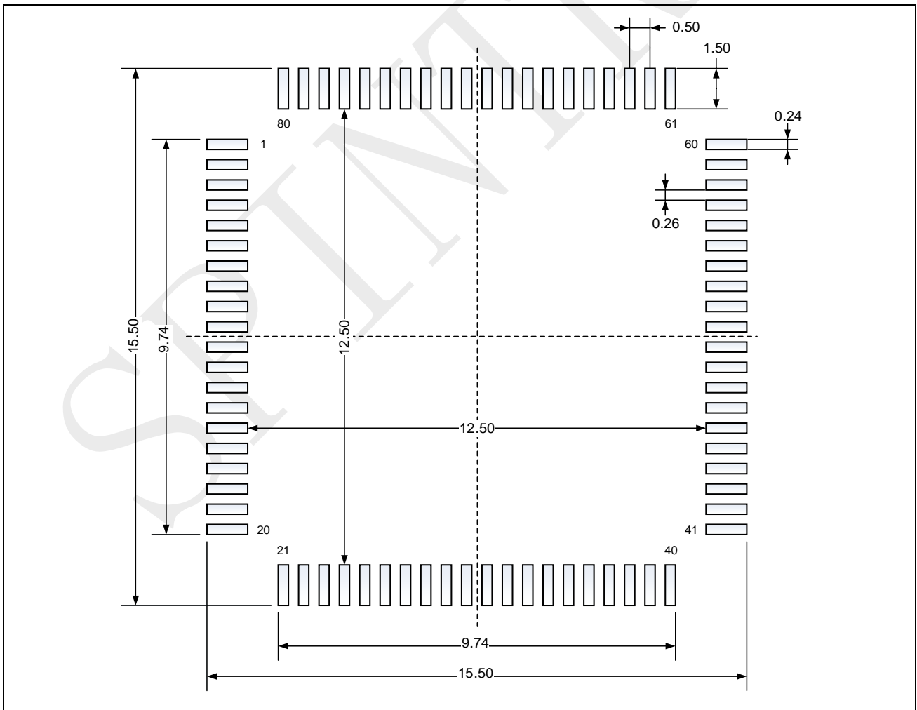
图 6-2: LQFP80 - 80 脚, 12 x 12 mm 薄型正方扁平封装建议焊垫尺寸
