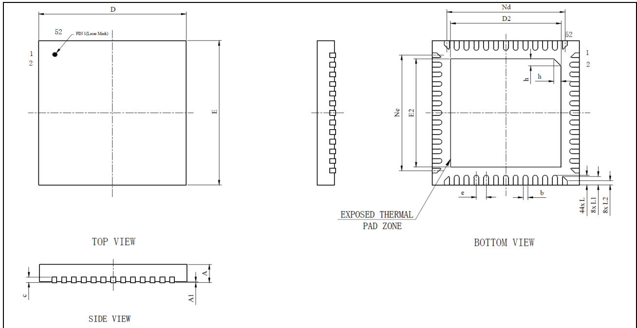
图 6-9: QFN52 - 52 脚, 6 x 6 mm 方形扁平无引脚封装图
