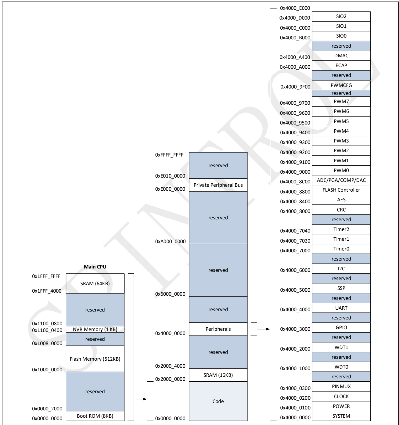
图 4-1: SPC1198 在 Cache 禁用下的存储器映射
