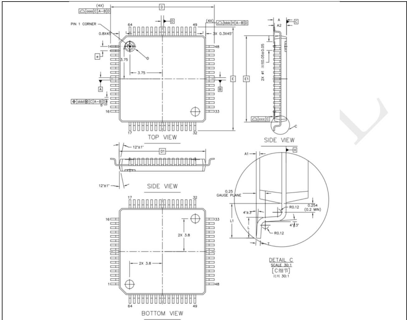
图 6-3: LQFP64 - 64 脚, 10 x 10 mm 薄型正方扁平封装图
