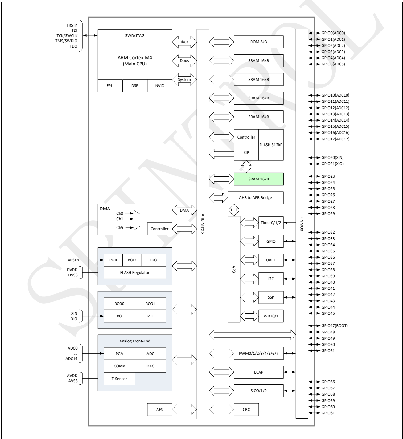
图 1-1: SPC1198 功能框图
