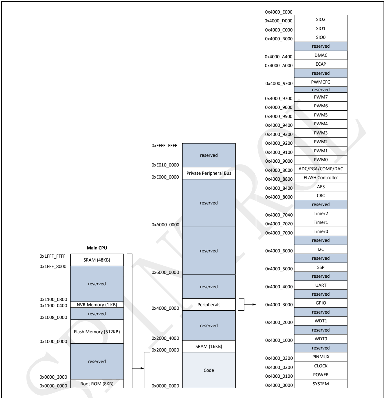
图 4-2: SPC1198 在 Cache 使能下的存储器映射
