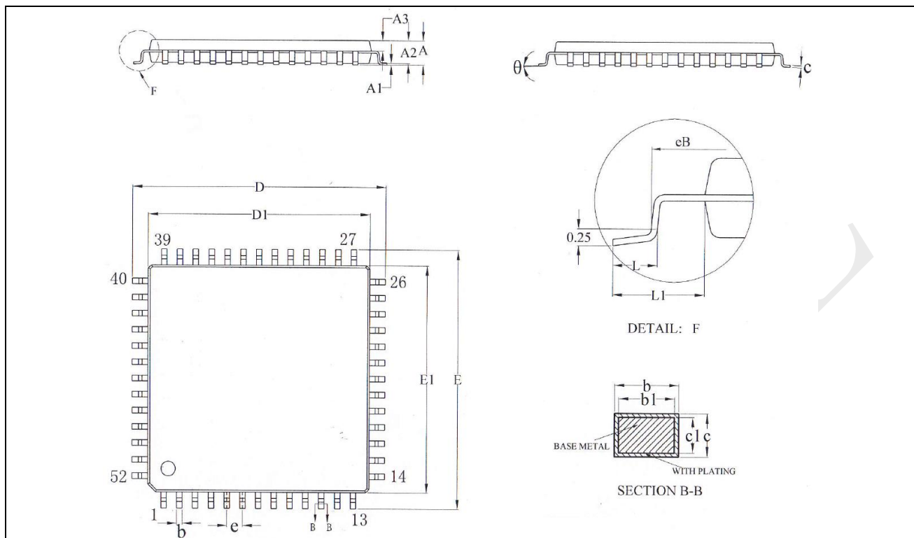
图 6-5: LQFP52 – 52 脚, 14 x 14 mm 薄型正方扁平封装图
