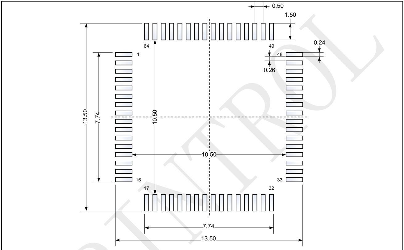
图 6-4: LQFP64 - 64 脚, 10 x 10 mm 薄型正方扁平封装建议焊垫尺寸
