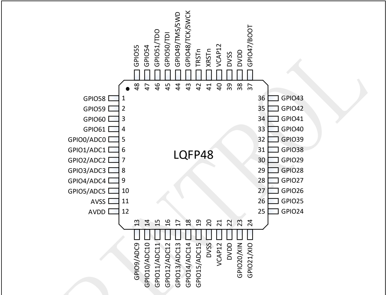
图 3-4: SPC1198 LQFP48 引脚排列
