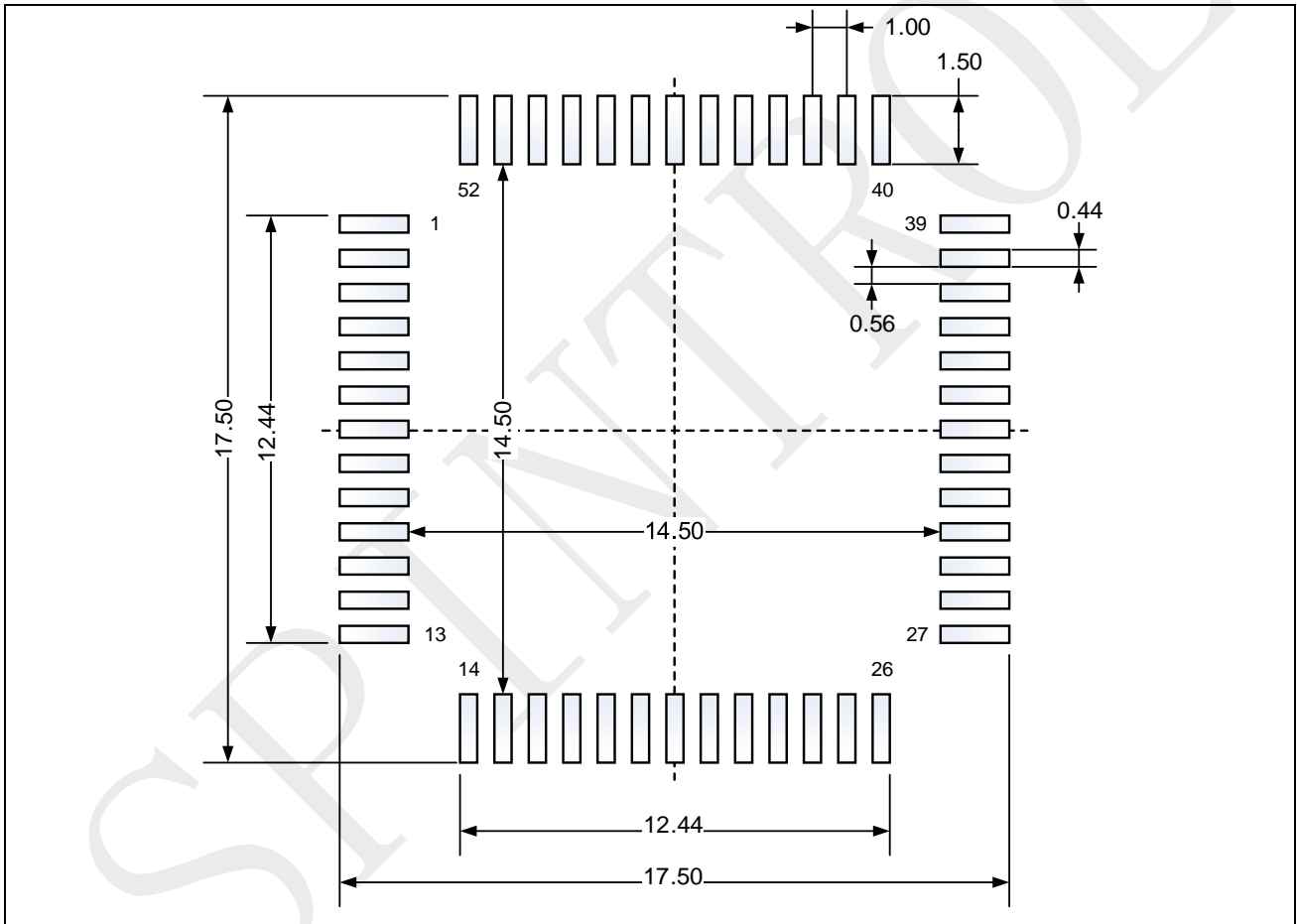
图 6-6: LQFP52 - 52 脚, 14 x 14 mm 薄型正方扁平封装建议焊垫尺寸
