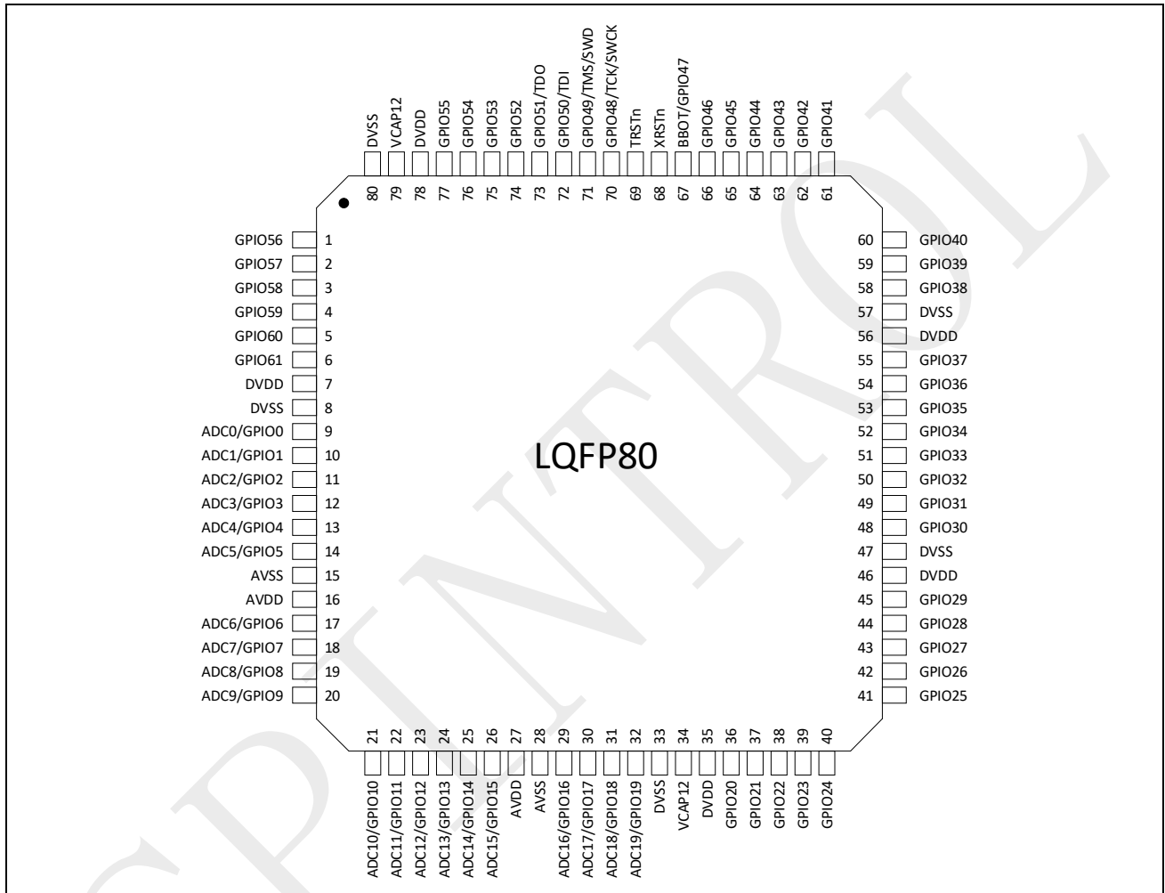
图 3-1: SPC1198 LQFP80 引脚排列
