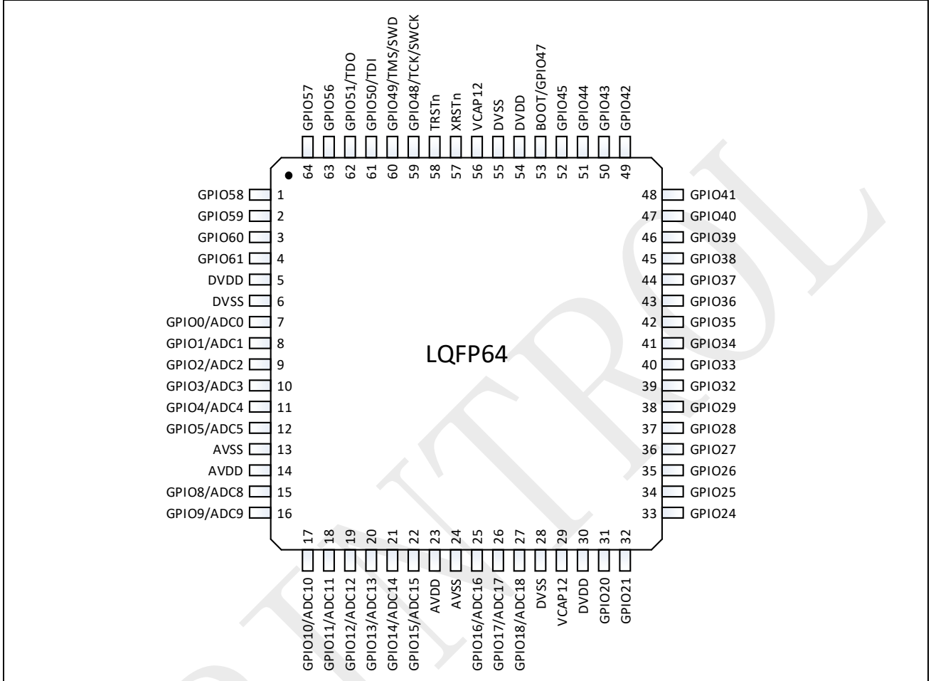
图 3-2: SPC1198 LQFP64 引脚排列
