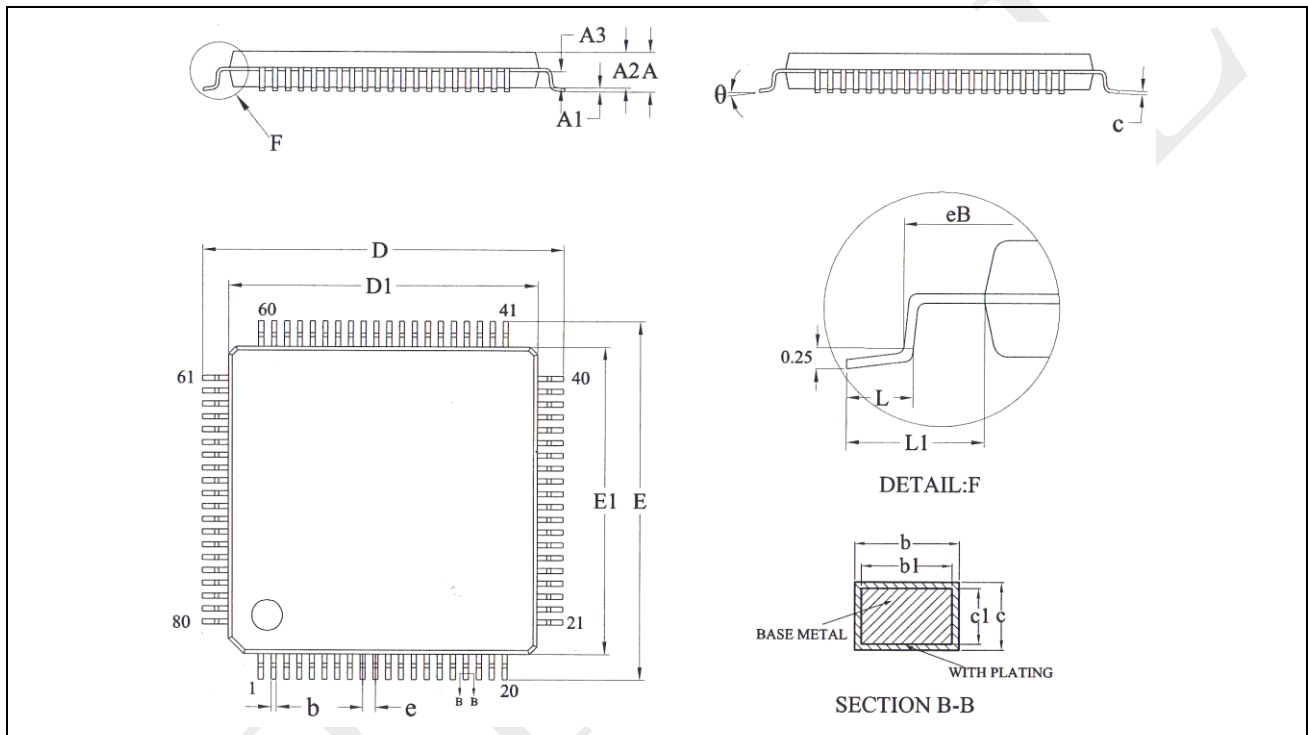
图 6-1: LQFP80 - 80 脚, 12 x 12 mm 薄型正方扁平封装图
