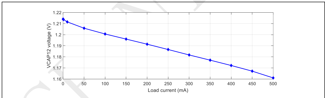
图 5-2: 内部 1.2V 稳压器负载调节率 ( T_A = 25^\circ C )
