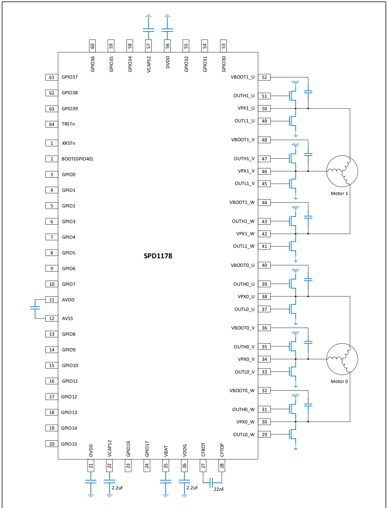
图 24-1: SPD1178 典型应用图
