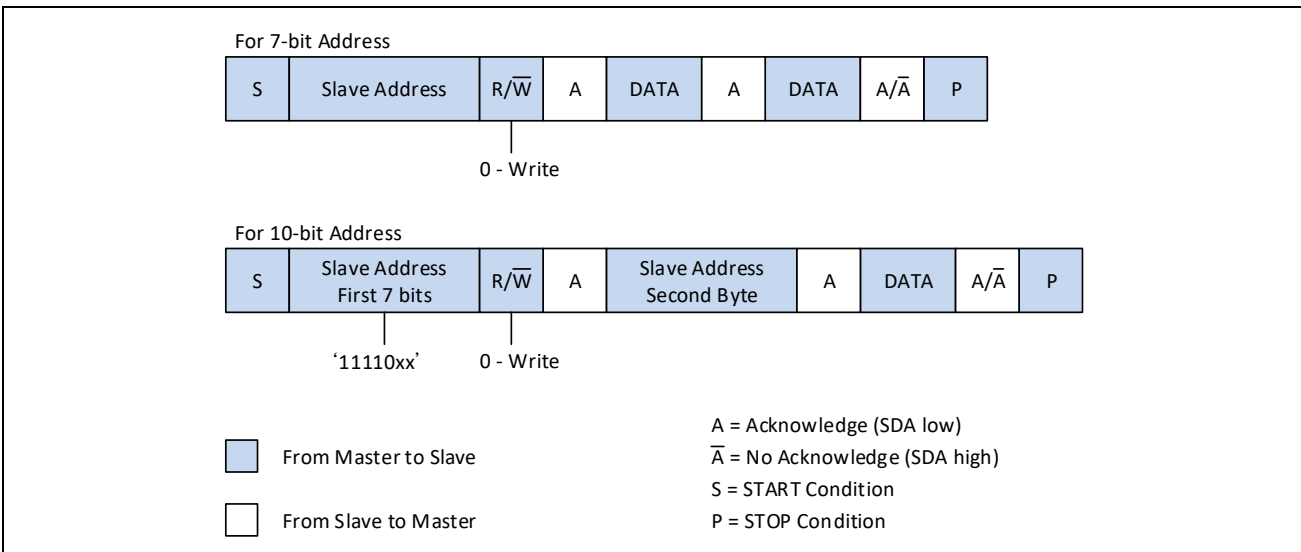
图 18-5：主机-发送器协议
