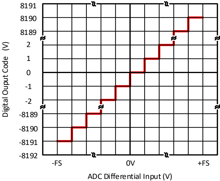
图 12-15: ADC 转换曲线
