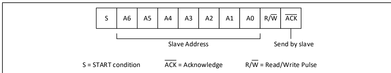
图 18-3: 7 位地址格式
