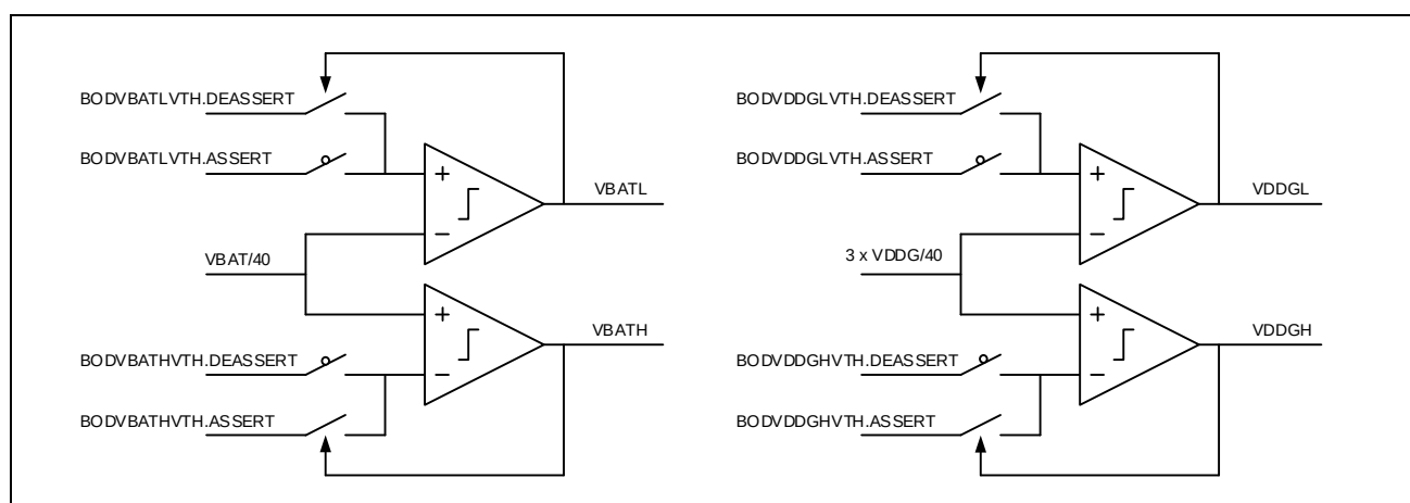
图 24-8: VBAT 和 VDDG 电源检测器
