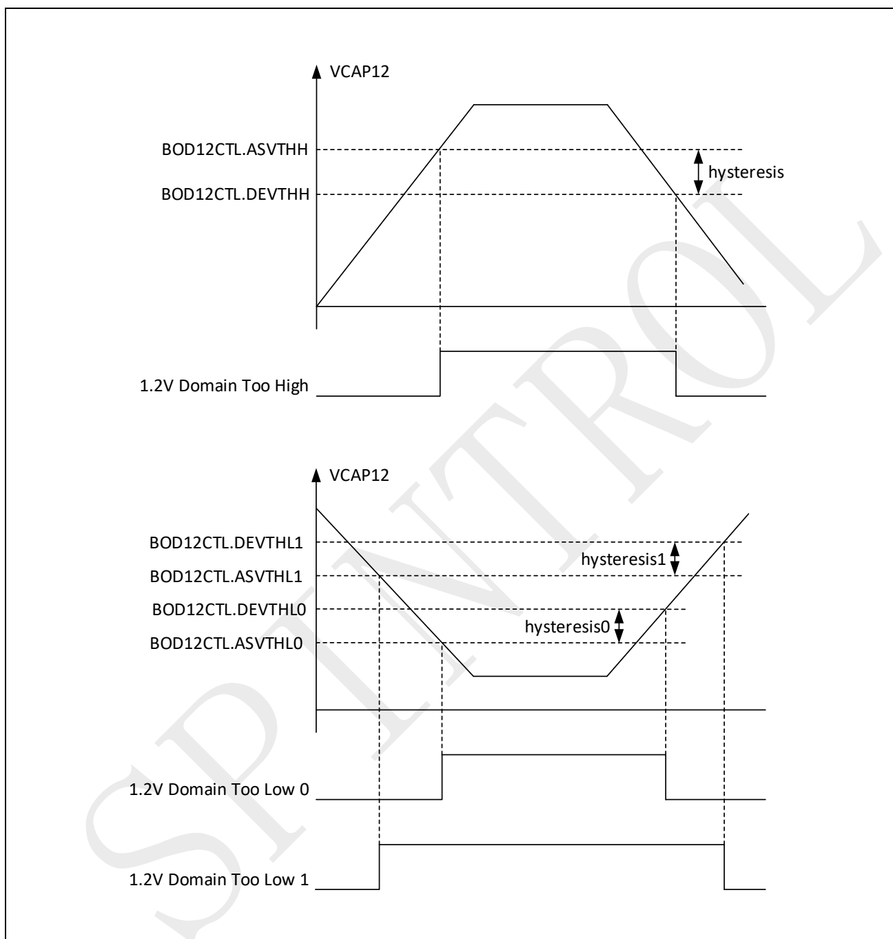
图 2-6: VCAP12 阈值
