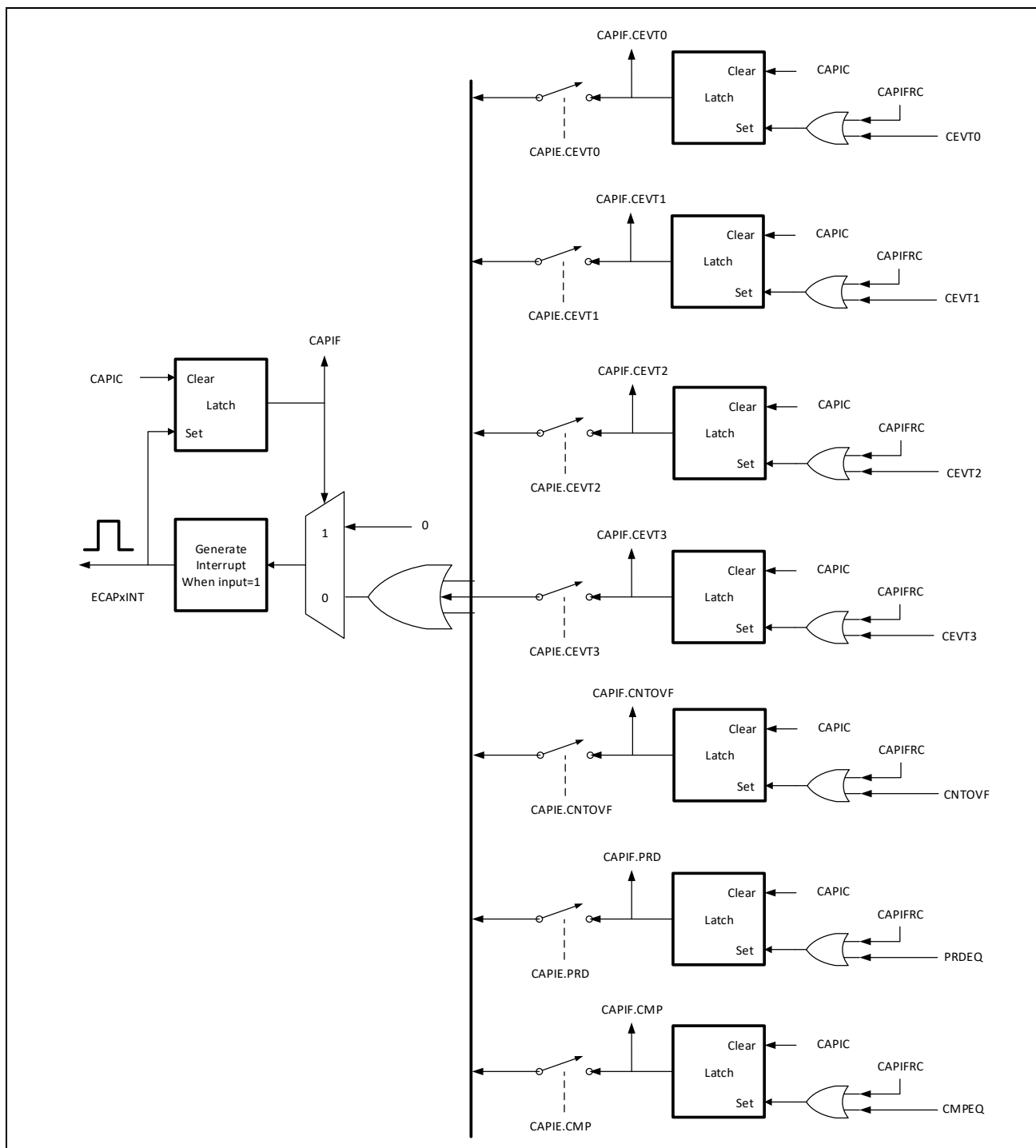
图 11-8: ECAP 模块的中断
