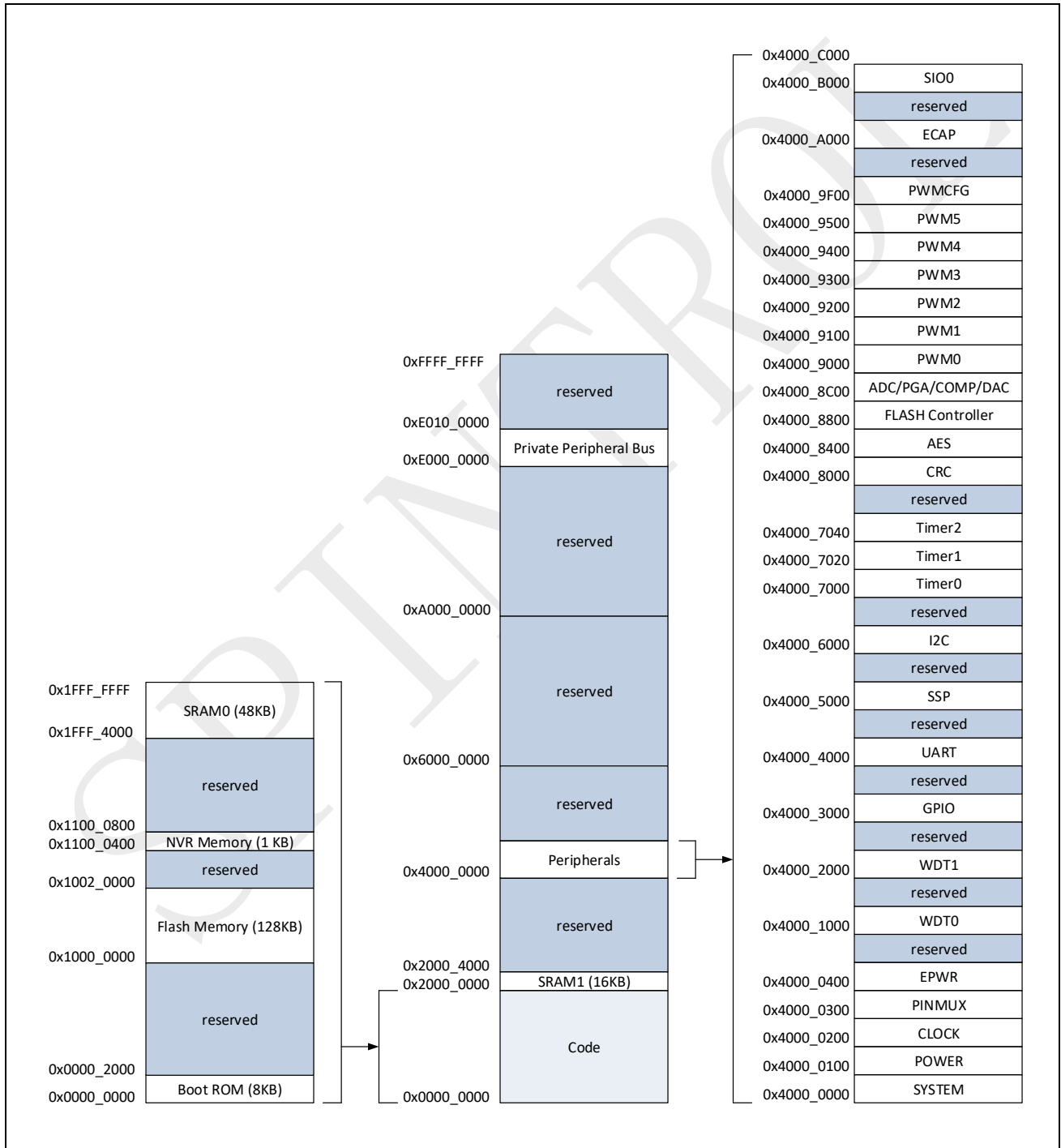
图 1-3: SPD1178 存储空间地址映射
