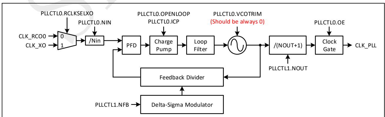
图 3-6: PLL 结构总览
