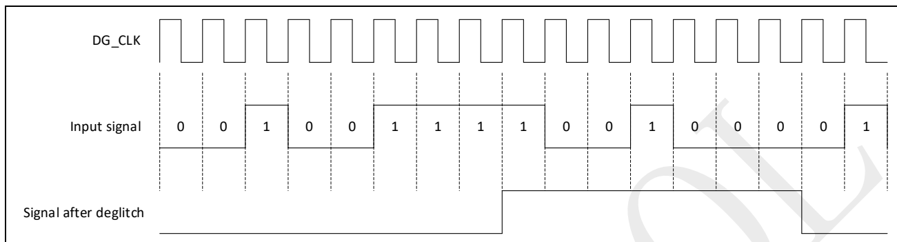
图 4-4：输入消抖
