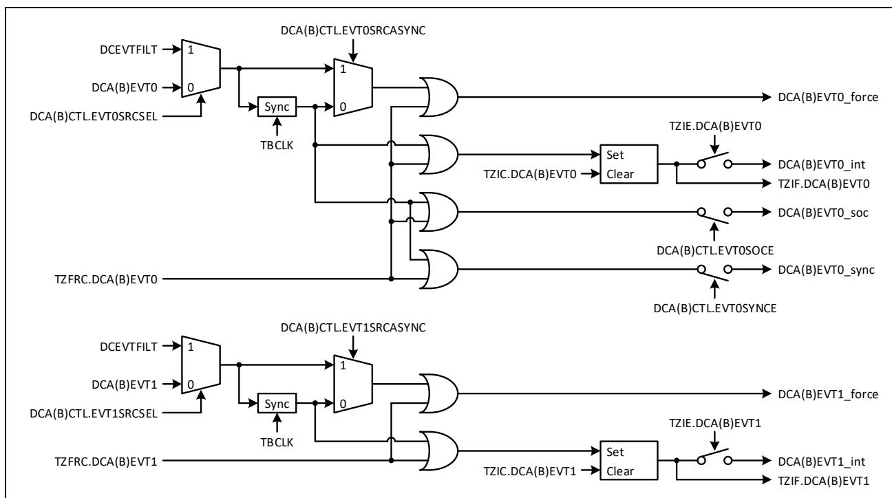
图 10-19: 事件处理
