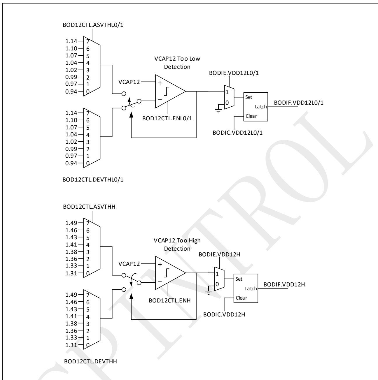
图 2-4: 1.2V 额定电压域检测电路框图
