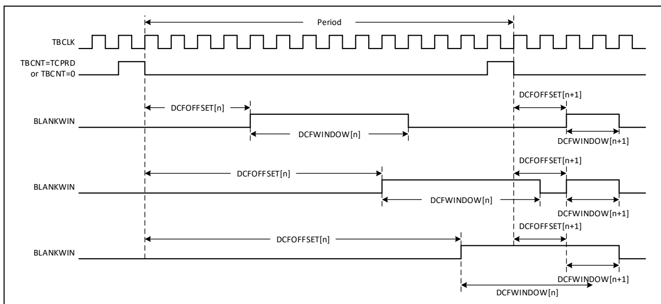
图 10-18: 消隐窗口时序图
