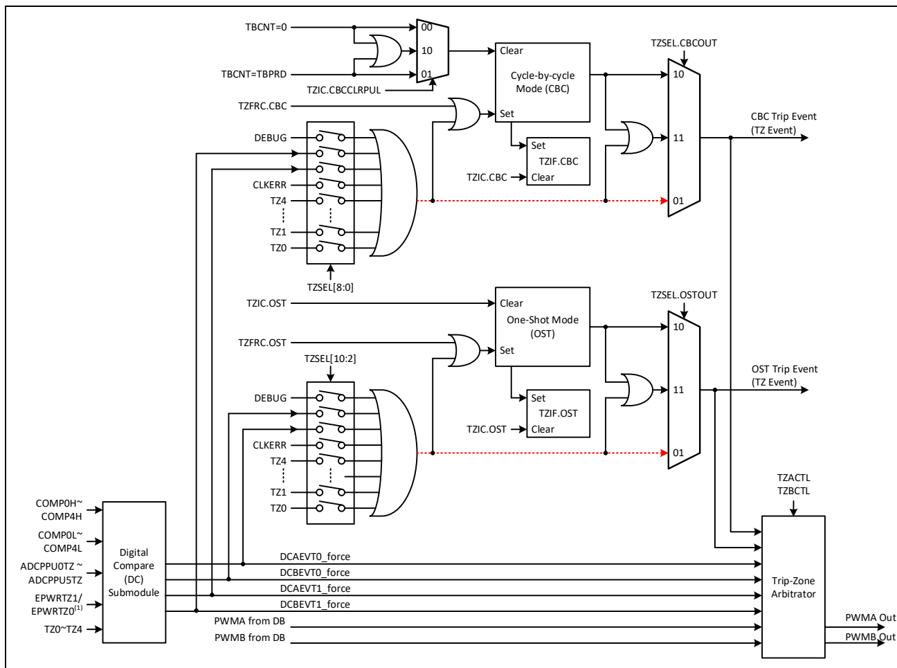
图 10-14：信号封锁子模块结构
