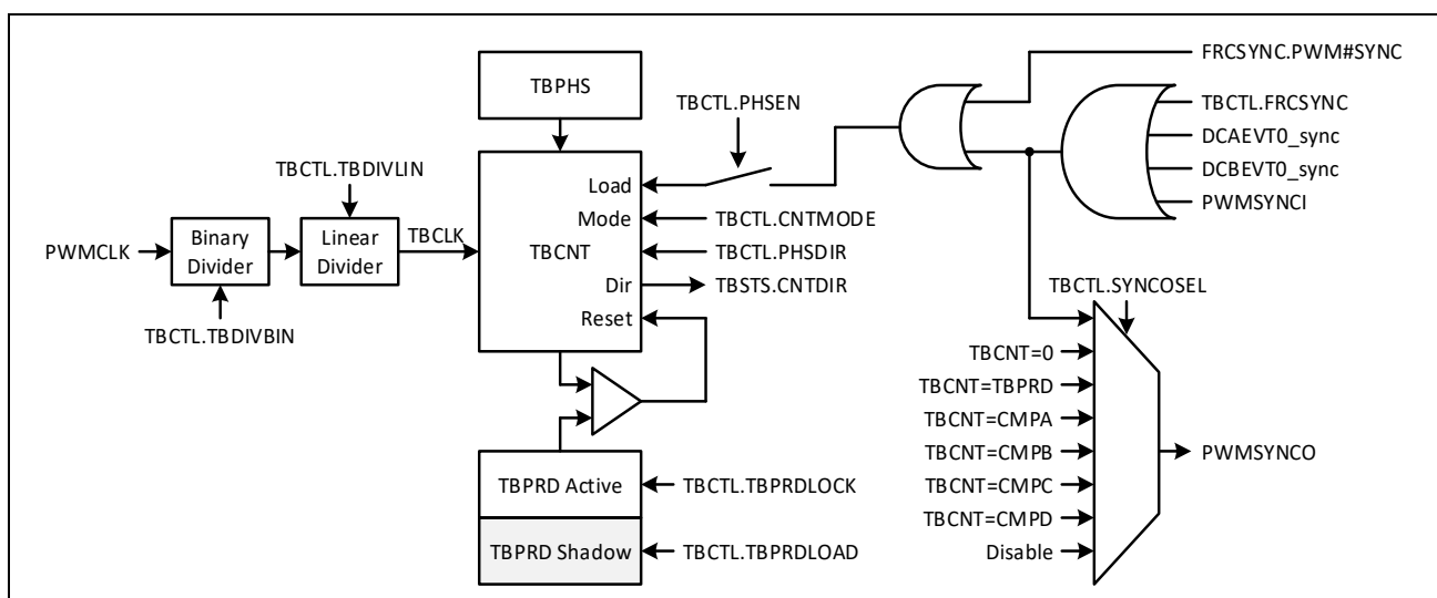
图 10-3: PWM 时基产生子模块信号链
