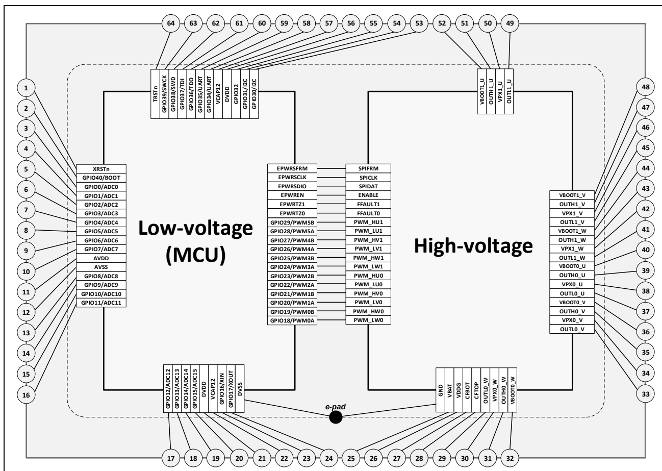
图 24-2: MCU 和高压模块之间的物理通信原理
