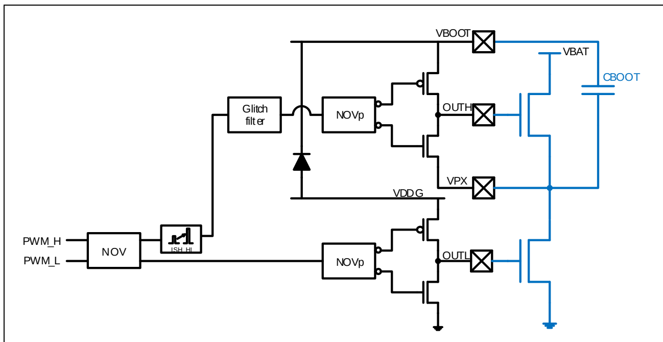
图 24-6：单相预驱简化框图
