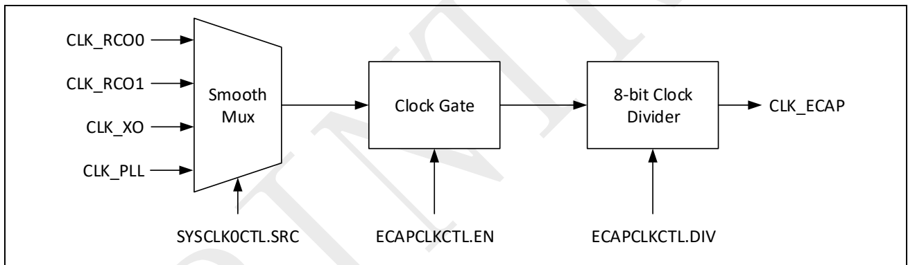
图 3-16: ECAP 时钟控制框图
