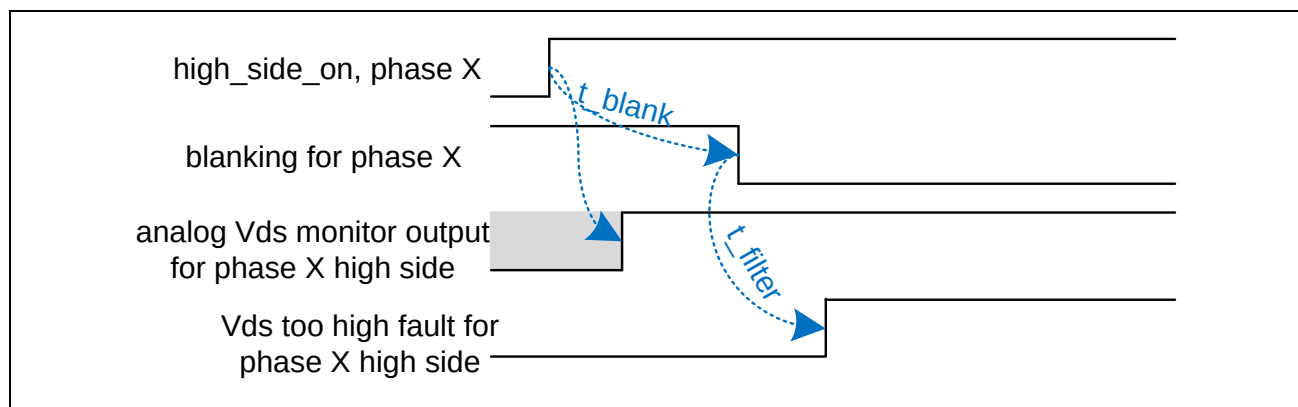
图 24-10：故障信号的消隐和滤波效果
