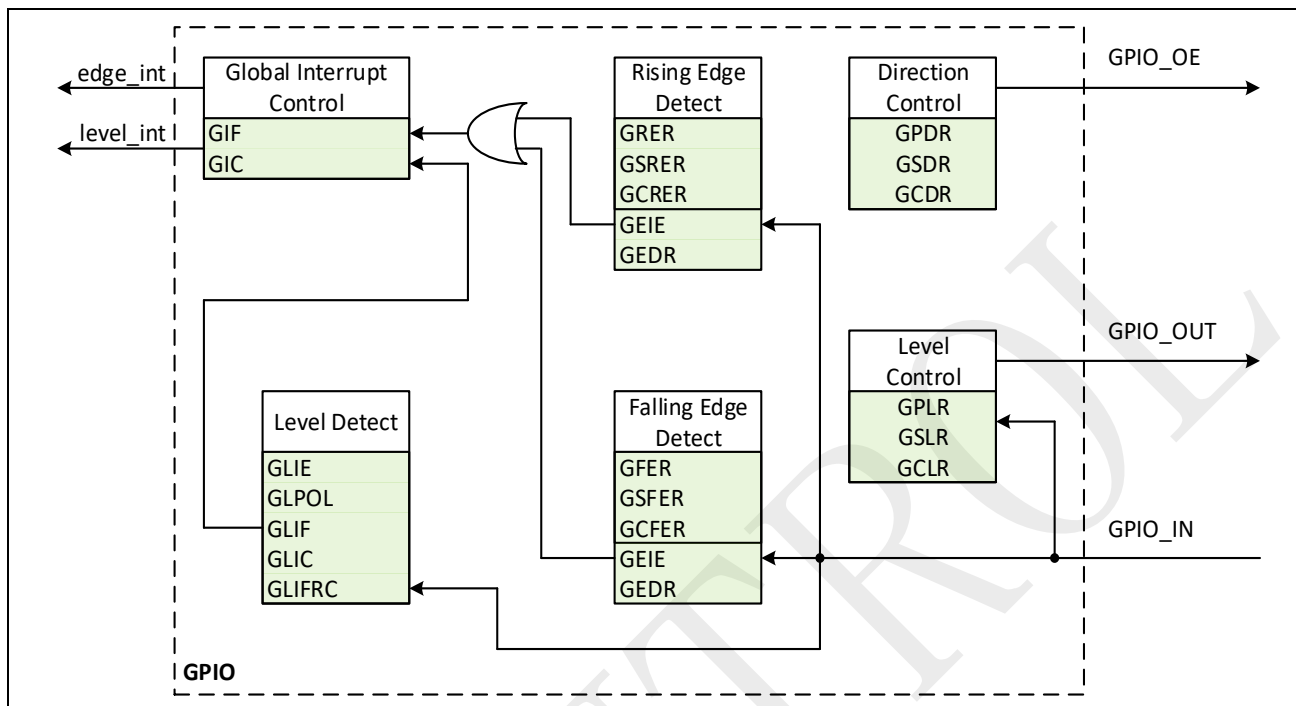
图 4-5: GPIO 结构框图
