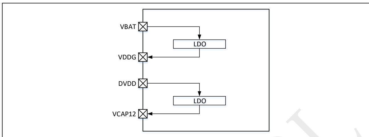
图 2-2：电源产生单元
