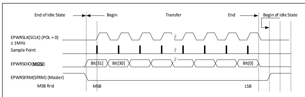
图 24-3：MCU 向高压模块发送数据
