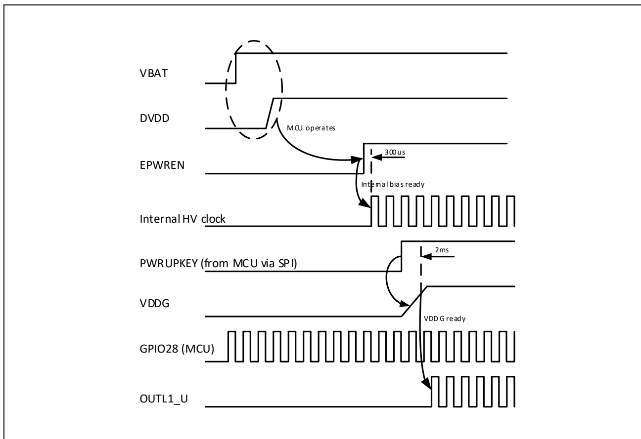
图 24-5：预驱信号上电方案
