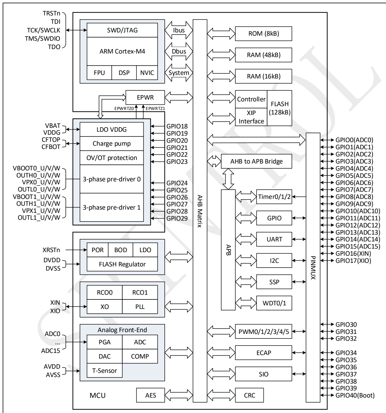
图 1-1: SPD1178 系统框图
