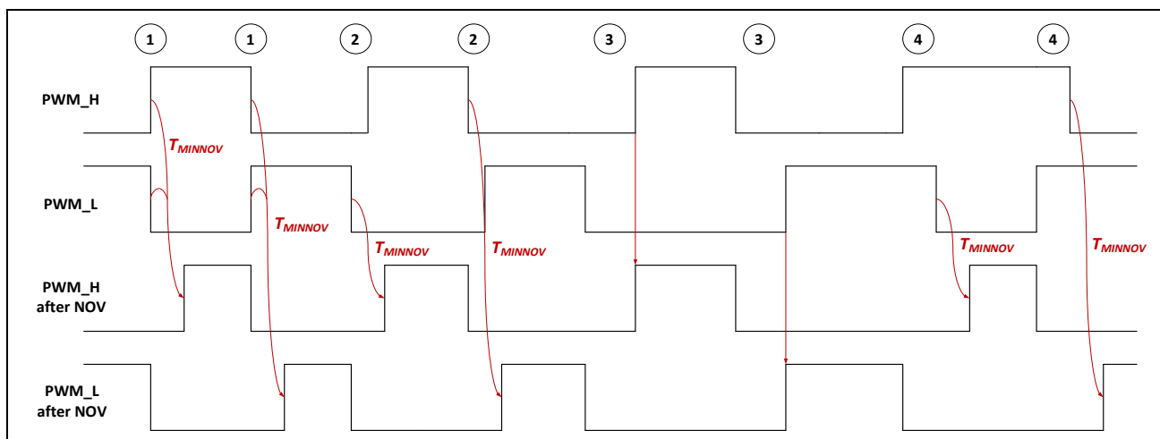
图 24-7: NOV 模块工作描述
