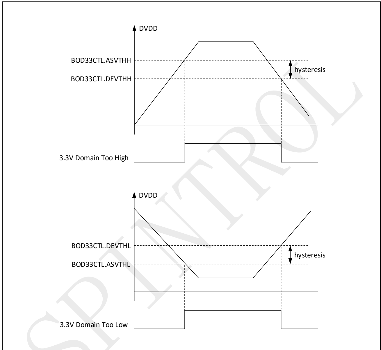
图 2-5: DVDD 阈值
