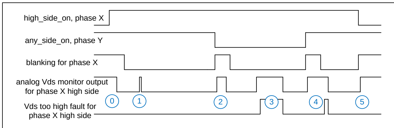
图 24-9: V_{ds} 监测器消隐框图
