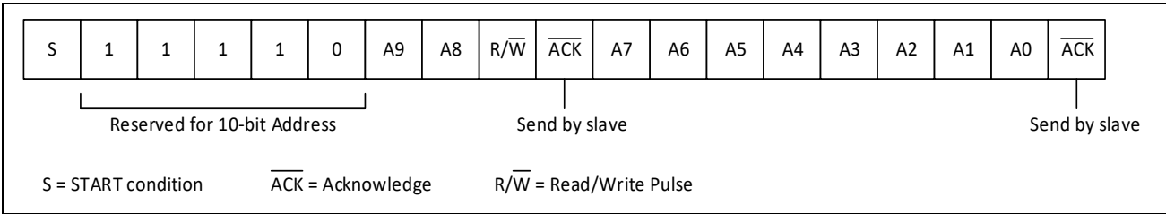
图 18-4：10 位地址格式
