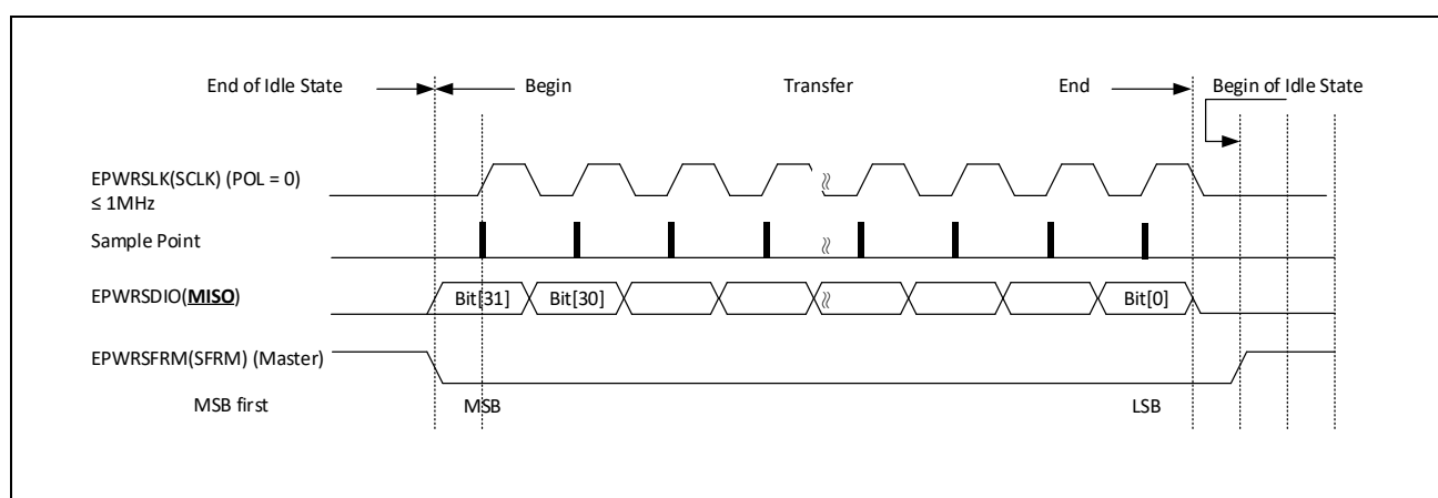
图 24-4：MCU 从高压模块接受数据
