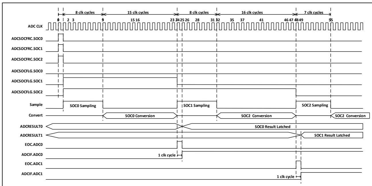
图 12-12: 顺序转换模式时序
