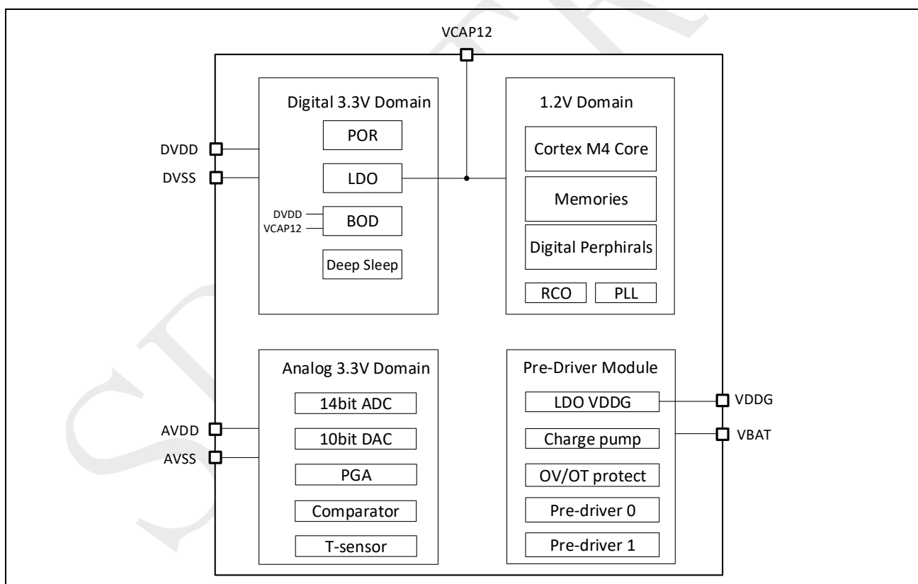
图 2-1: 电源系统总览
