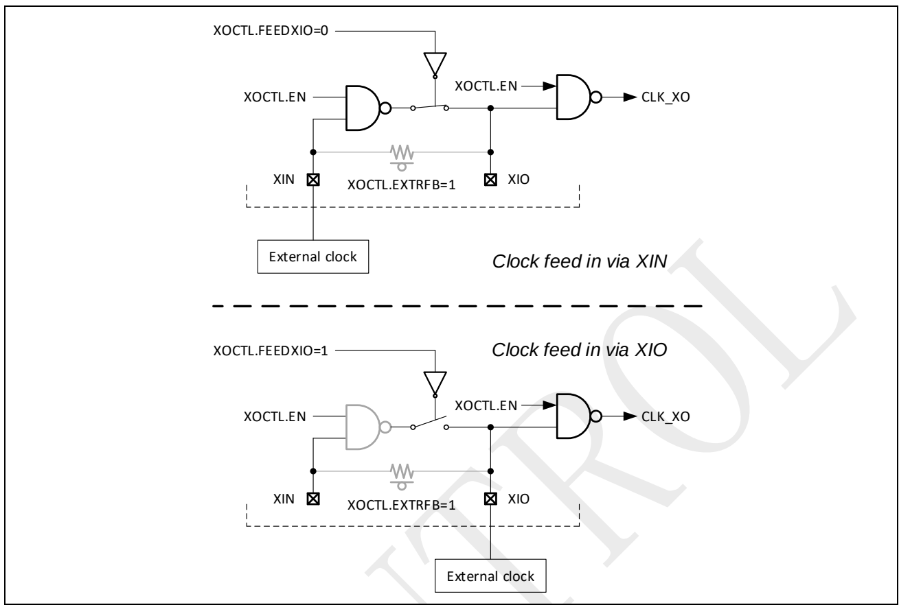
图 3-5: 外部时钟模式
