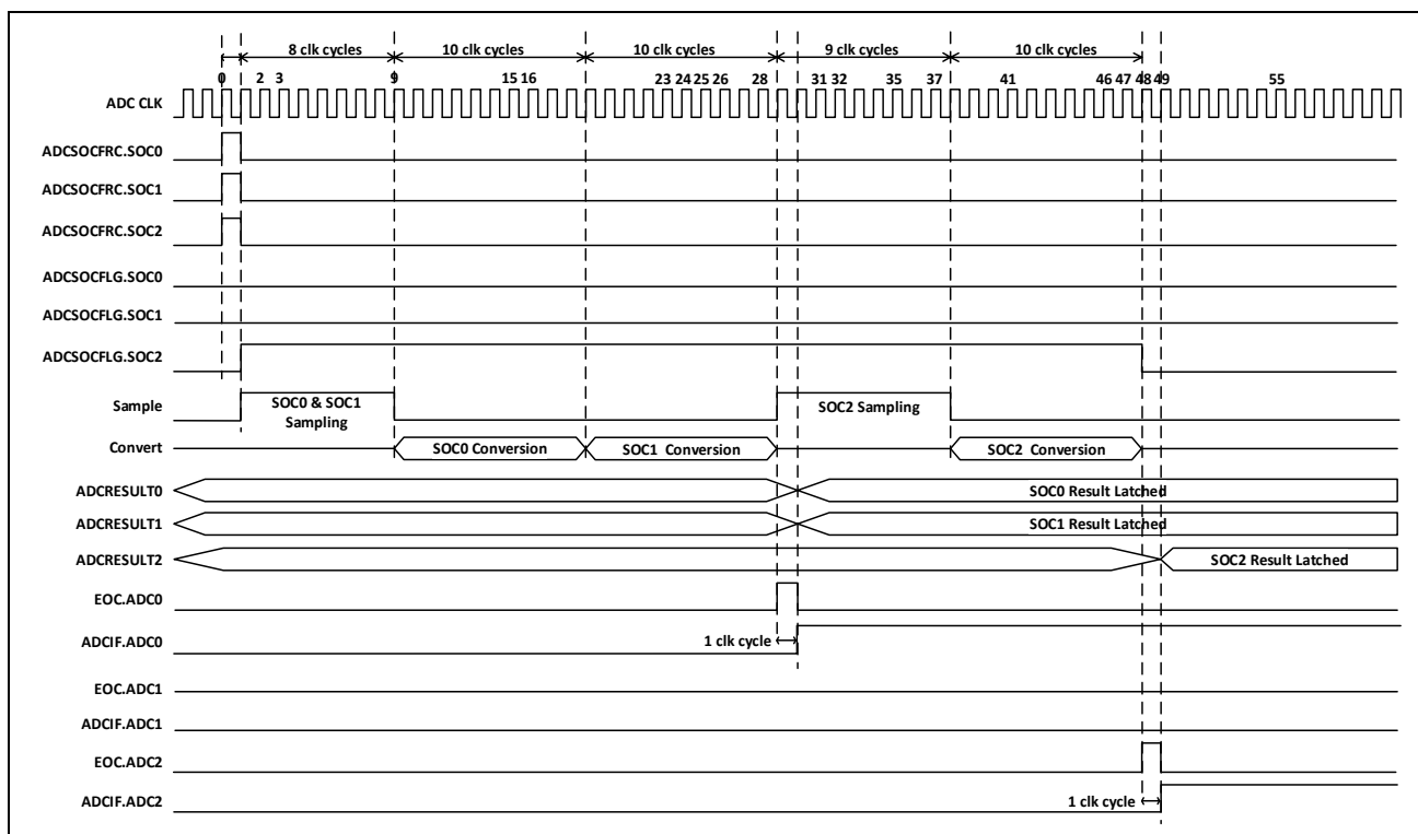
图 12-13: 同时采样模式时序
