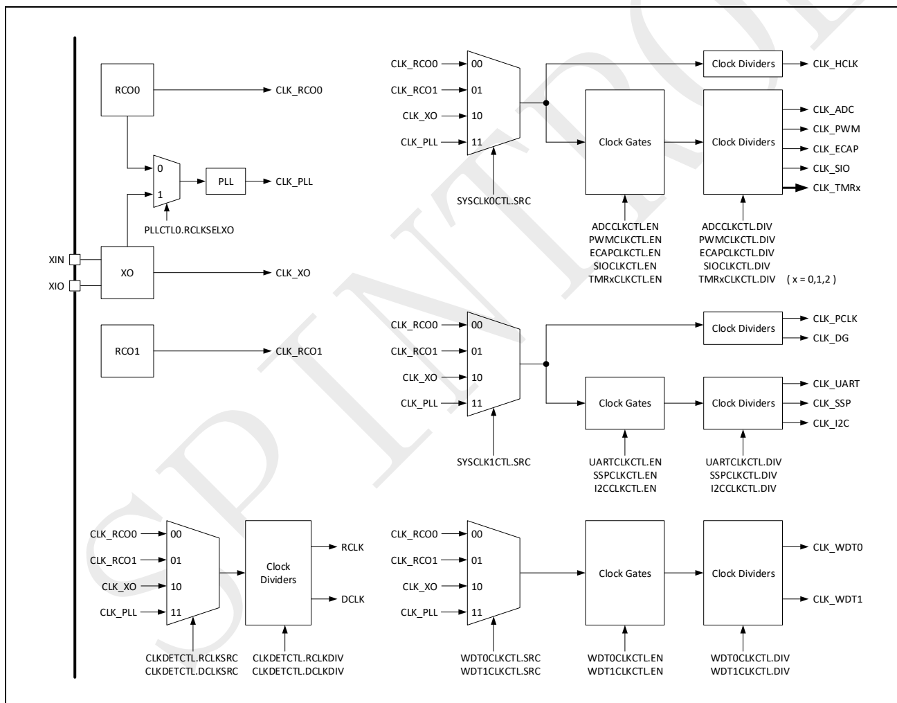
图 1-2：SPD1178 时钟树
