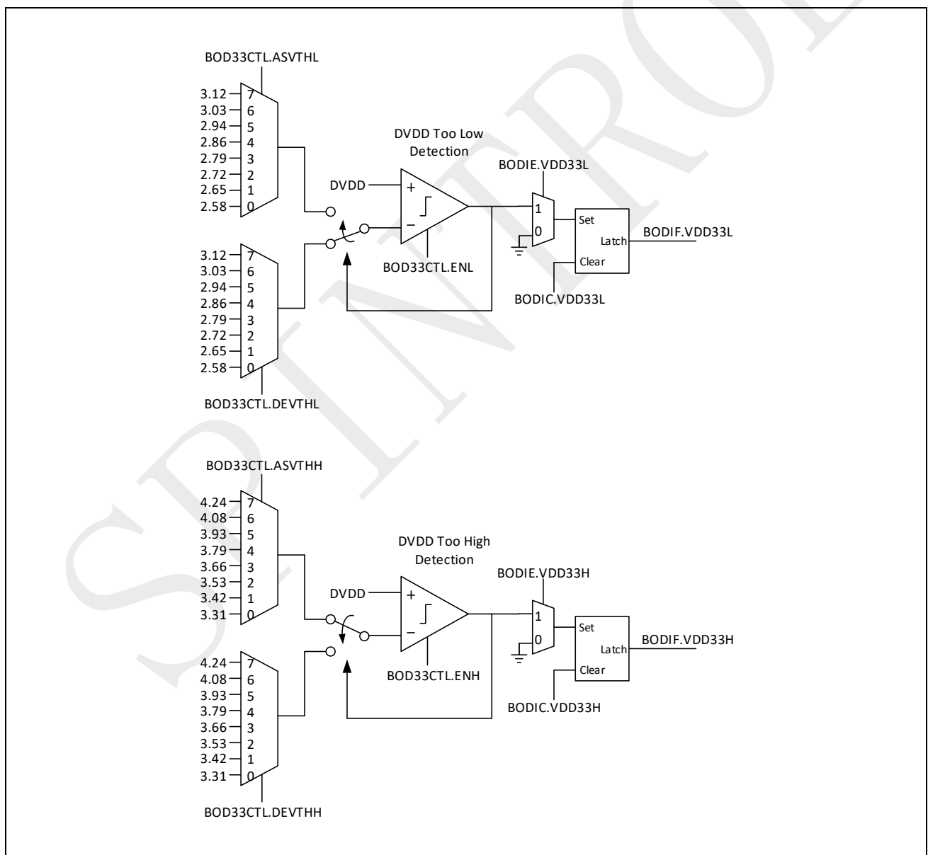
图 2-3：3.3V 额定电压域检测电路框图
